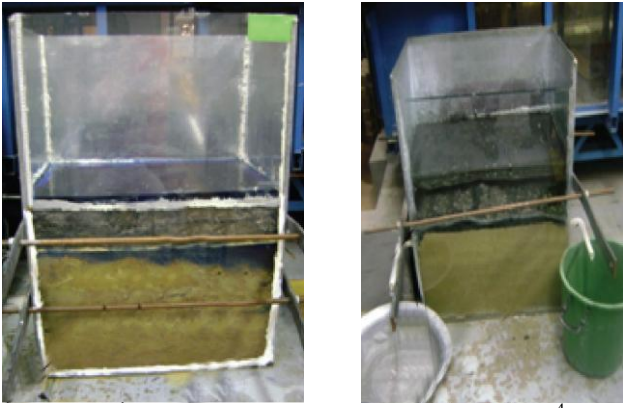
Figura N°3-4 Modelo experimental 1 y 2 4
