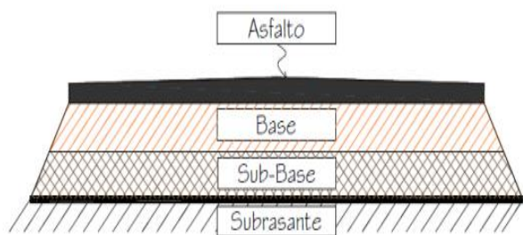
Figura N°1. Sección típica de un pavimento flexible. 2
