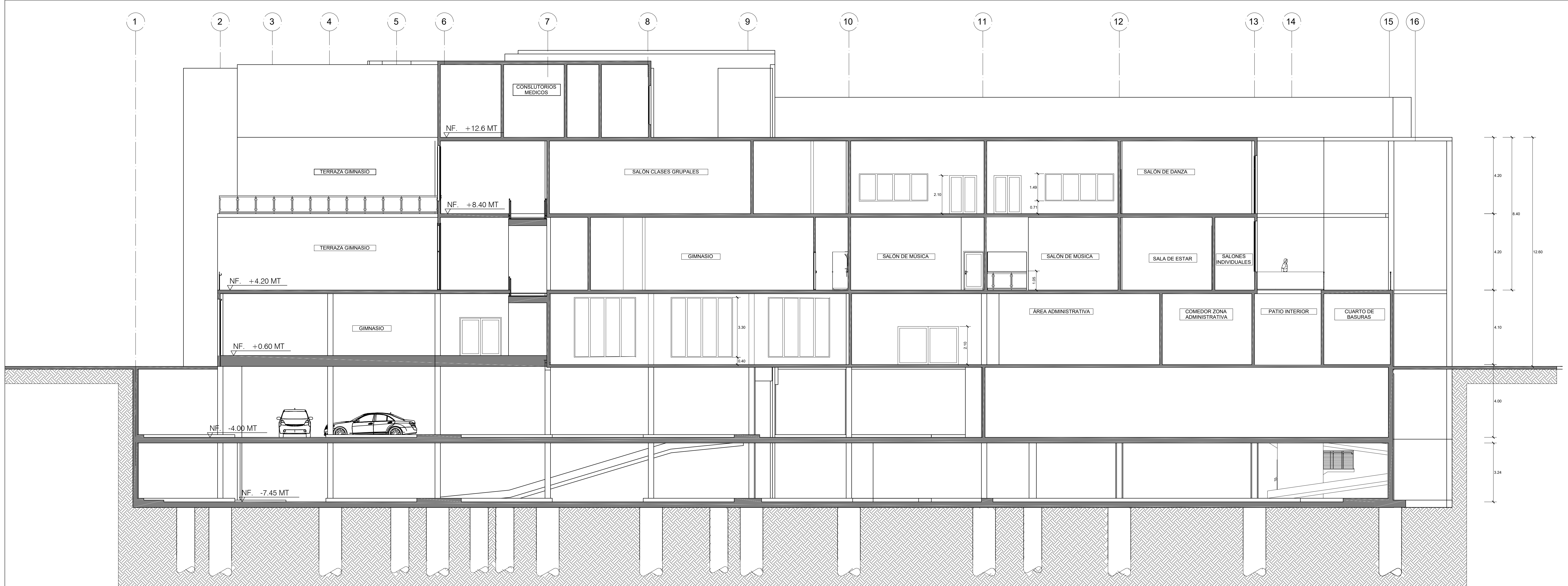
A CORTE 3 ESCALA 1:100
