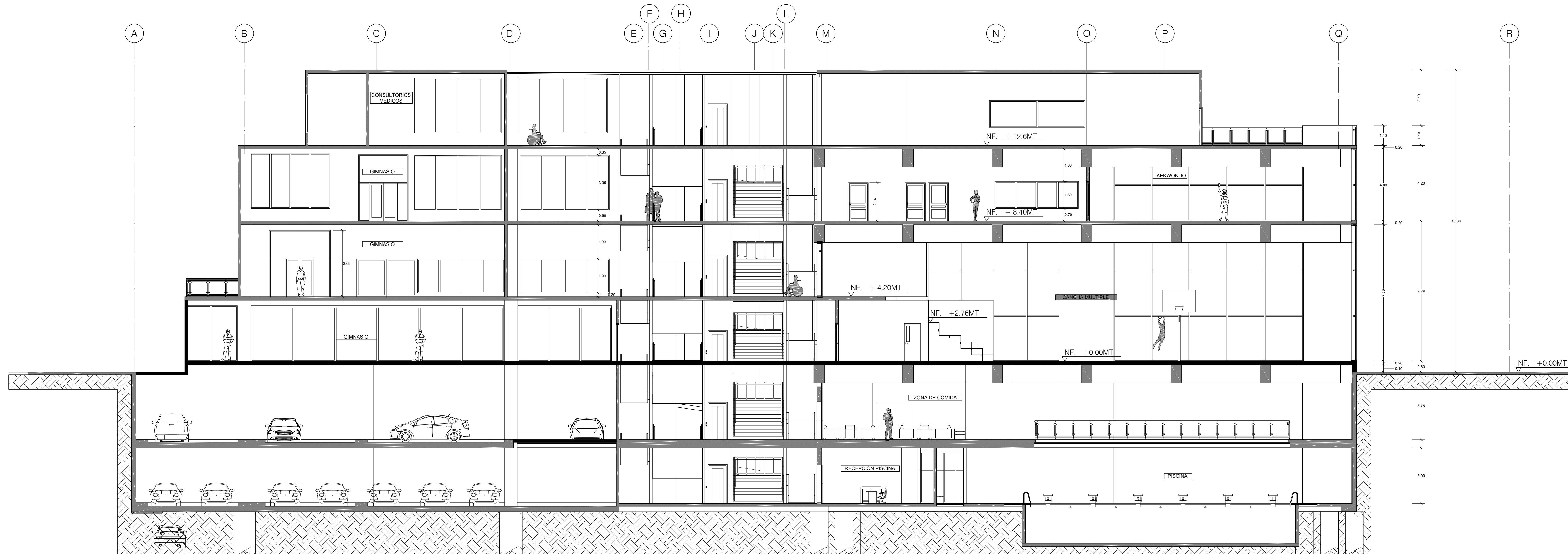
A CORTE 4 ESCALA 1:100
