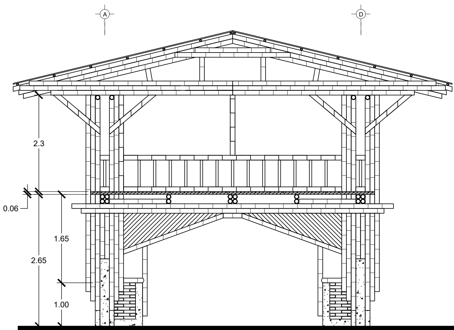
FACHADA OESTE
