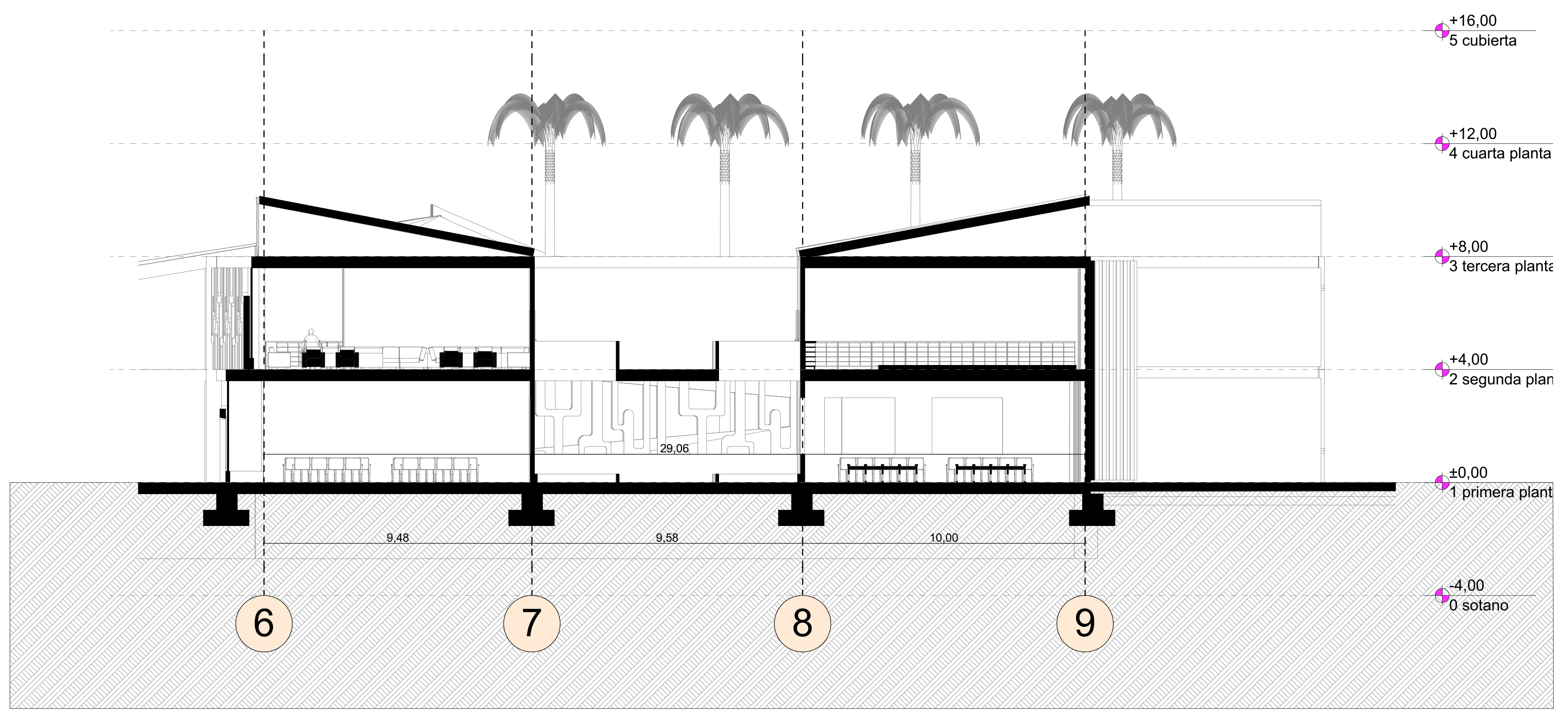
S-05 Seccion Modulo inclusividad Esc 1:100
