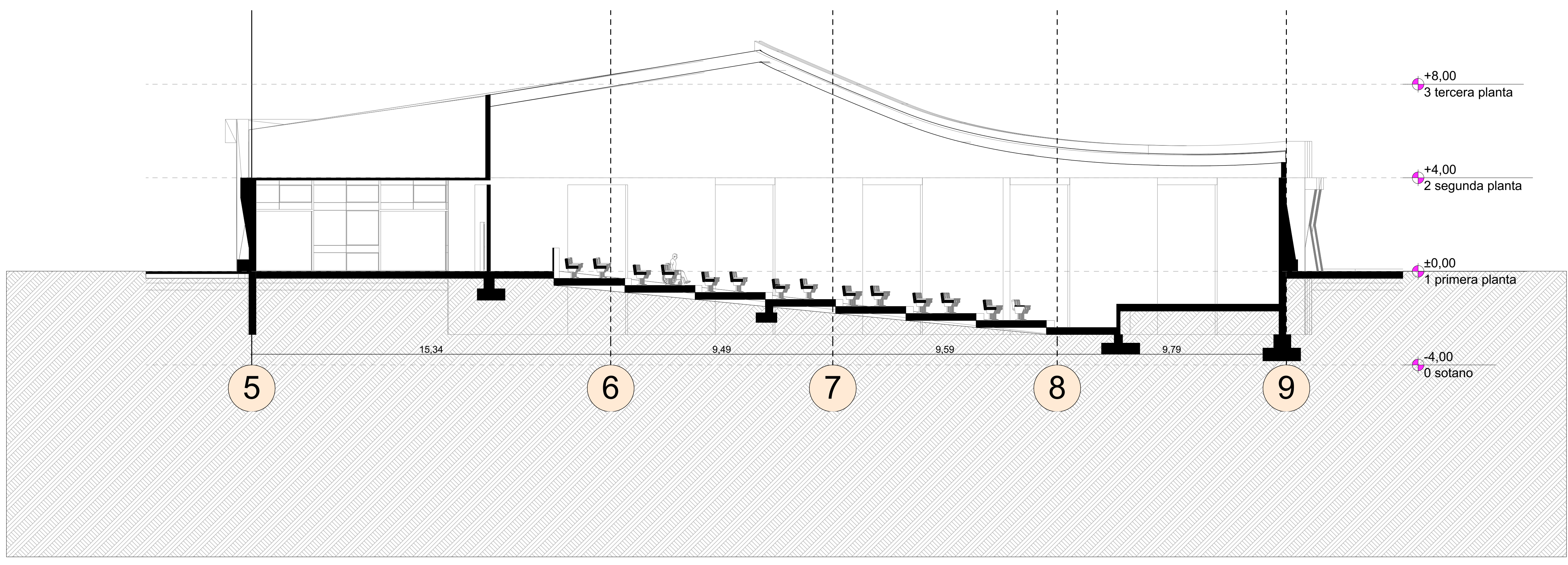
S-07 Seccion Auditorio Esc 1:100
