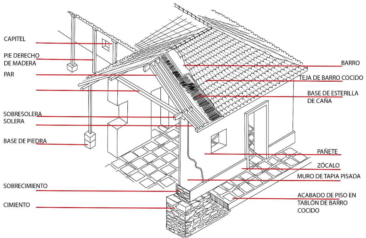
Ilustración 25 cartilla, técnicas de construcción tradicionales con tierra, ministerio de cultura, 2008.
