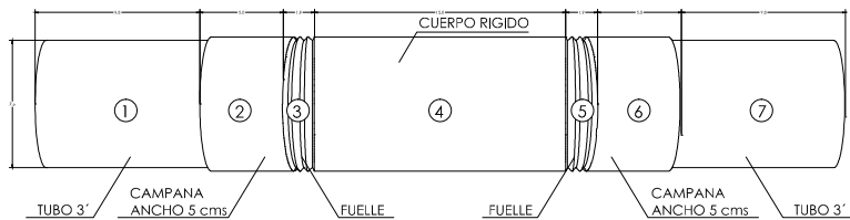
VISTA SUPERIOR ESC: 1/100
