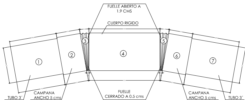
VISTA LATERAL ESC: 1/100
