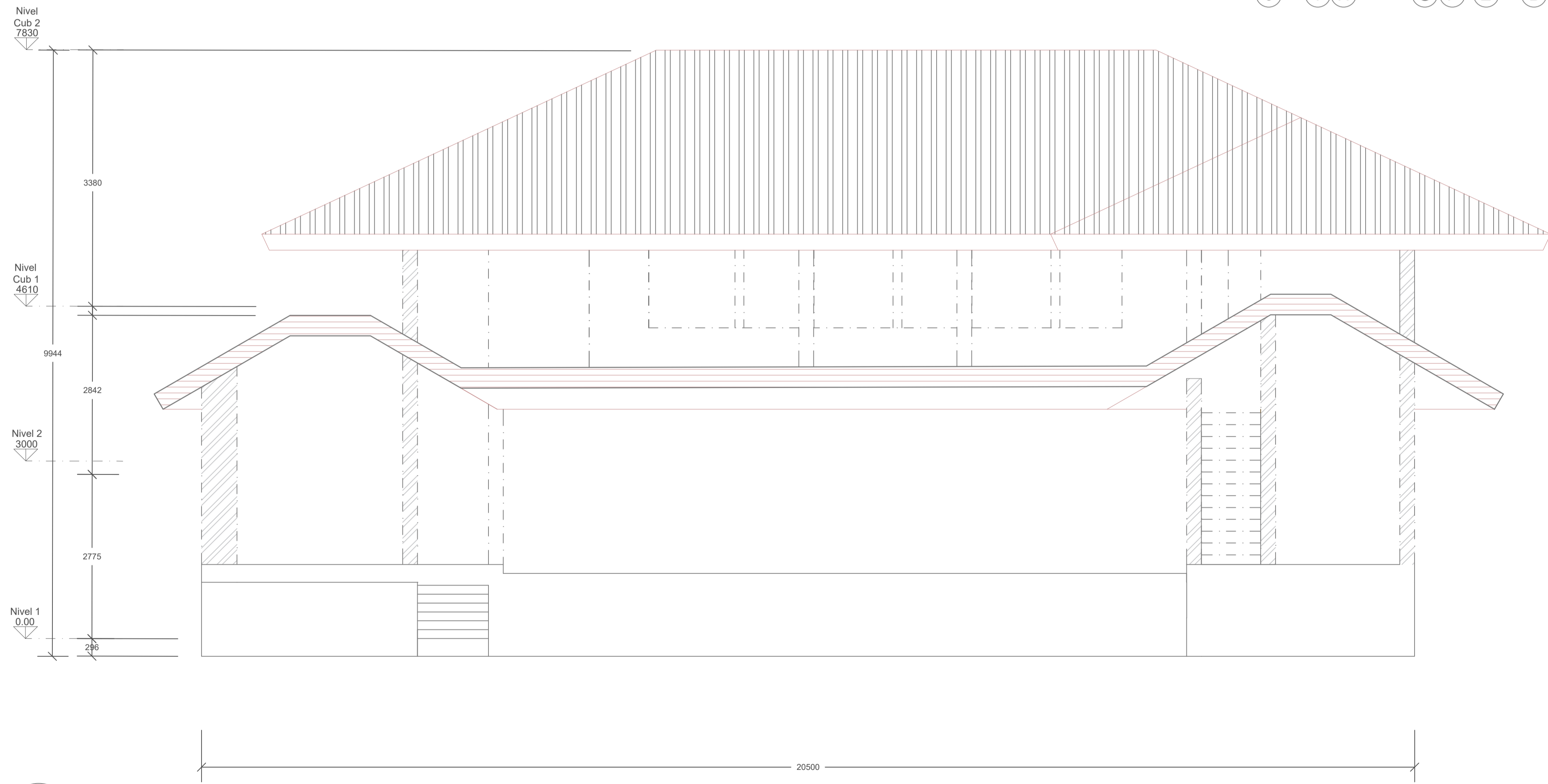
C-1 CORTE TRANSVERSAL ESCALA: 1:50
