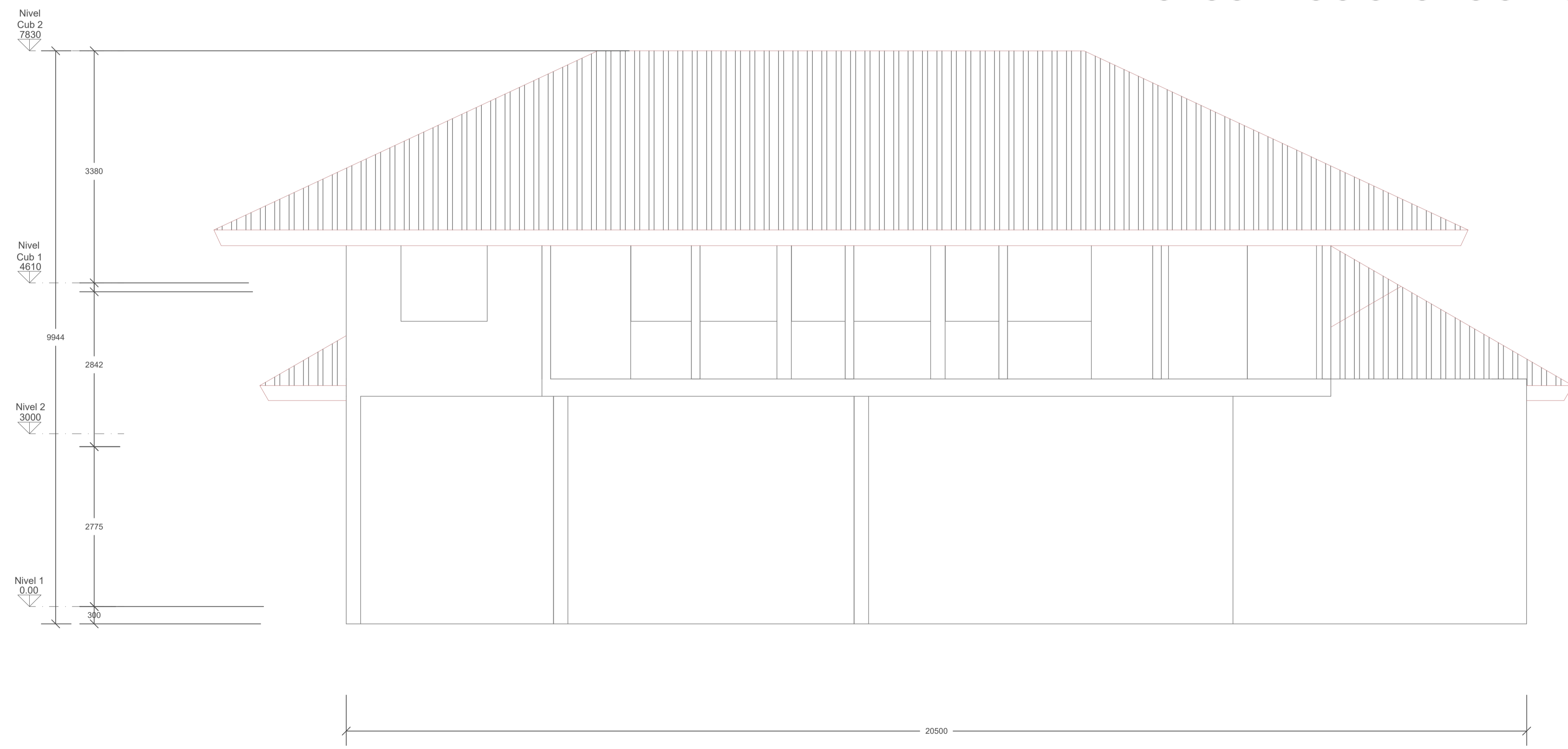
A-2 FACHADA NORTE ESCALA: 1:50
