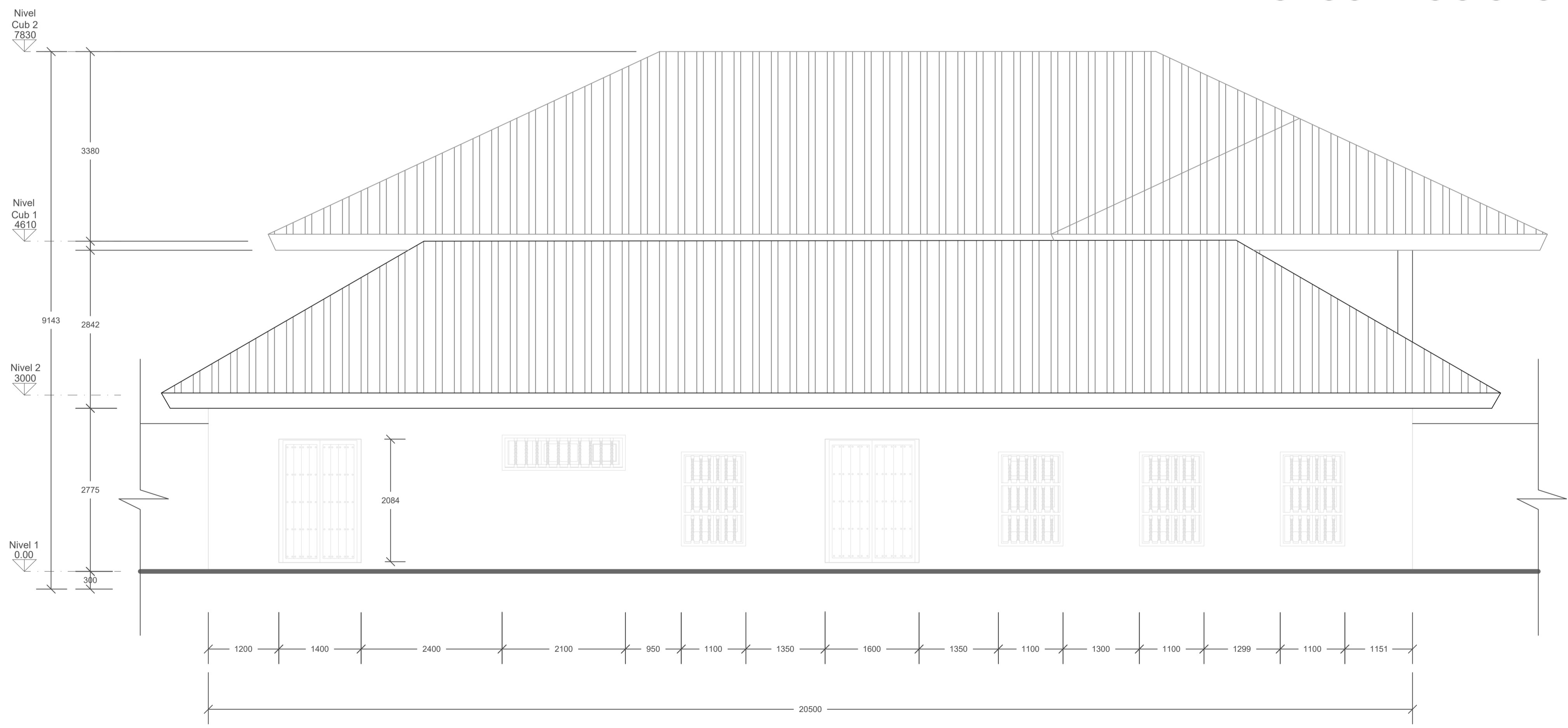
A-1 FACHADA SUR ESCALA: 1:50
