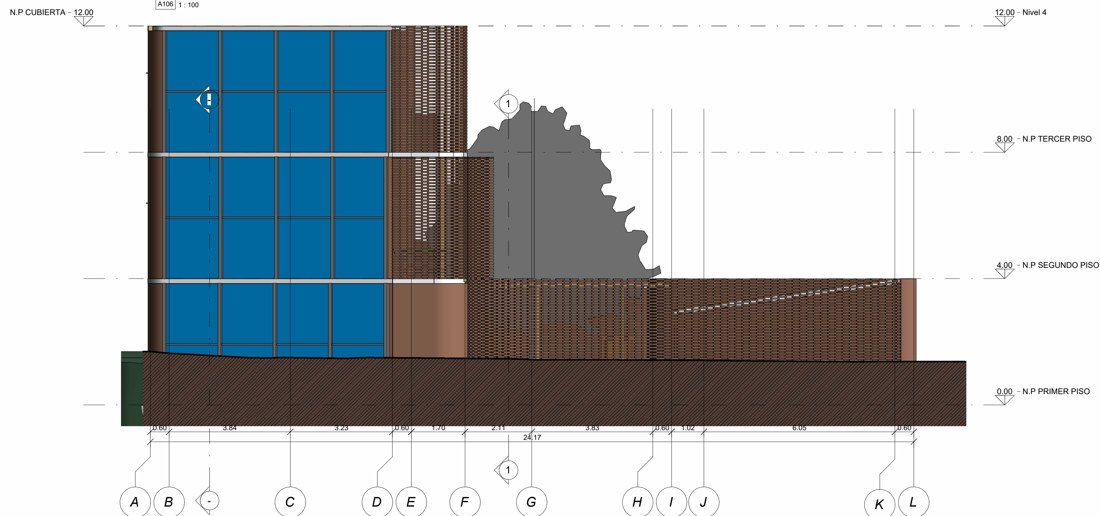
2 FACHADA OESTE A106 1: 75
