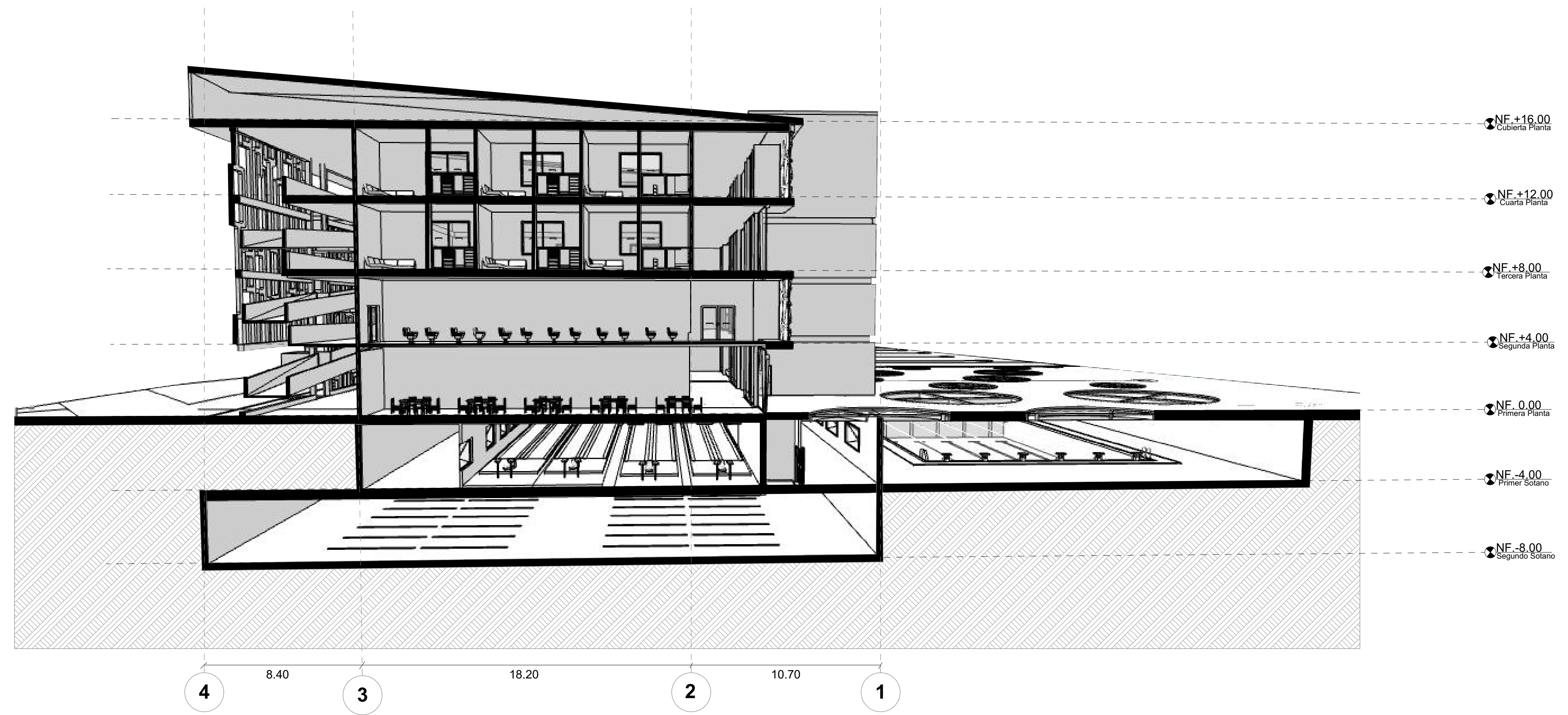
S-01 Seccion Fugada Bienestar Esc 1:200
