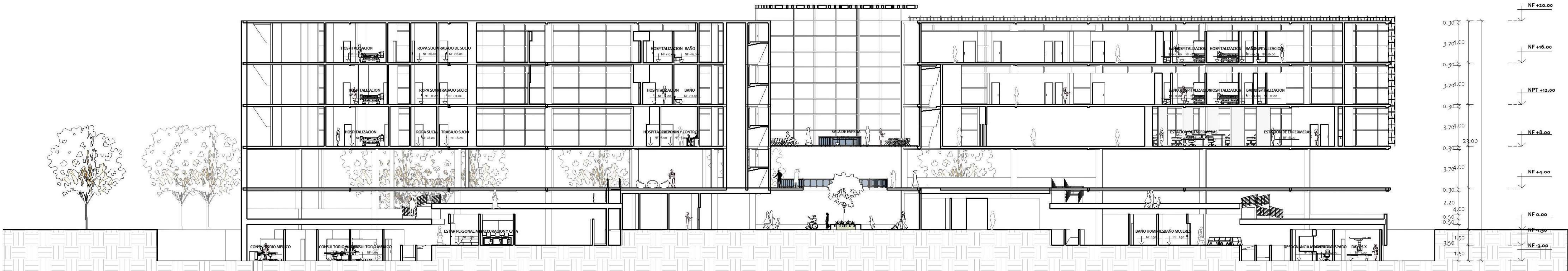
CORTE B-B
