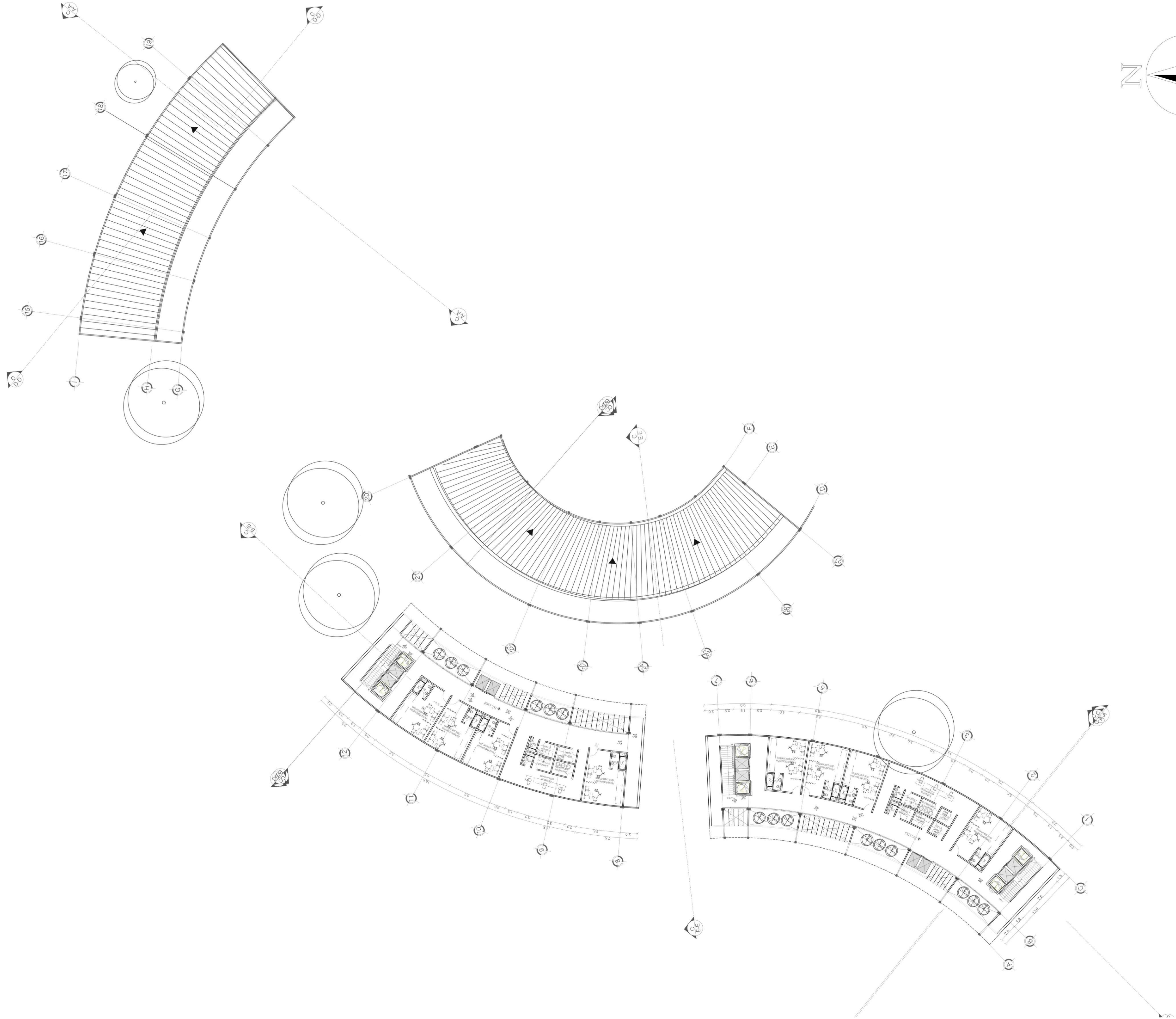
Planta Quinto Piso Escala 1:250 PP
