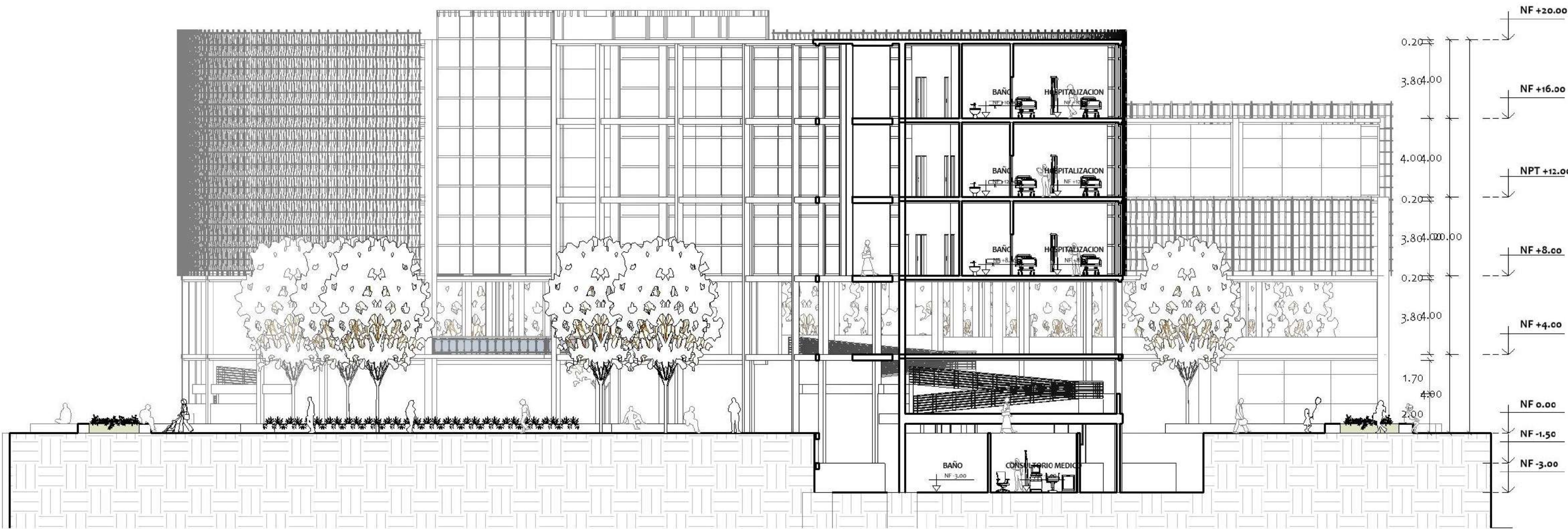
CORTE A-A
