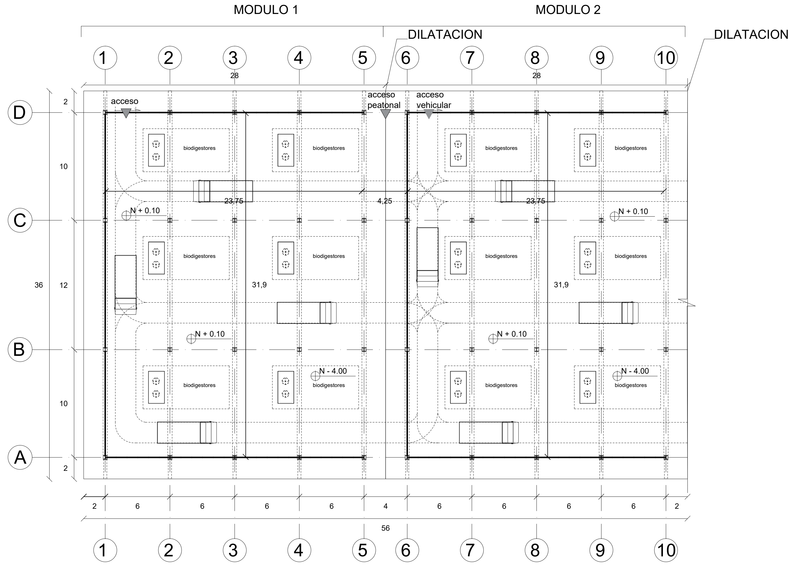
PRIMERA PLANTA ESCALA 1:200
