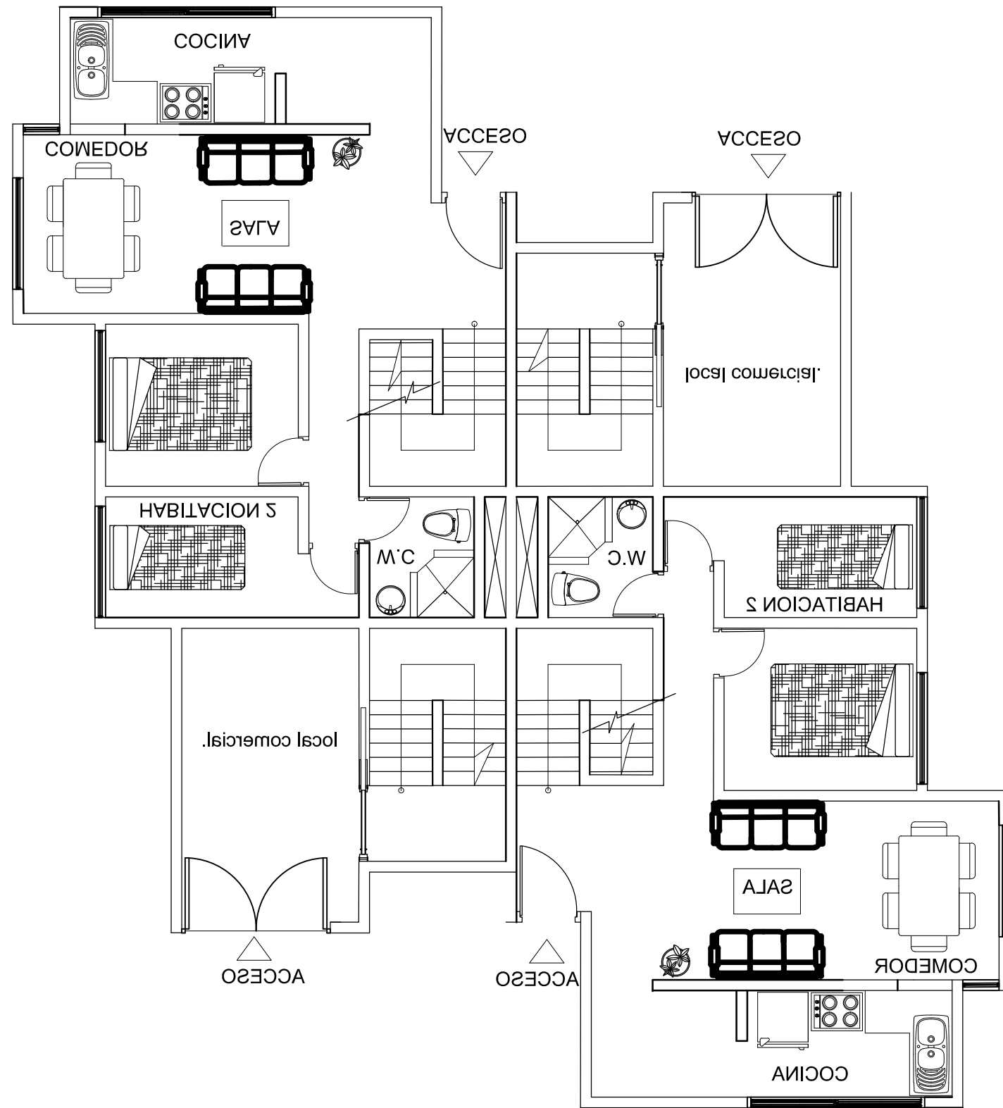
planta con desarrollo progresivo zona comercio Esc.1.75
