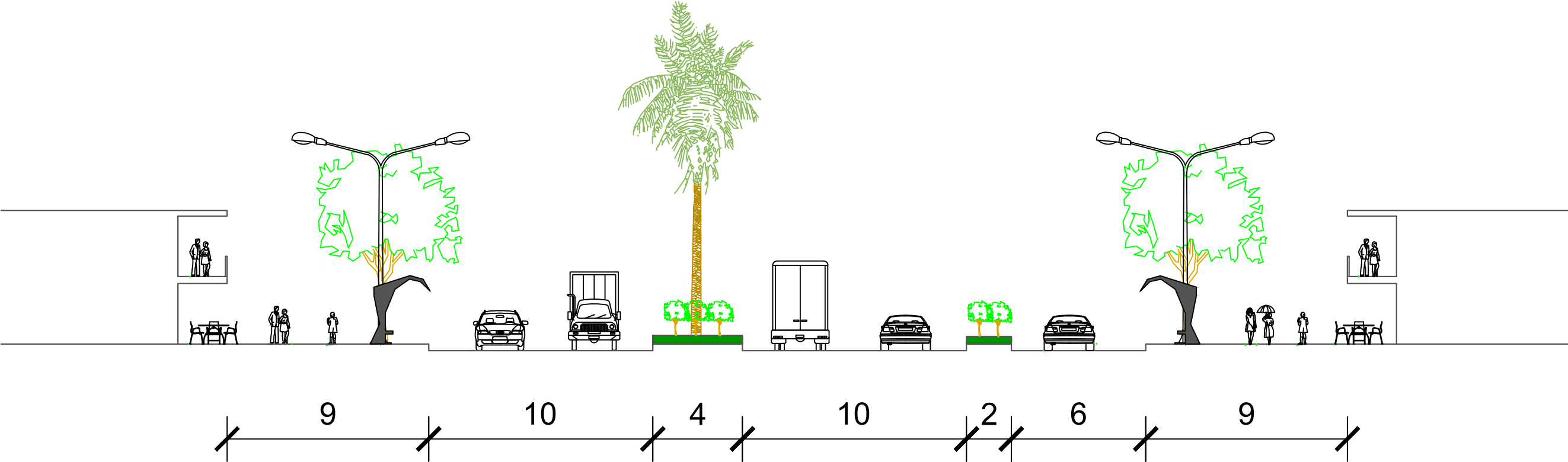
C CORTE VIA PANAMERICA - BULEVAR ESC 1:200
