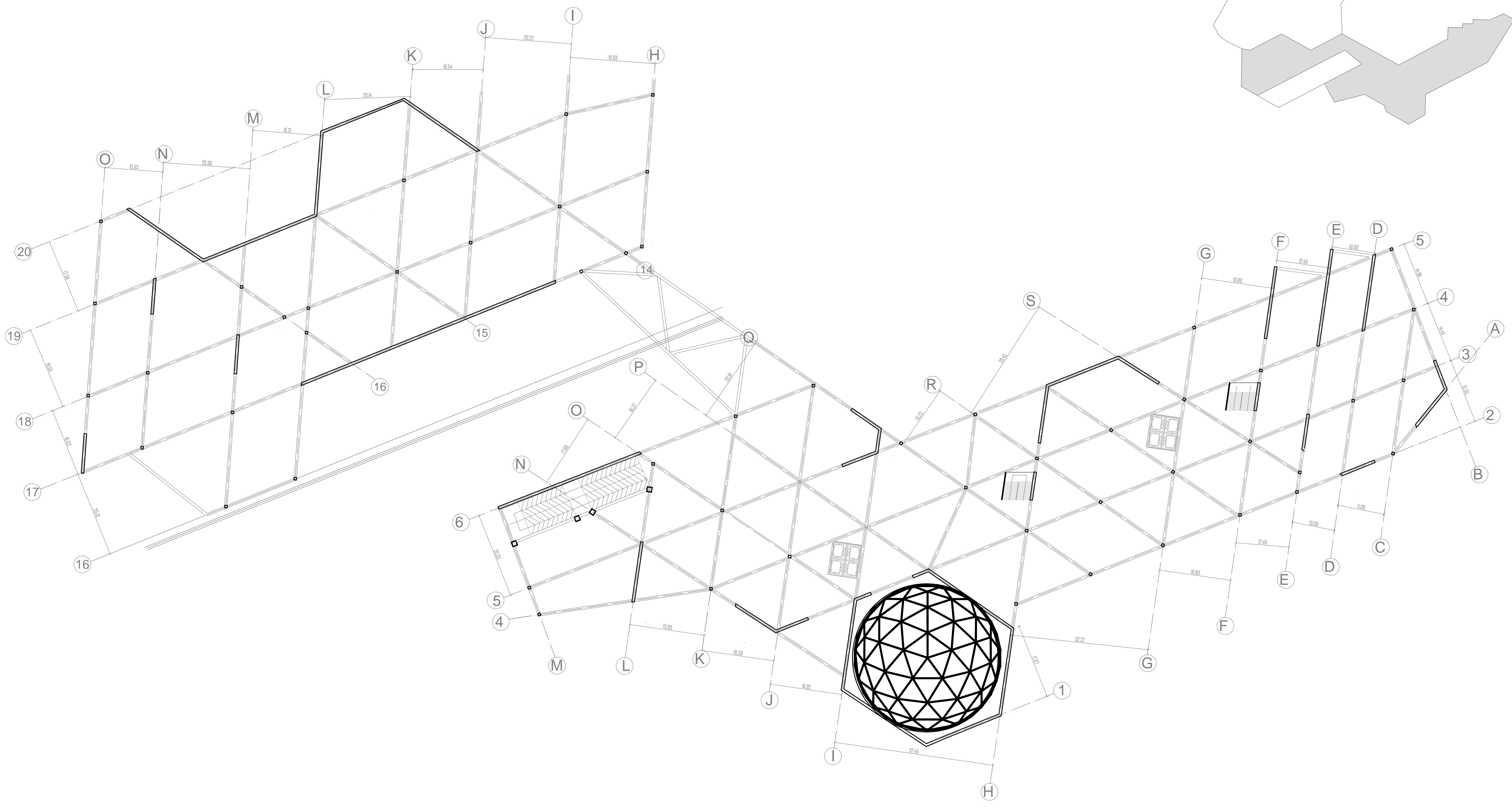
E2 PLANTA ESTRUCTURAL ENTREPISO - CUBIERTAS DE ASAMBLEAS- ESTACION DEL TREN ESCALA 1:400
