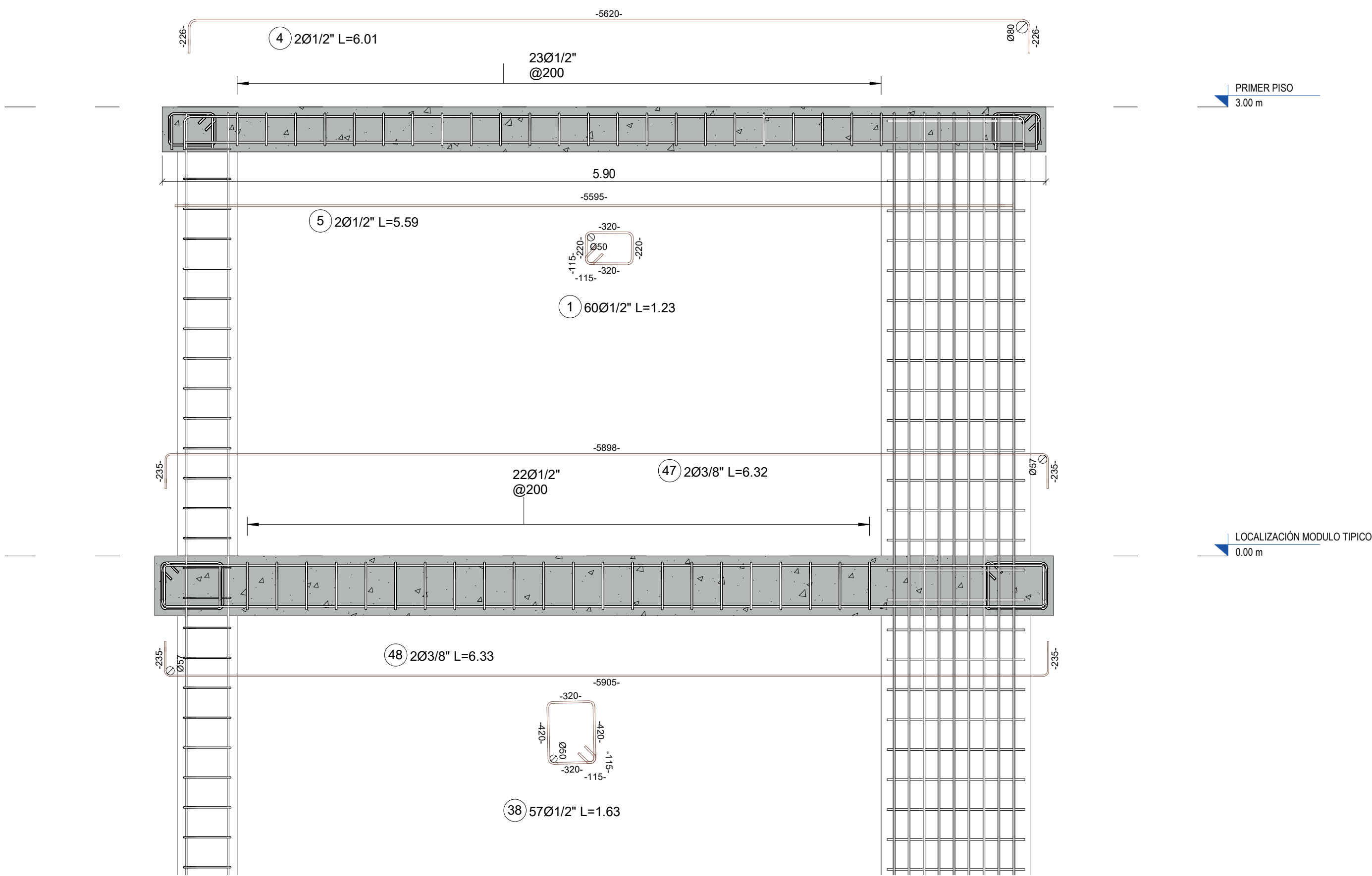
CORTE N+3.00 ESC 1 : 25
