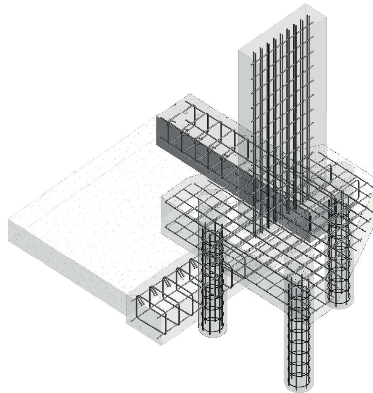
ISOMETRICO DE DETALLE 2 ESC
