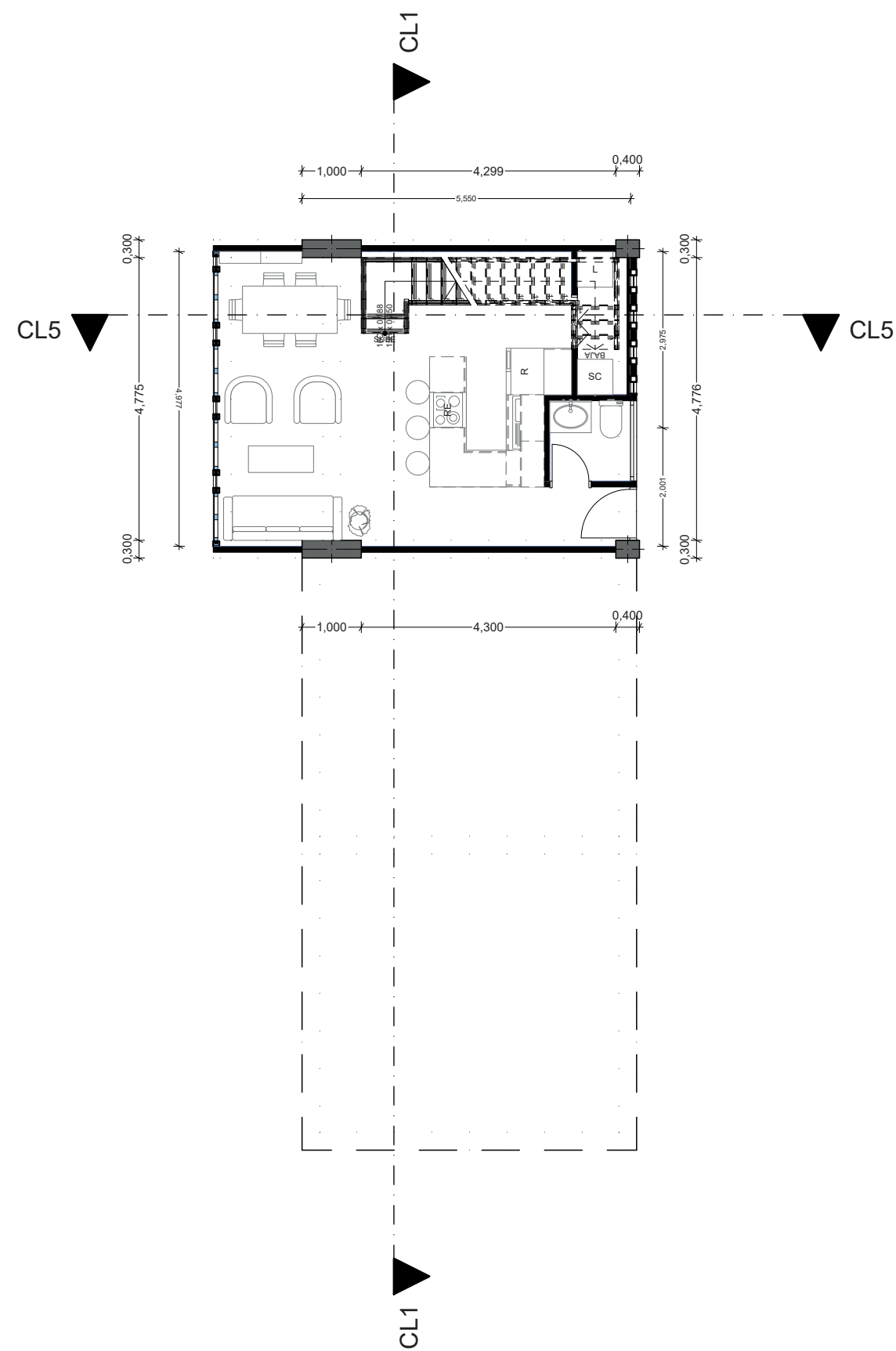
PLANTA 1
