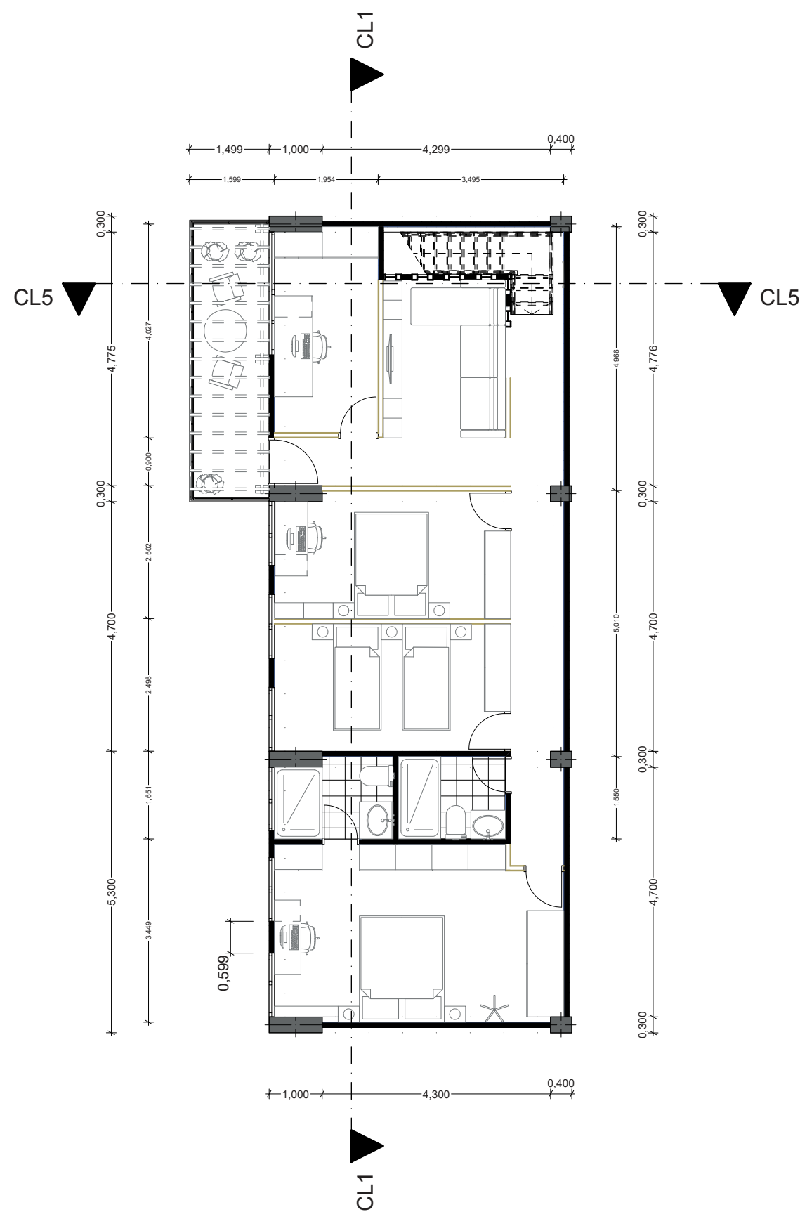
PLANTA 2
