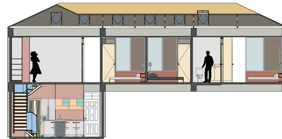
SECCION CL1
