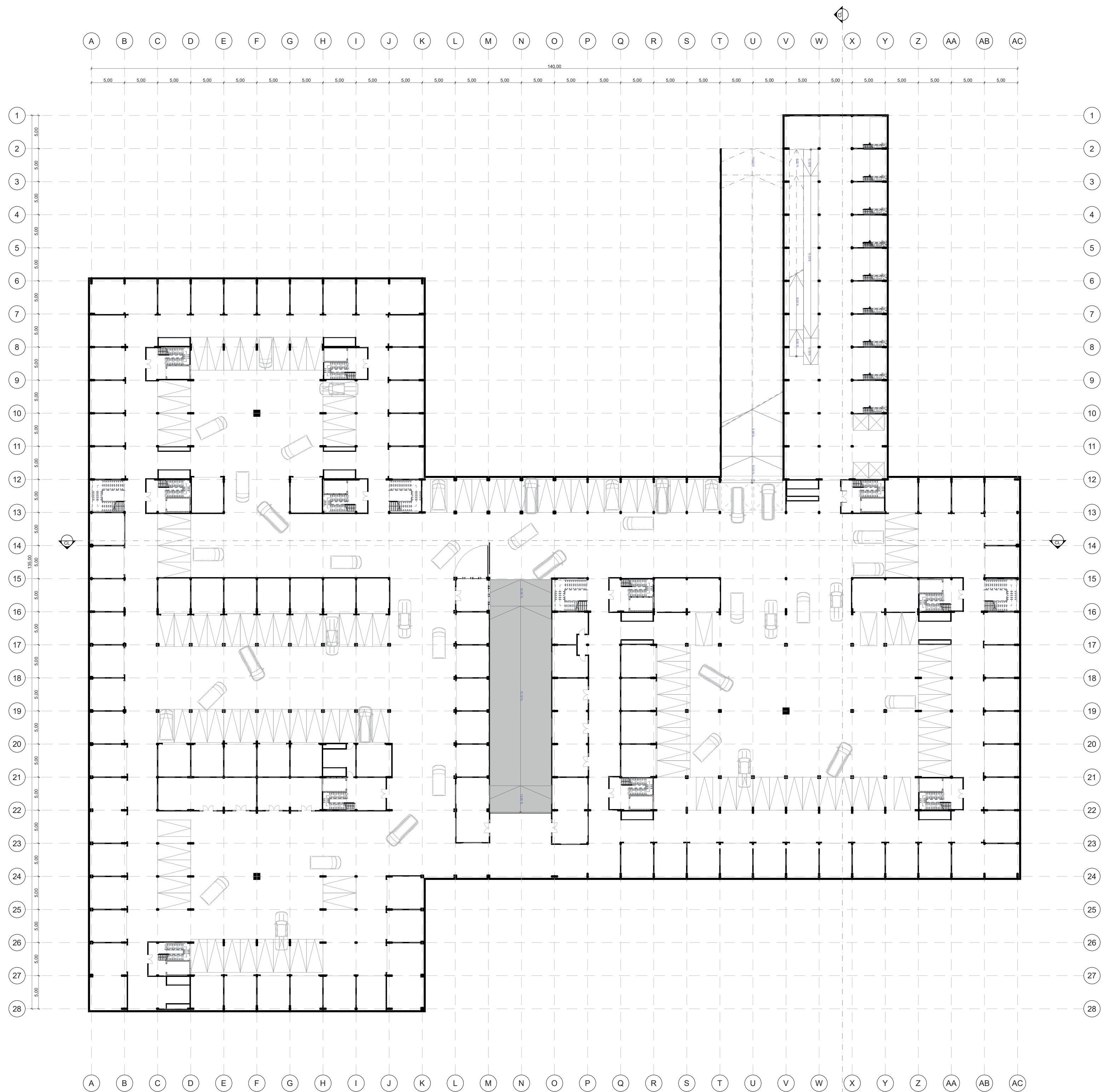
P0 PLANTA SOTANO SUPERIOR ESC 1:400
