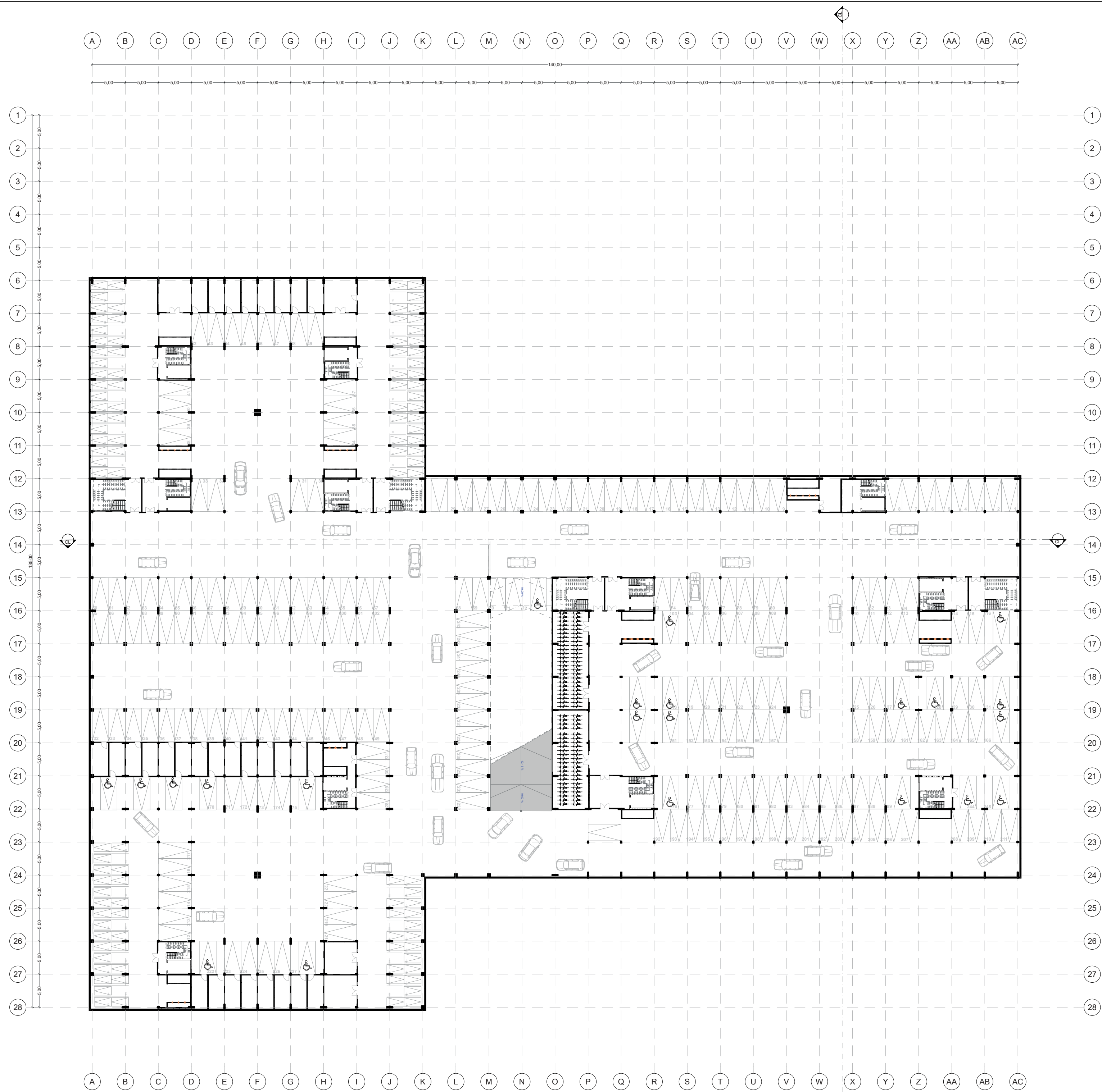
P0 PLANTA SOTANO INFERIOR ESC 1:400
