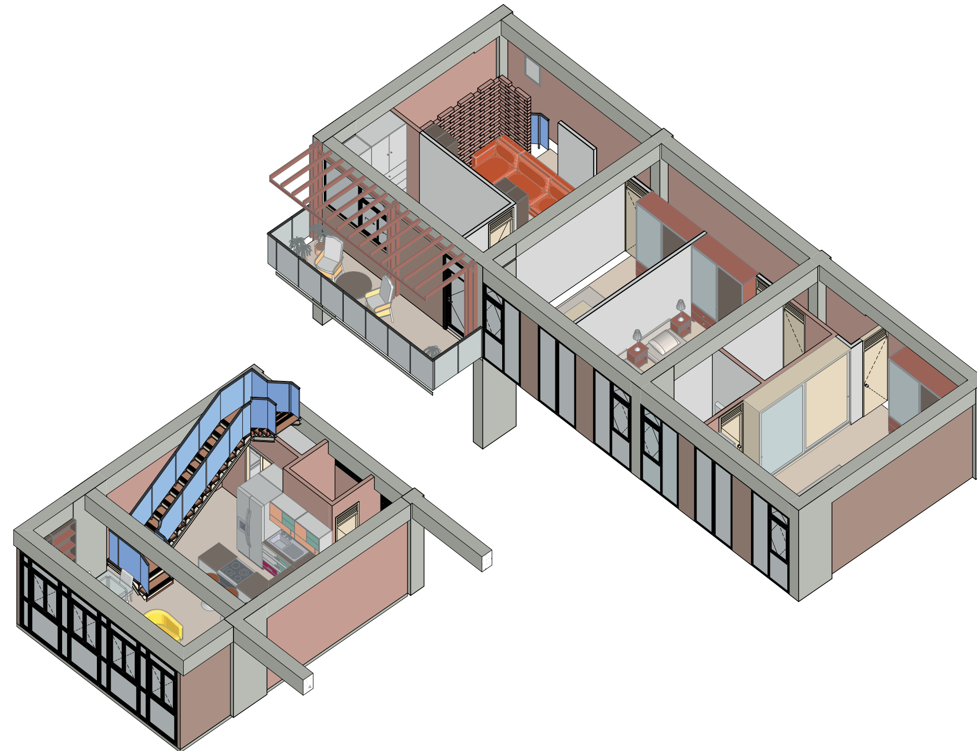
SECCION CL1
