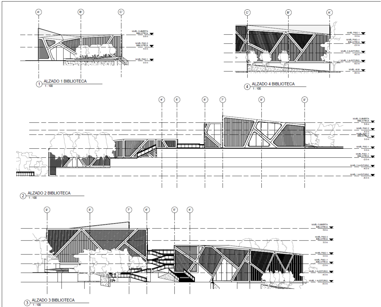
Figura 32, Elaboración propia mediante Revit, alzados de volumen auditorio y biblioteca.
