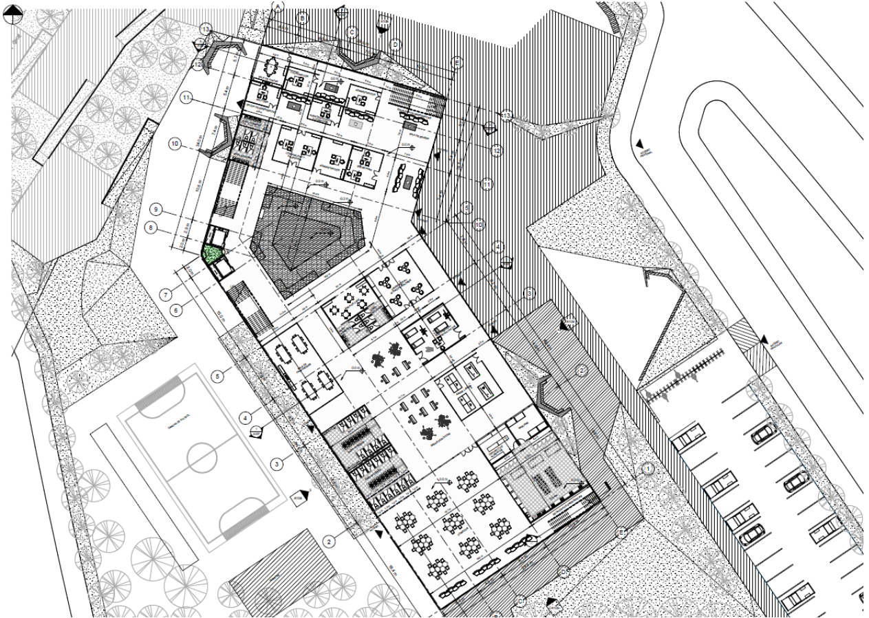
Imagen 27, elaboración propia, mediante Revit, Planta del primer piso bloque central.
