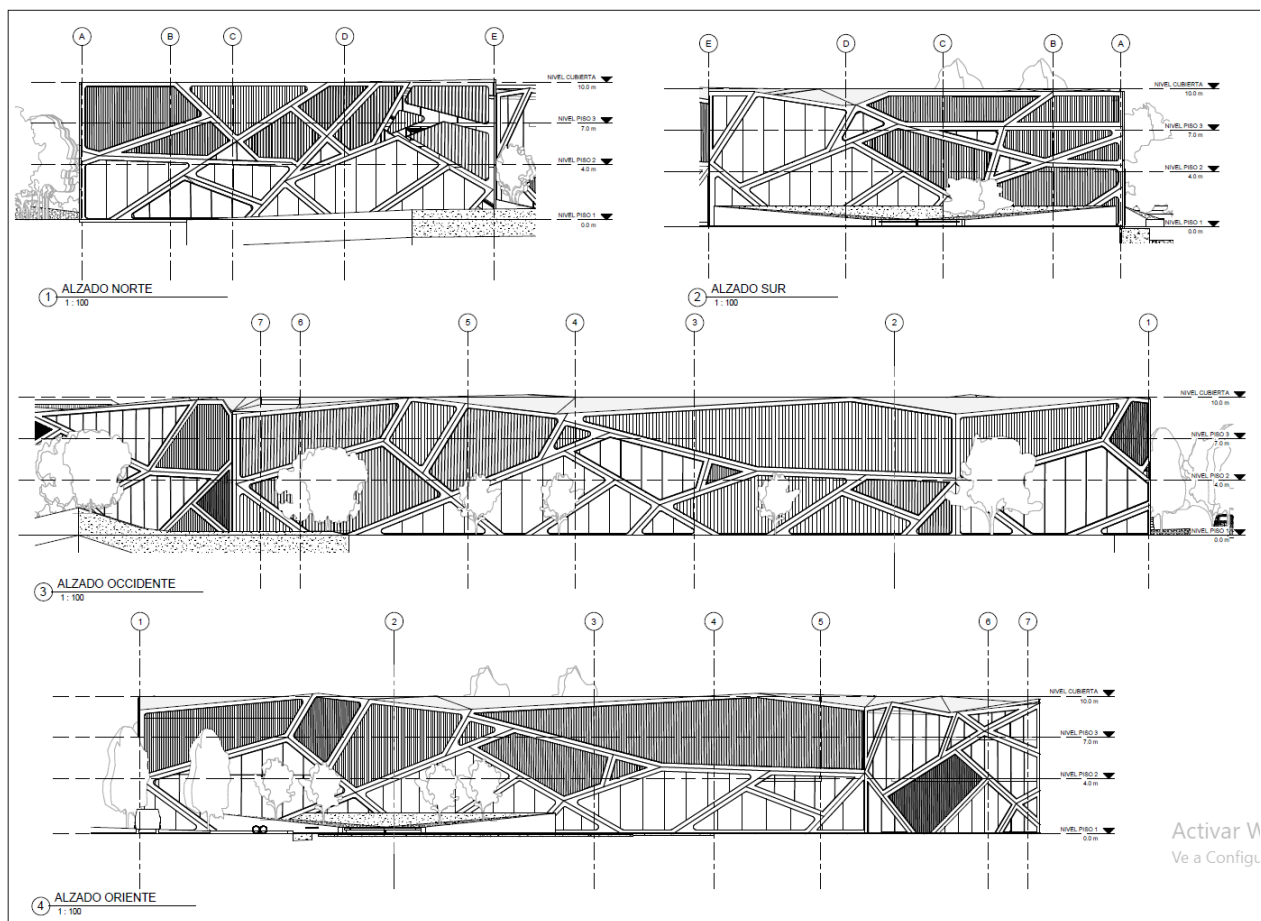
Figura 31, Elaboración propia mediante Revit, alzados del volumen principal.
