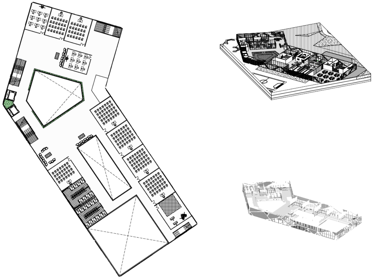
Imagen 28, Elaboración propia mediante revit, planta segundo nivel con axonometria de dicha planta.
