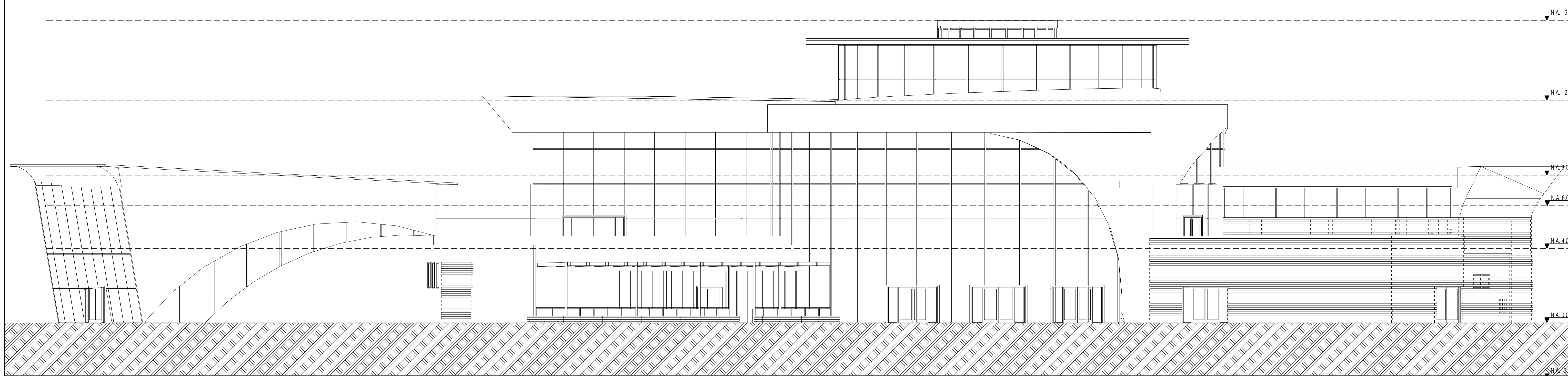
FACHADA NORTE ESCALA: 1:100
