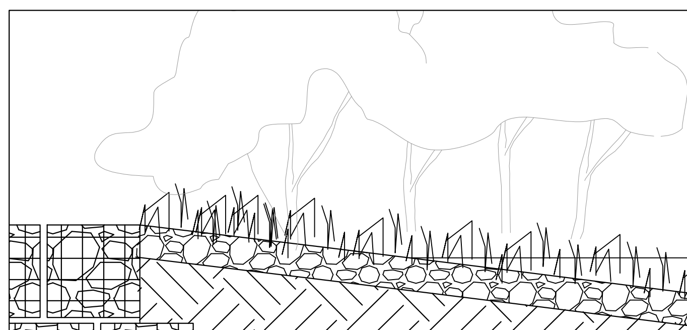
P43 DETALLE PASOS PEATONALES
