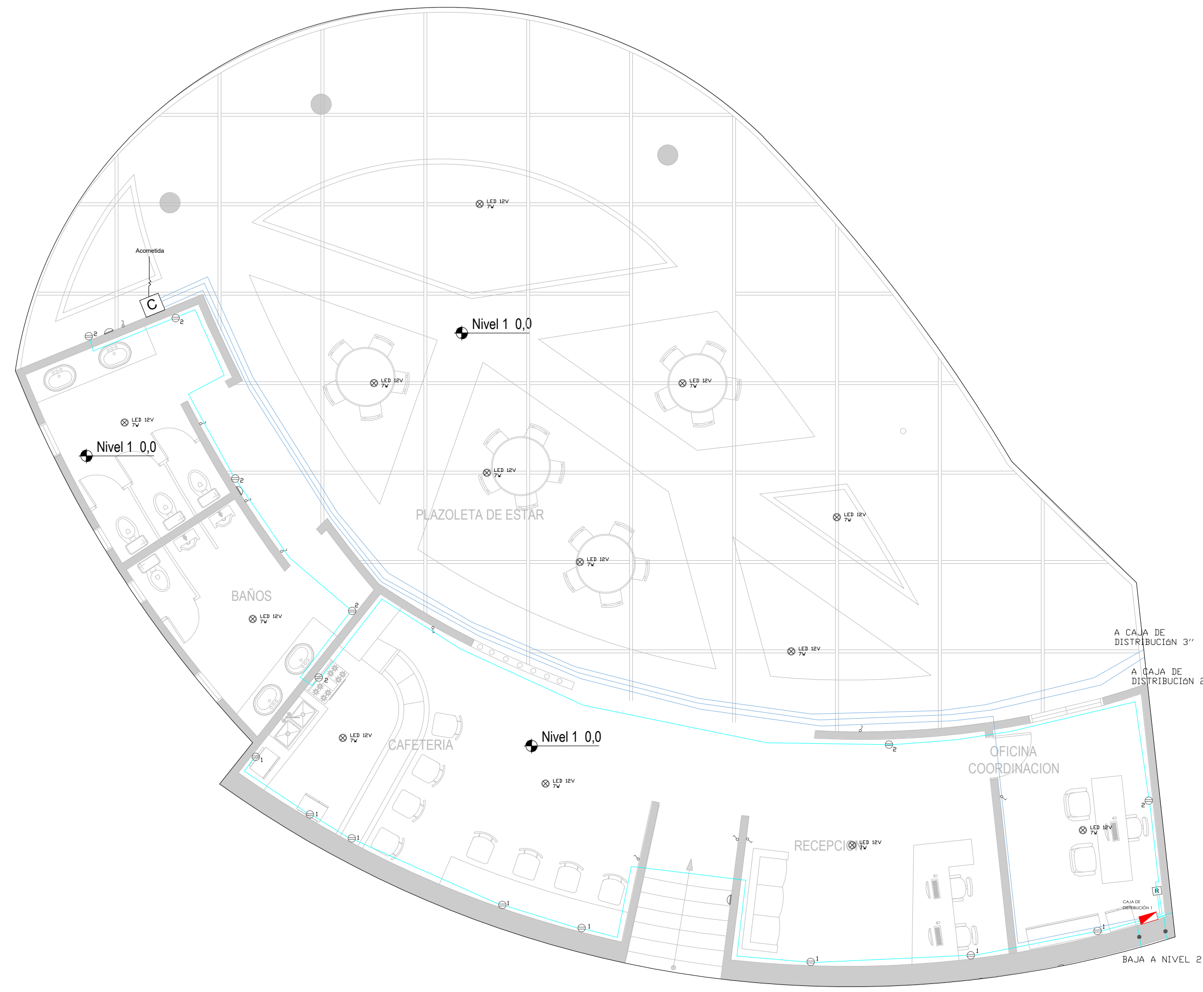
0. PLANTA NIVEL 1 DISTRIBUCIÓN DE TOMAS 1:75
