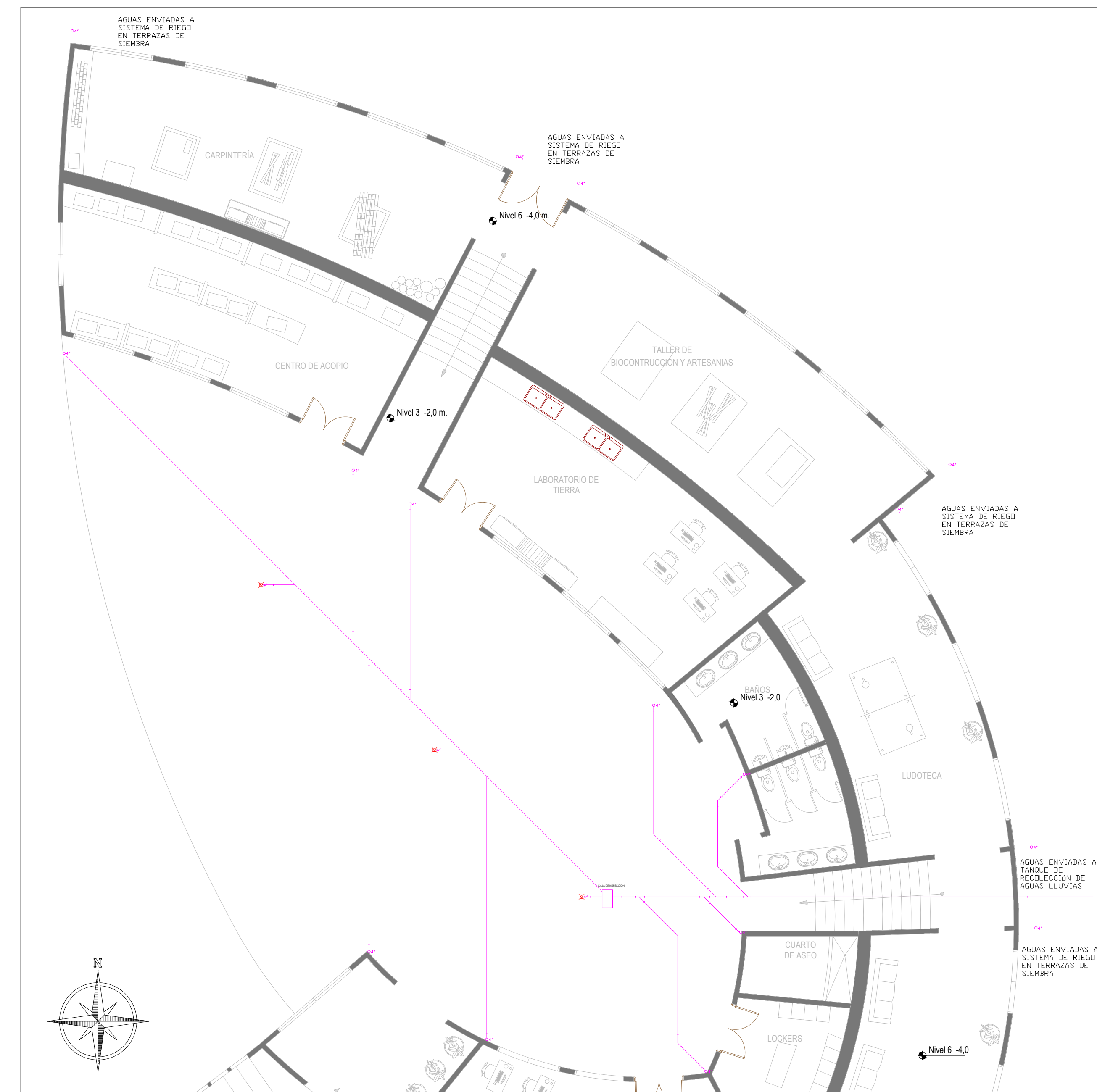
AGUAS LLUVIAS PLAZOLETA DE TALLERES
