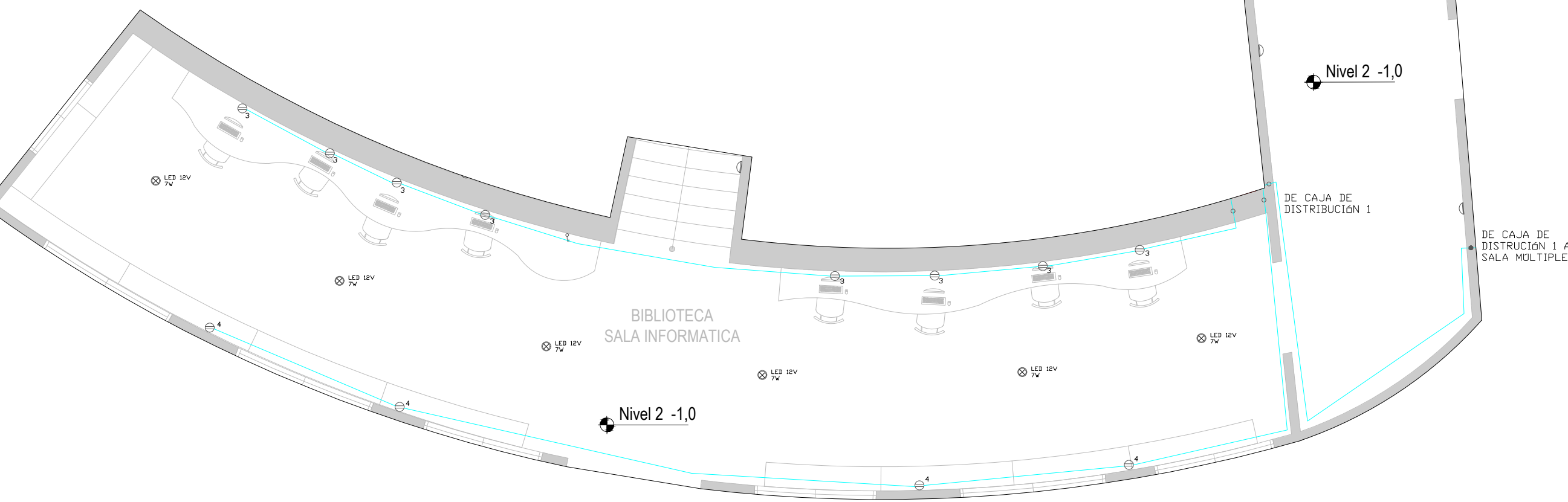
0. PLANTA NIVEL 2 DISTRIBUCIÓN DE TOMAS 1:75
