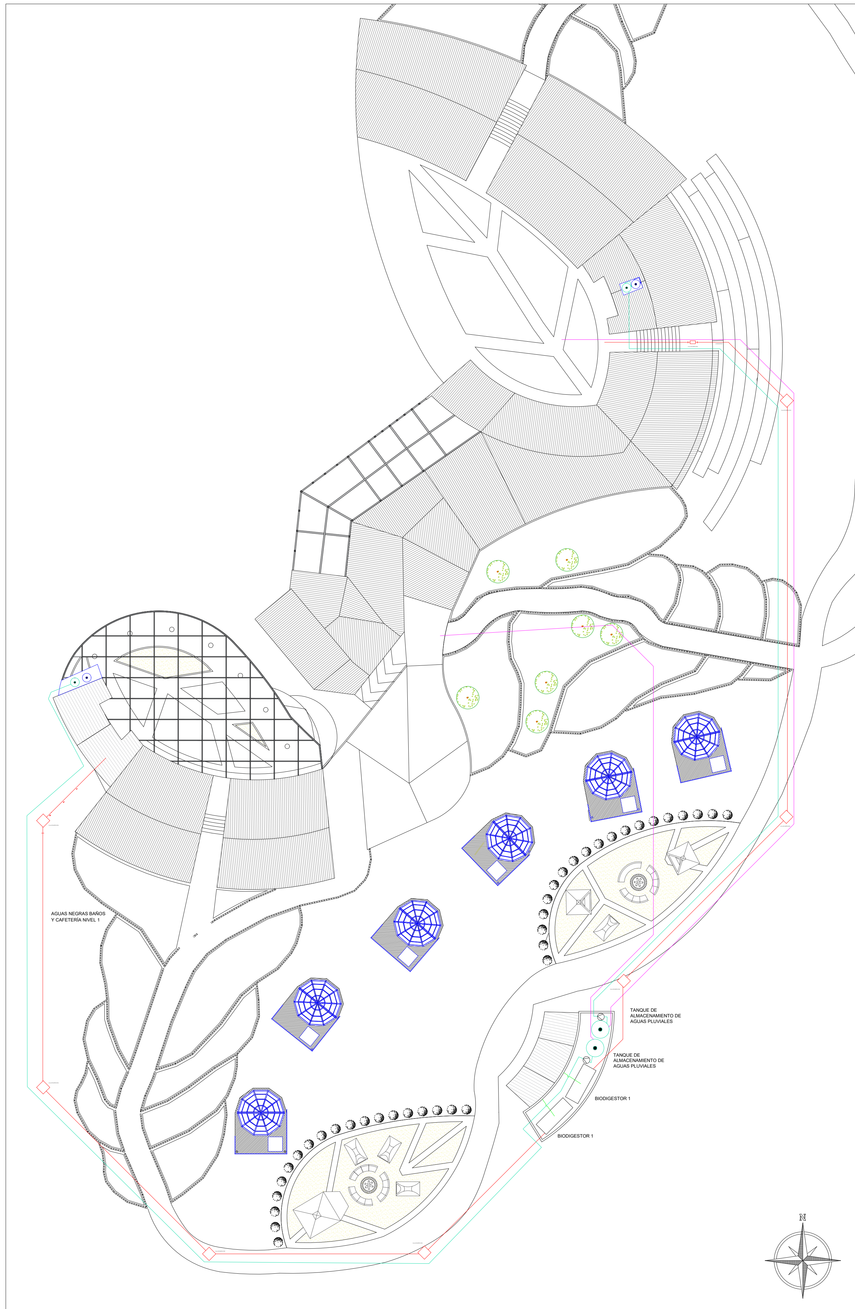
0. ALMACENAMIENTO Y REDISTRIBUCIÓN DE AGUAS NEGRAS Y PLUVIALES 1:200
