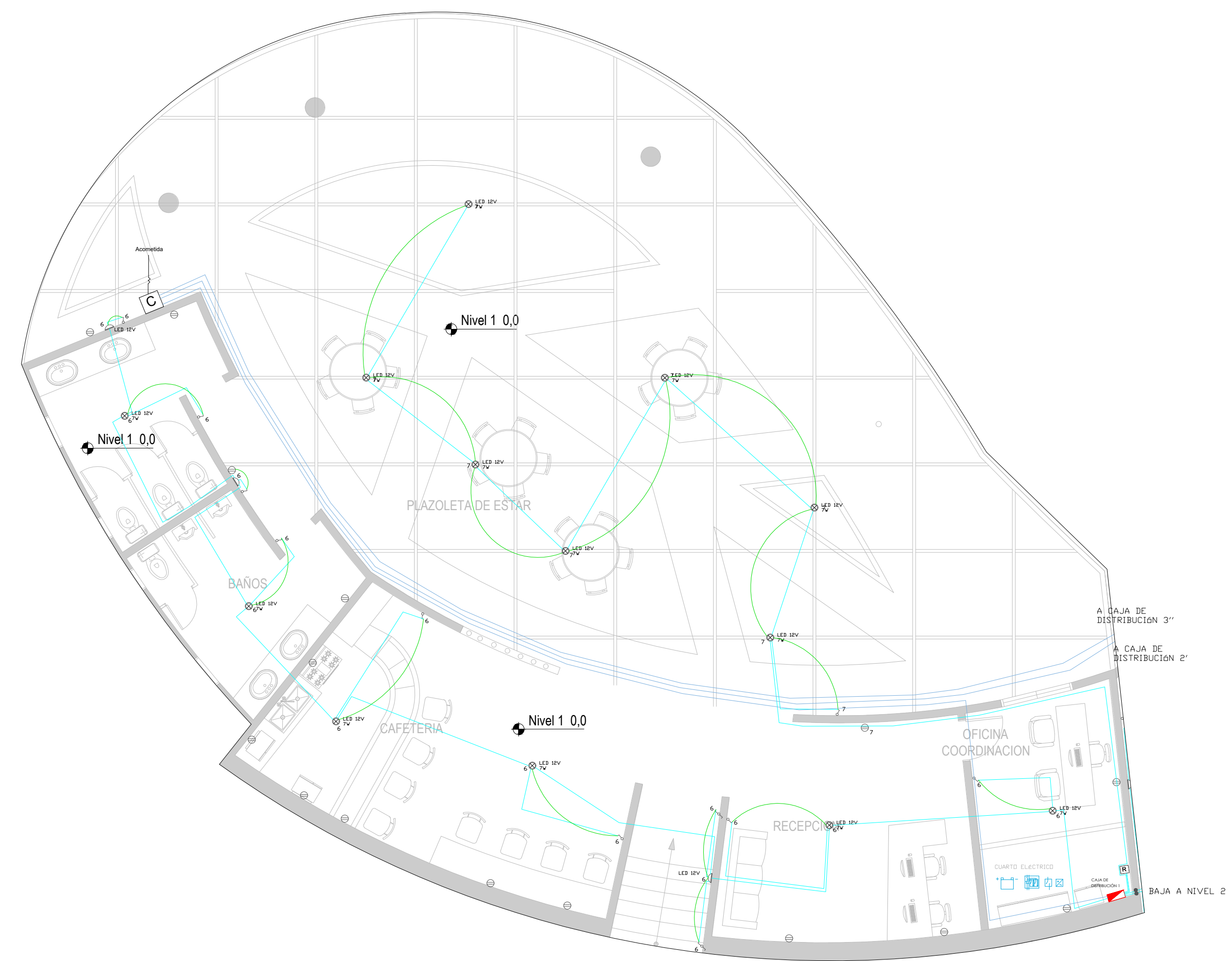
0. PLANTA NIVEL 1 DISTRIBUCIÓN LUMINARIAS E INTERRUPTORES 1:75
