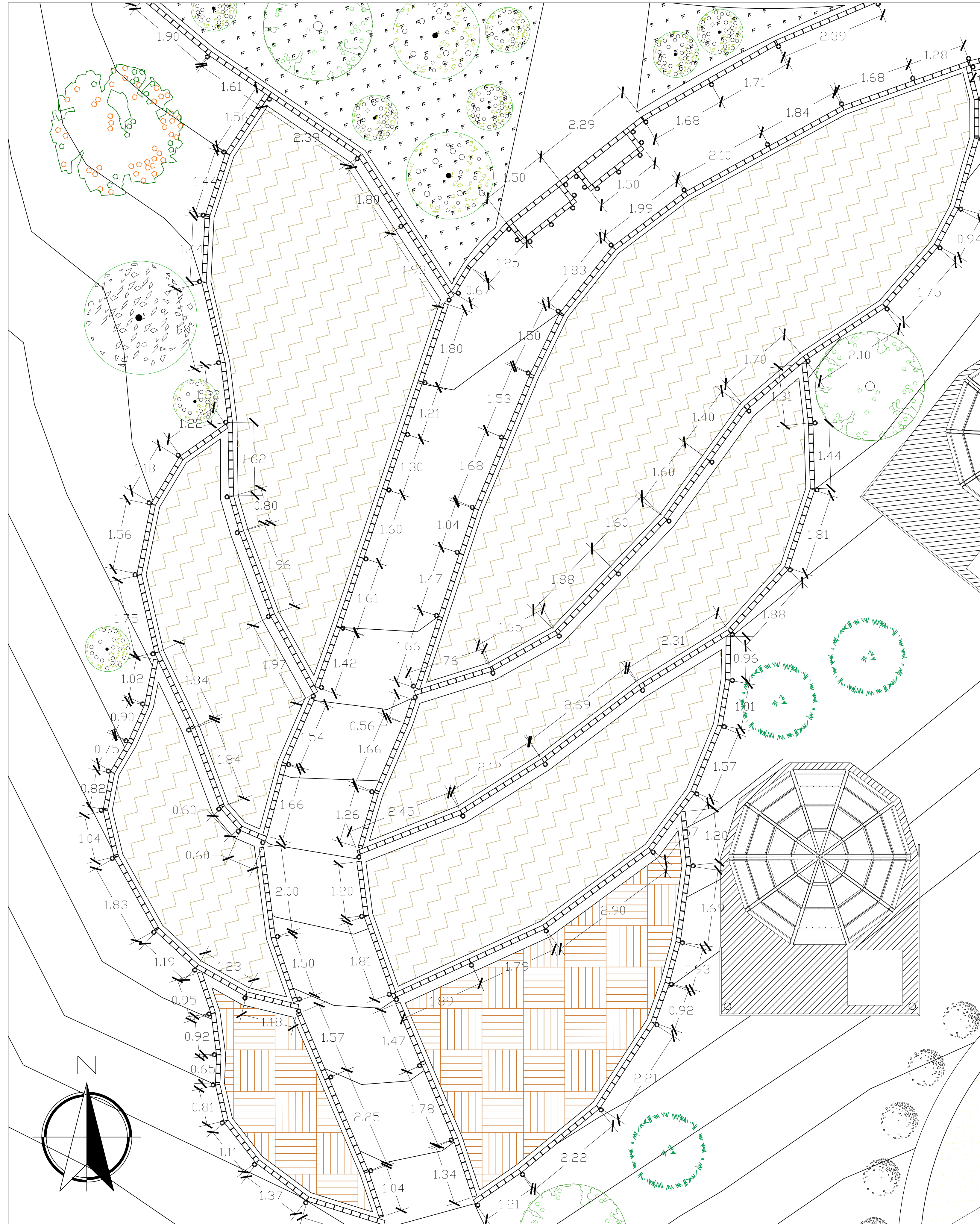
A DET. A015 TERRAZA DE SIEMBRA Esc. 1:50
