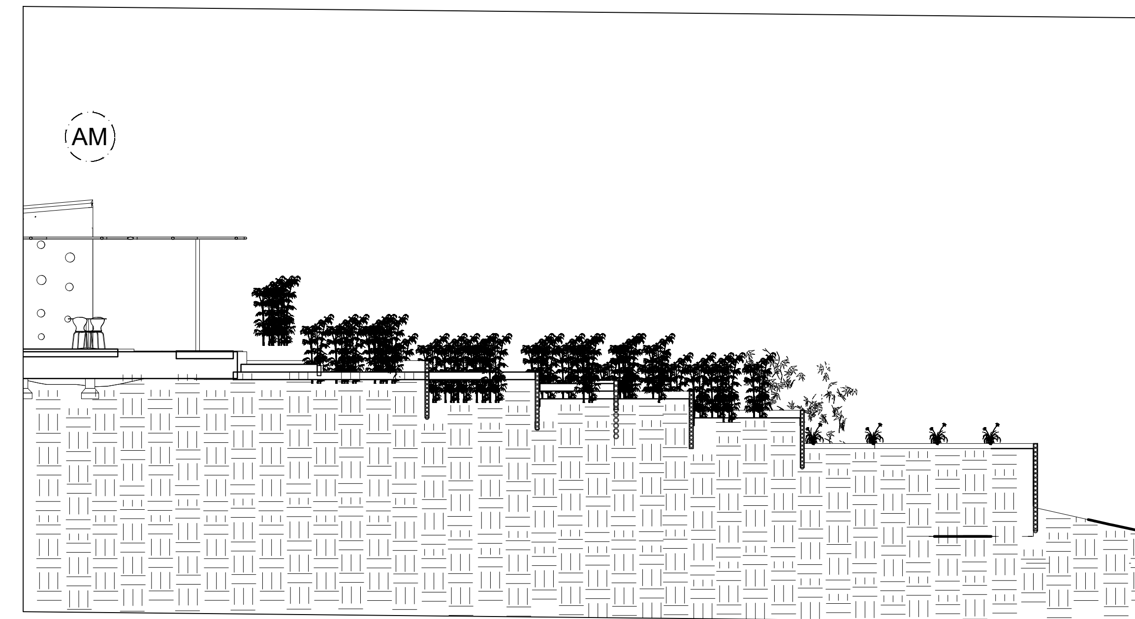
A CORTE TRANSVERSAL Esc. 1:100
