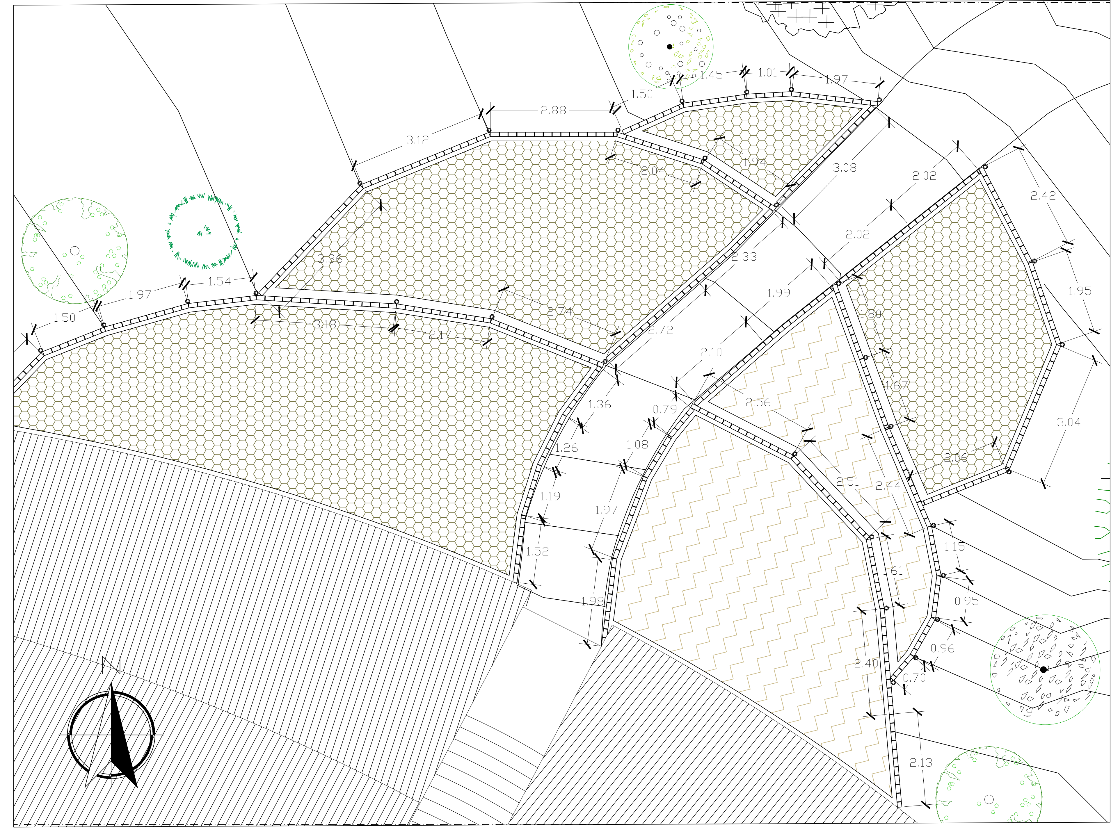
A DET. A017 TERRAZA DE SIEMBRA Esc. 1:150
