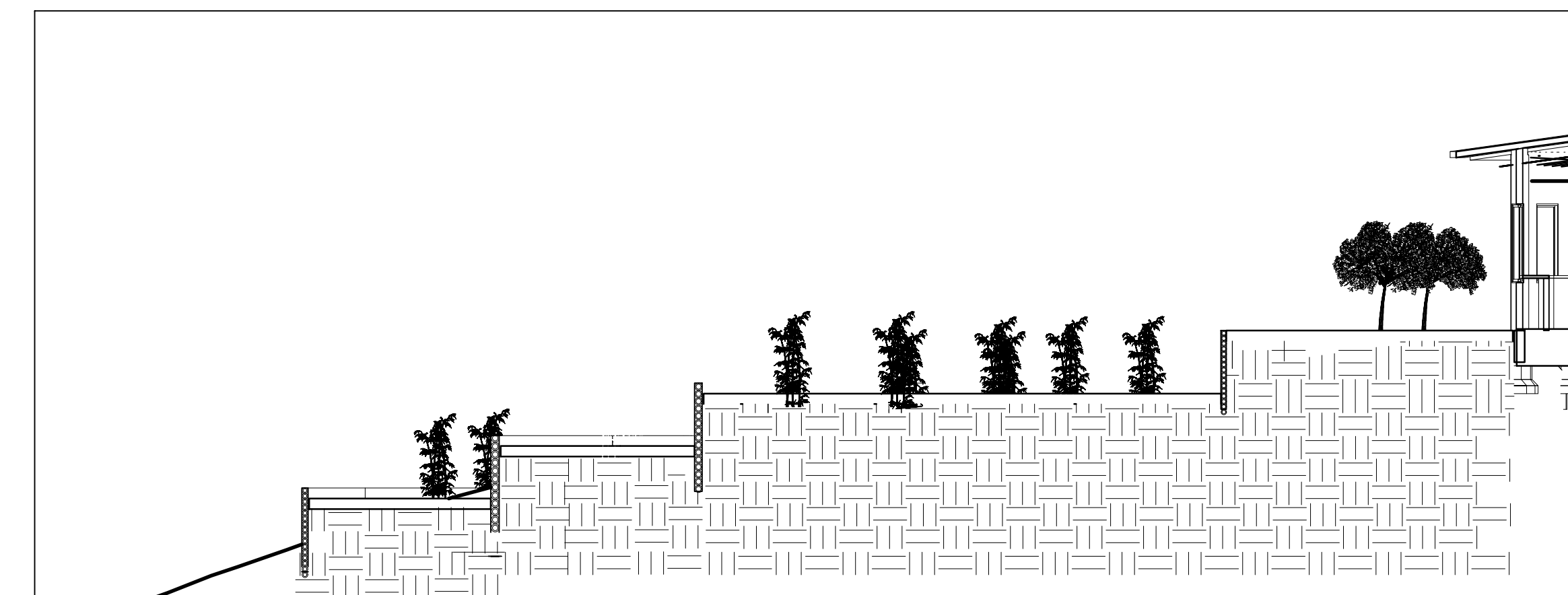
A CORTE TRANSVERSAL Esc. 1:100
