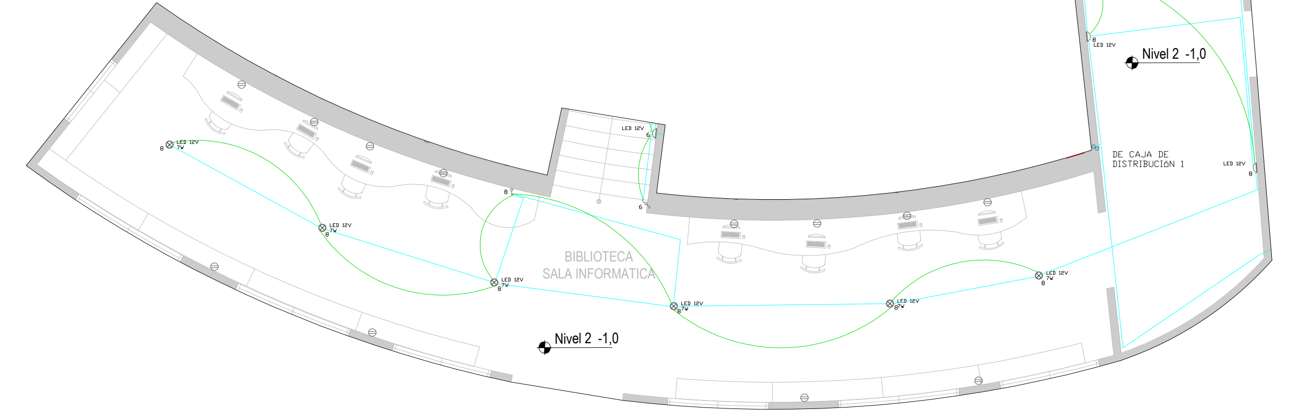
0. PLANTA NIVEL 2 DISTRIBUCIÓN LUMINARIAS E INTERRUPTORES 1:75
