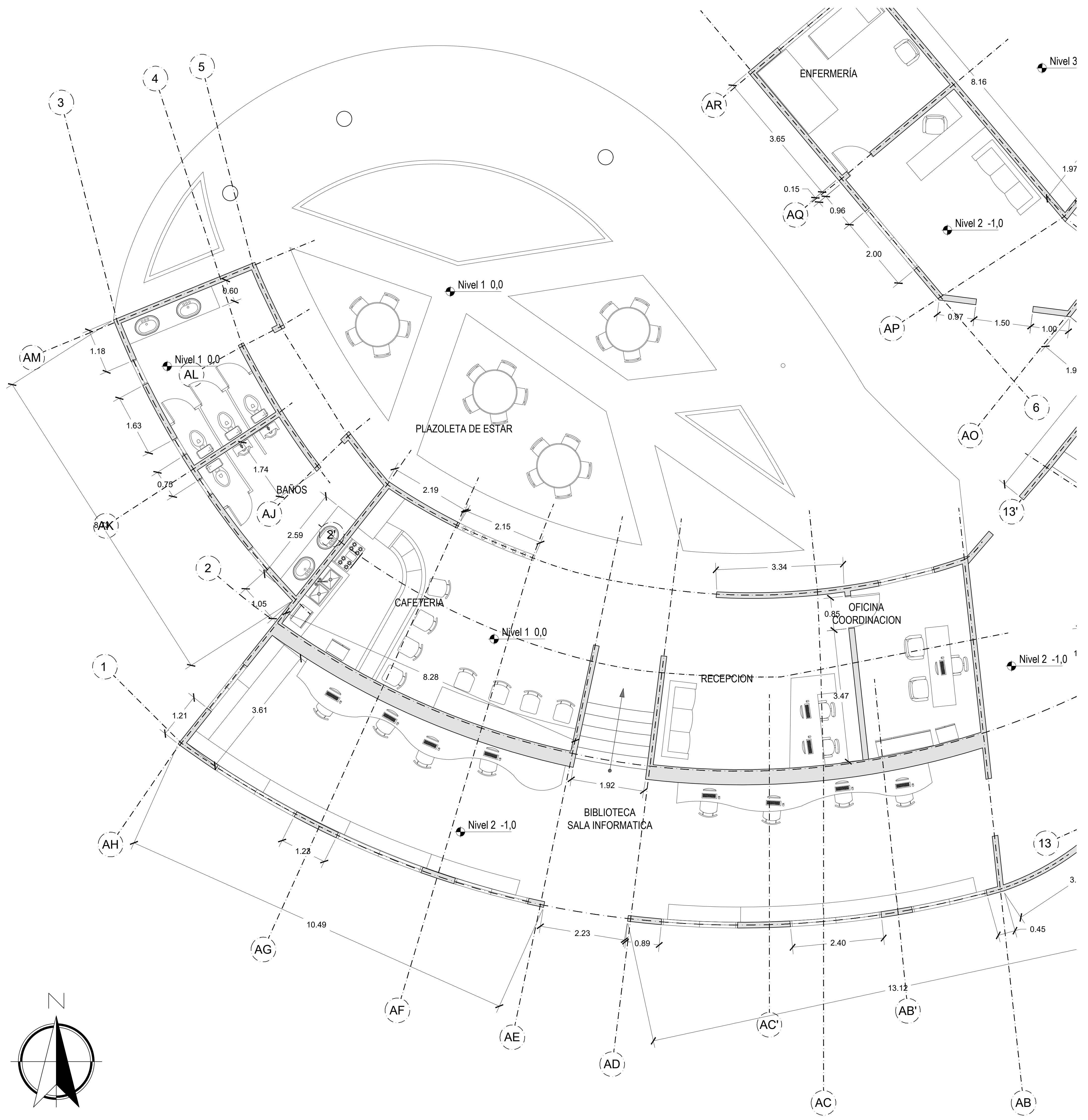
A PLANTA NIVEL 1 Esc. 1:50
