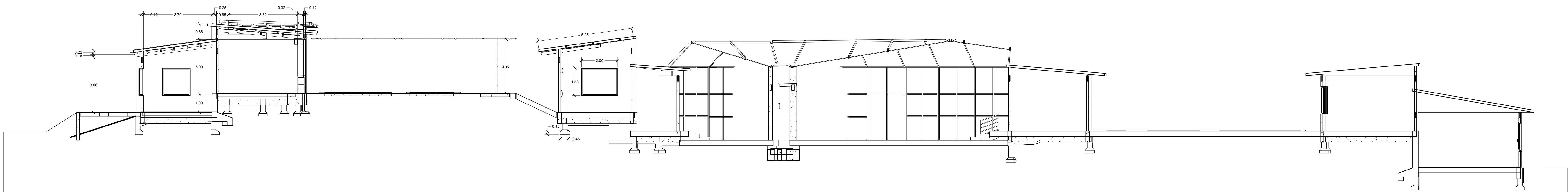
A CORTE LONGITUDINAL Esc. 1:100
