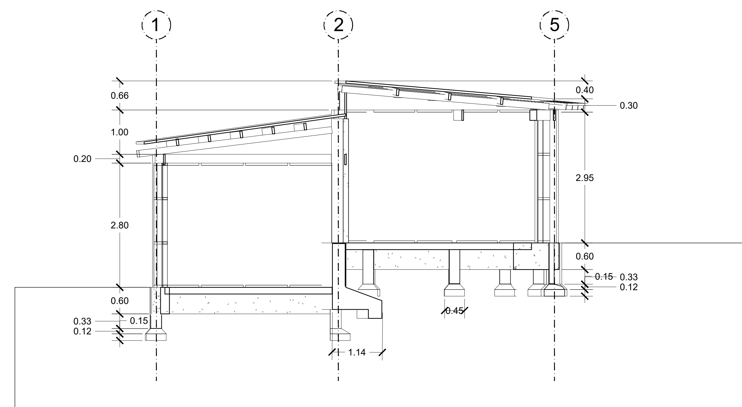
A CORTE TRANSVERSAL Esc. 1:50
