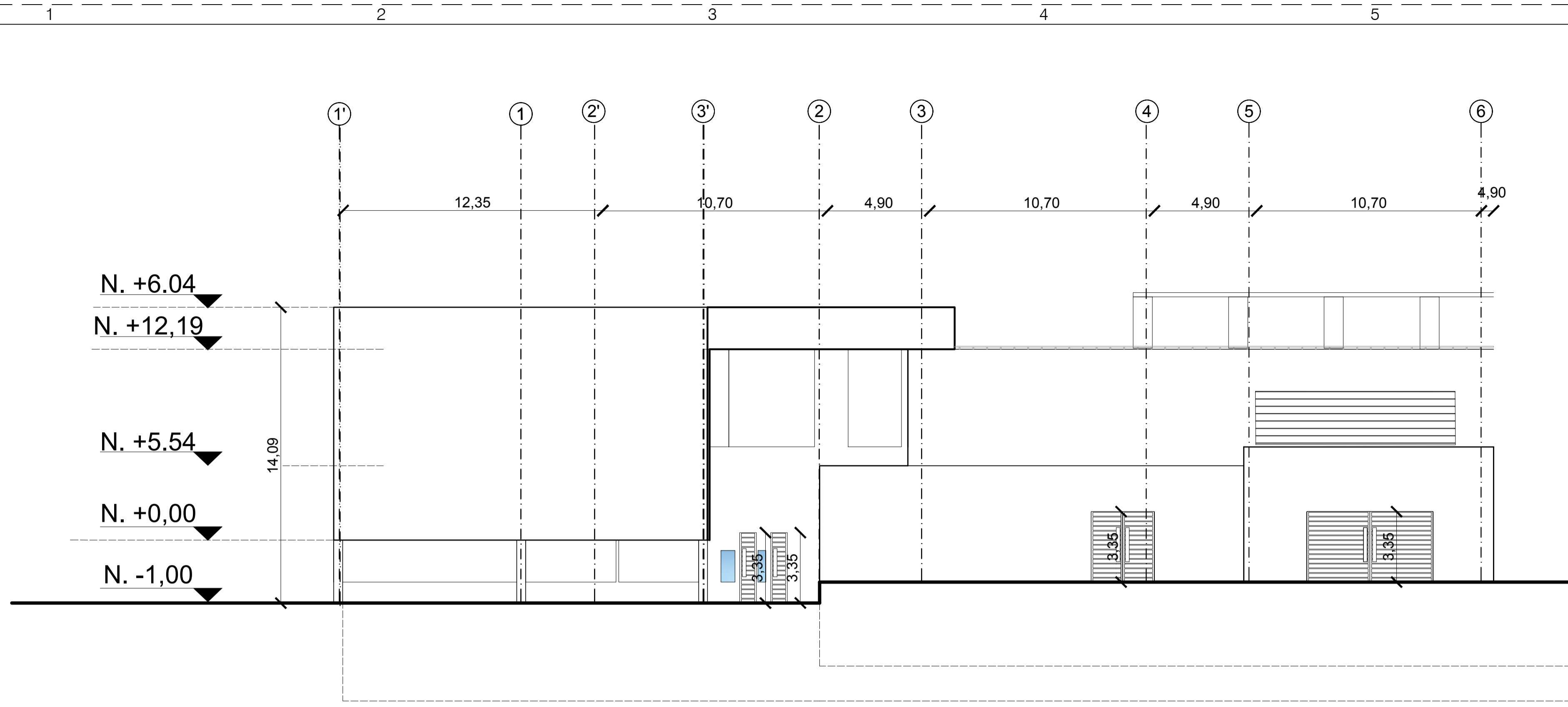
FACHADA SUR Esc 1:250
