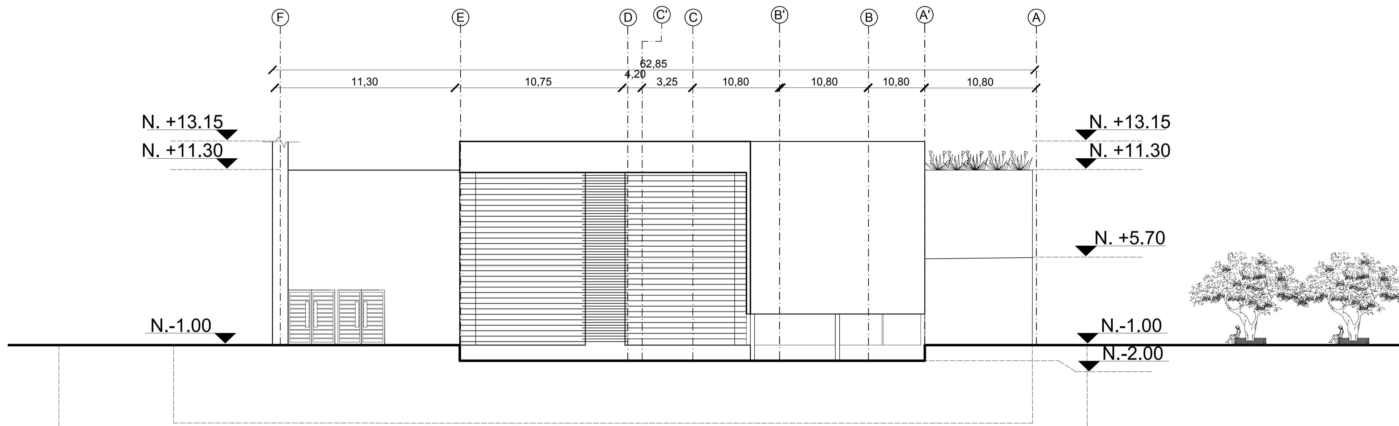
FACHADA ORIENTE Esc 1:150
