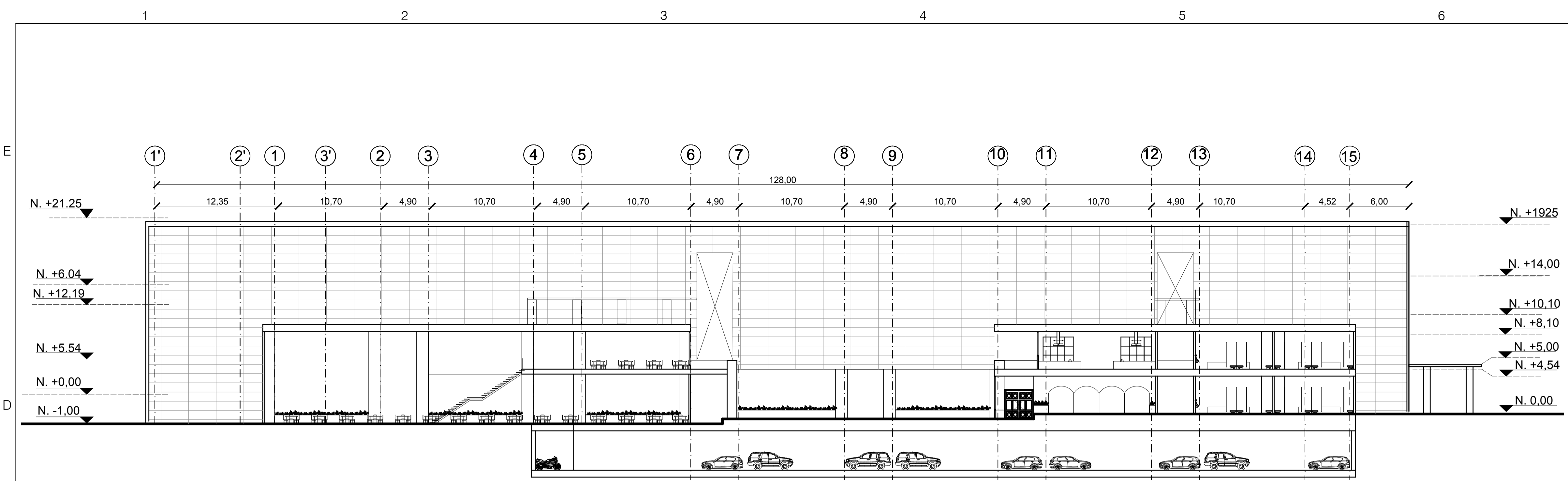
CORTE C-C Esc. 1:250
