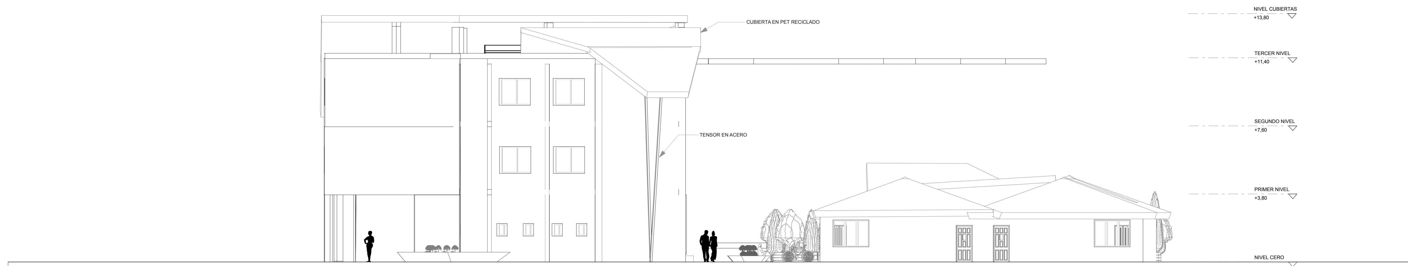
F HOGAR TERAPEUTICO Y COMEDOR FACHADA 01 ESC: 1:125
