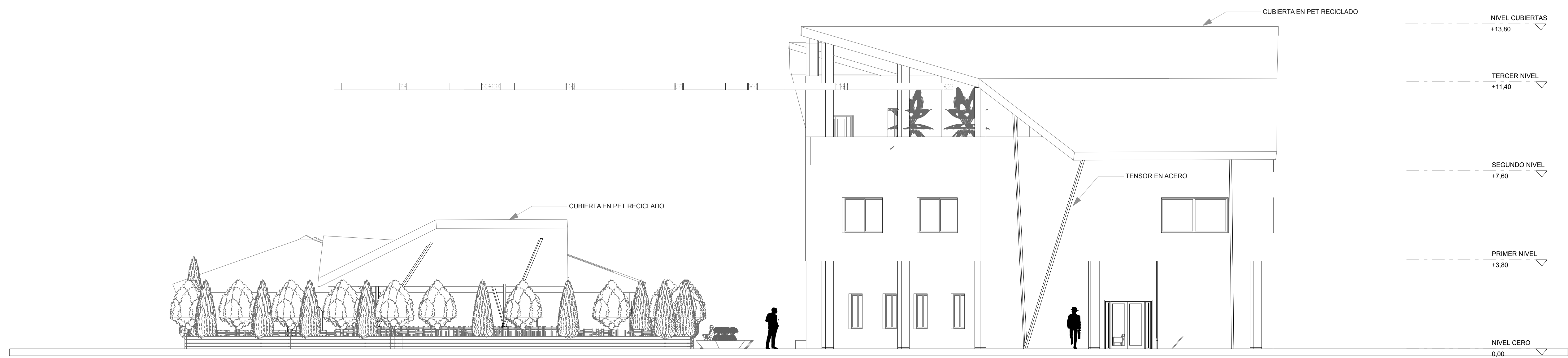
F HOGAR TERAPEUTICO Y COMEDOR FACHADA 02 ESC: 1:125
