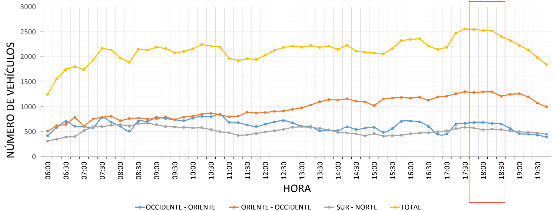
HORA VS NÚMERO DE VEHÍCULOS POR CADA ACCESO DIA 18 DE AGOSTO DE 2016
