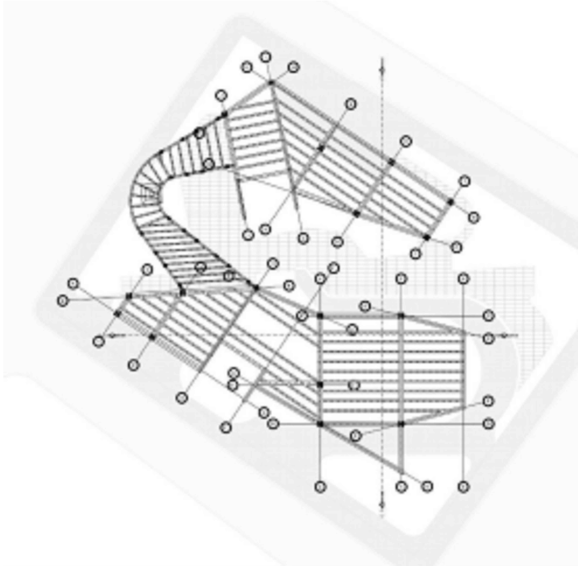
PLANTA ESTRUCTURAL PISO 2
