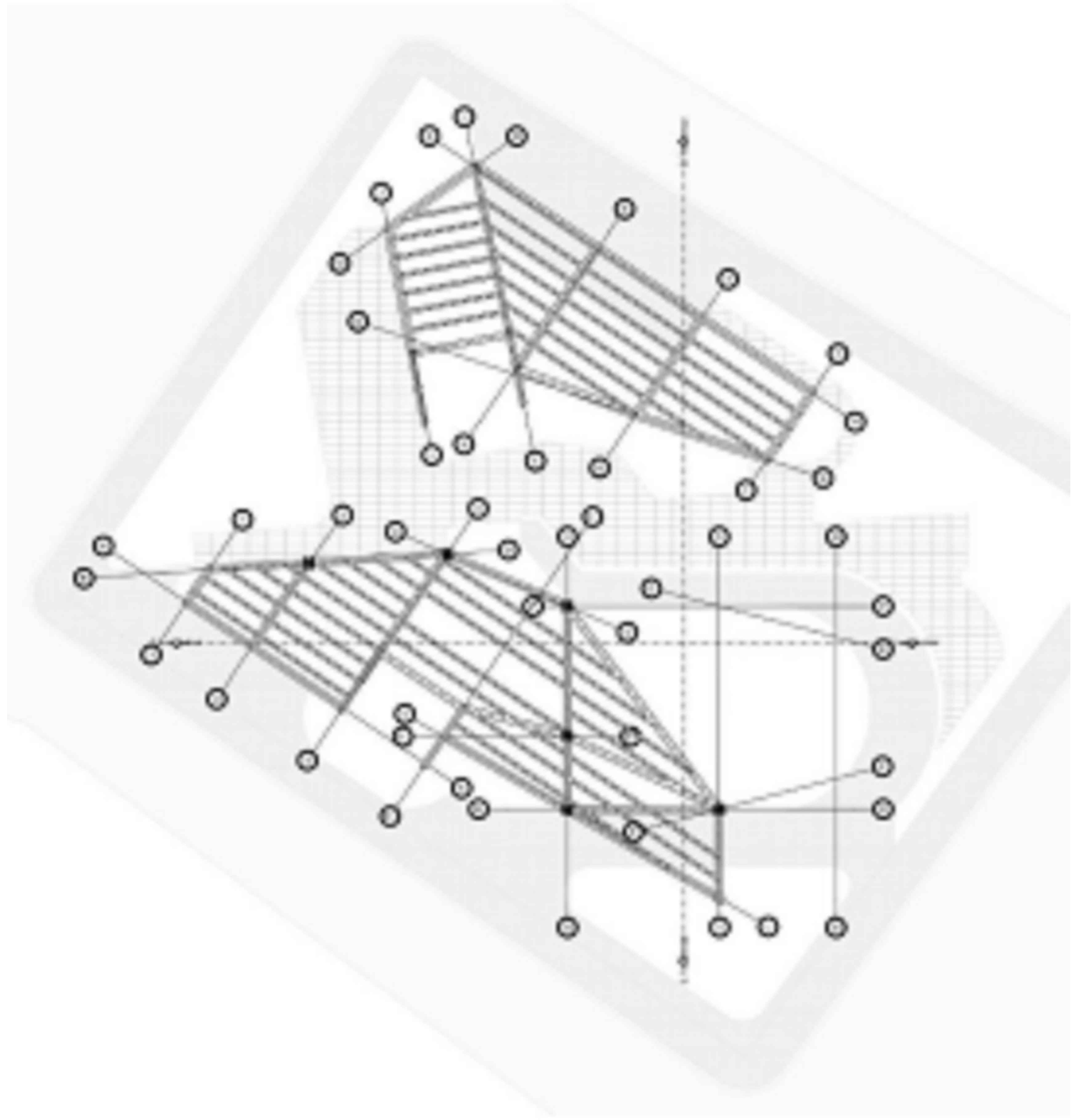
PLANTA ESTRUCTURAL PISO 4
