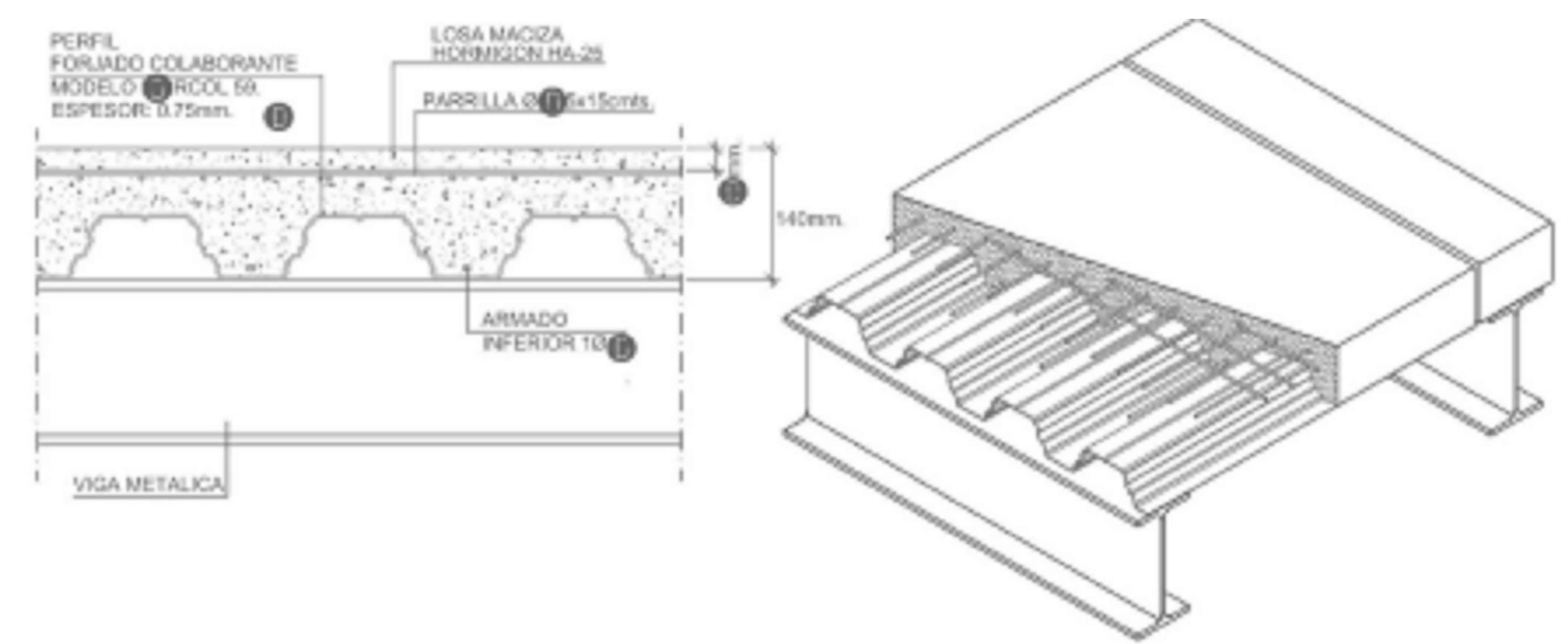
DETALLE CONSTRUCTIVO ENTRE PISO ESCALA 1:200
