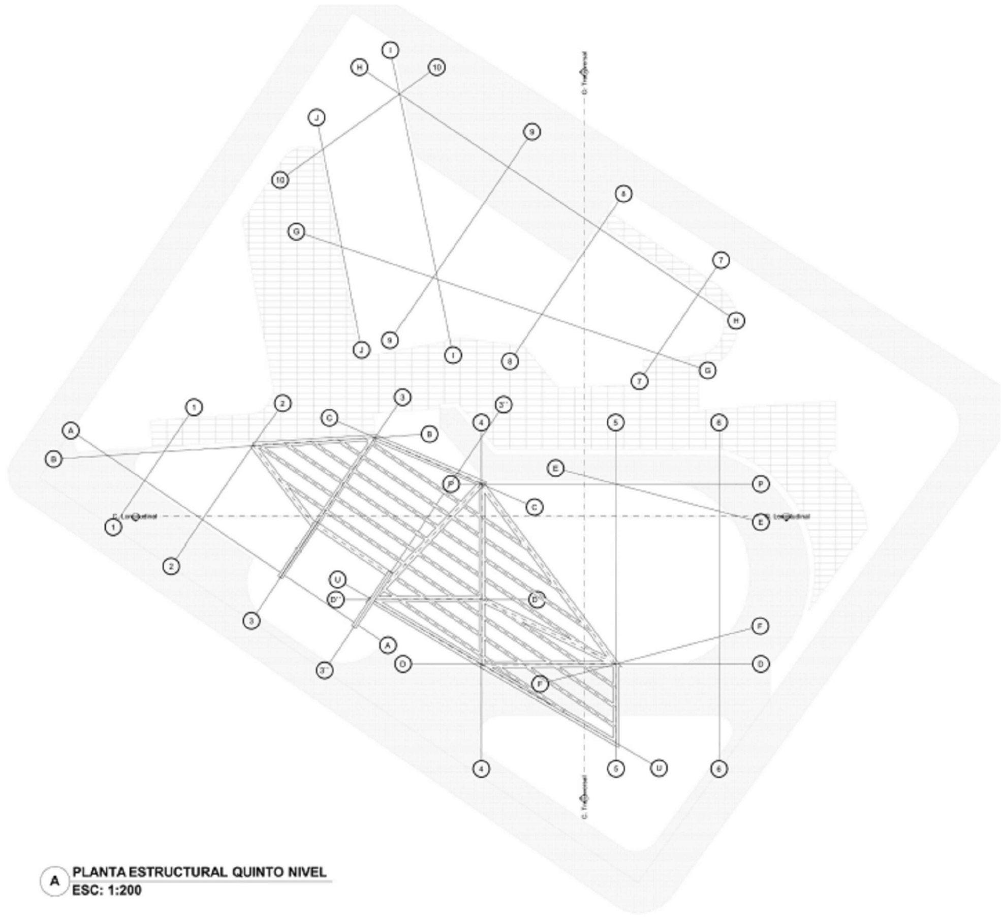
PLANTA ESTRUCTURAL PISO 5
