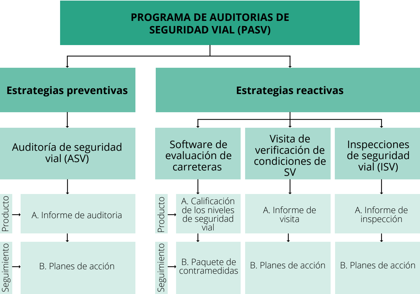
Figura 2. Programa de auditorías de seguridad vial
