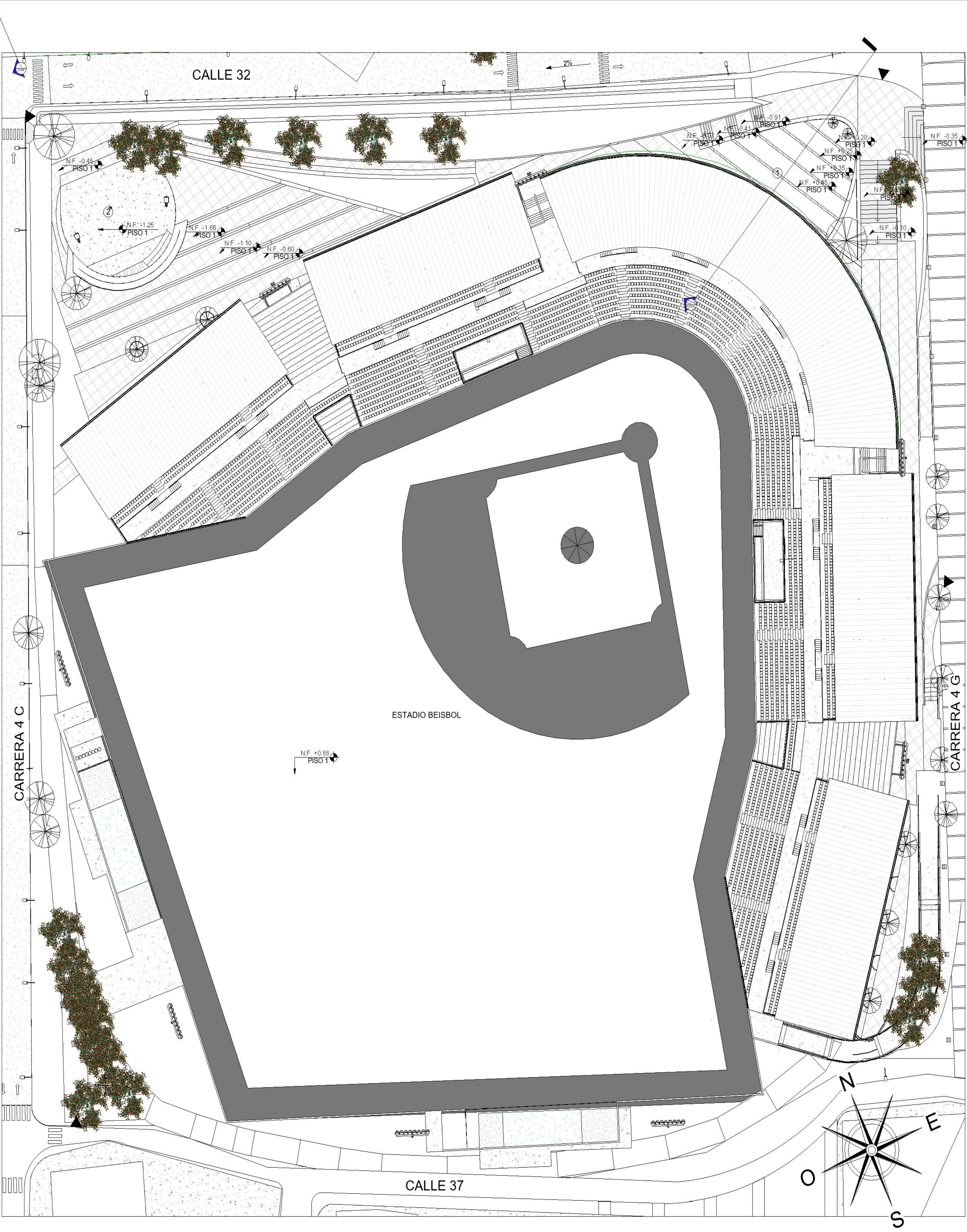
1 Planta plan parcial unidad 1 1 : 300
