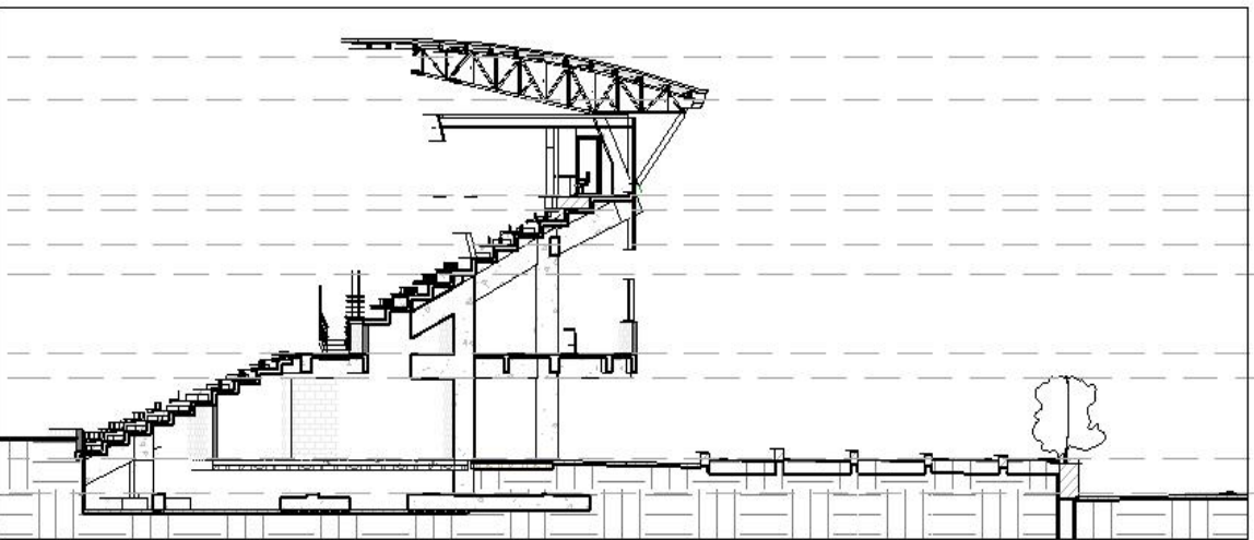
2 corte unidad 1 1 : 300
