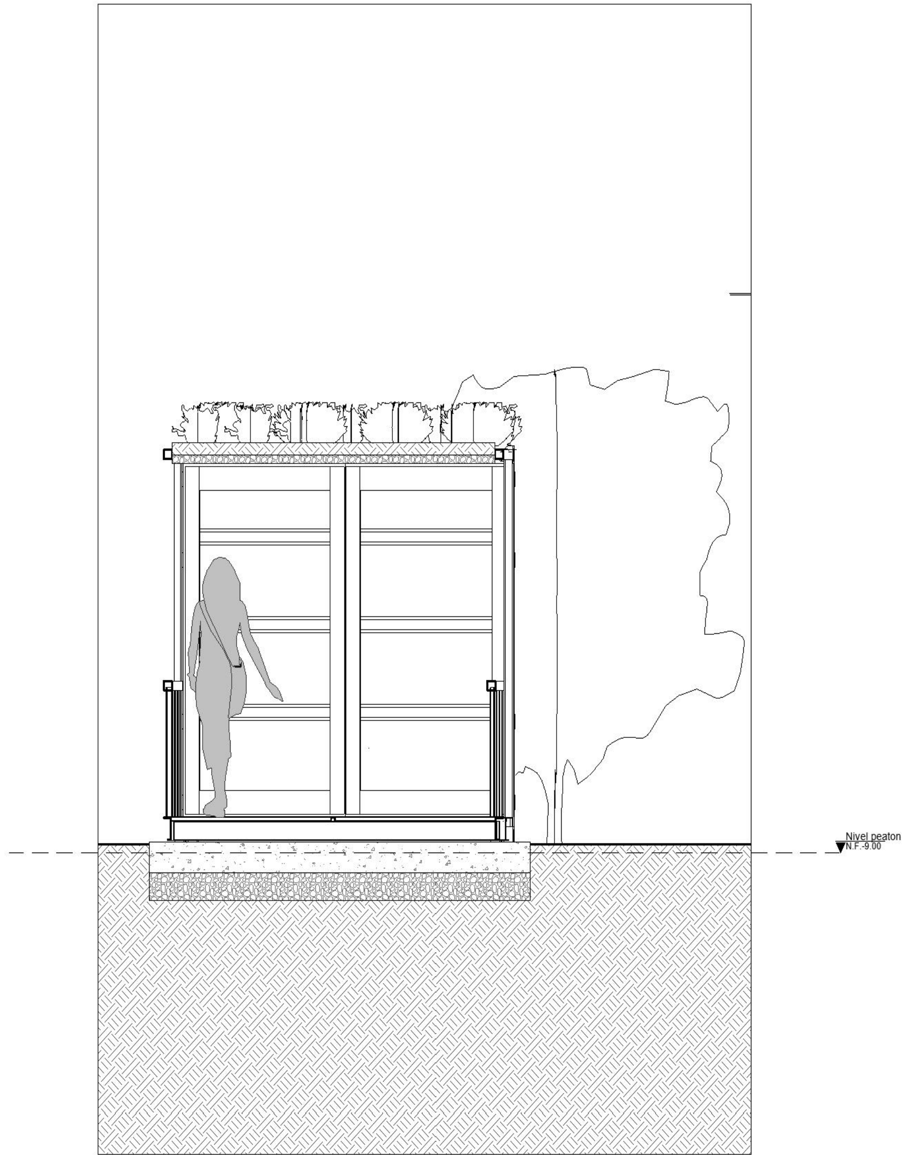
1 Detalle casetas 1 : 25
