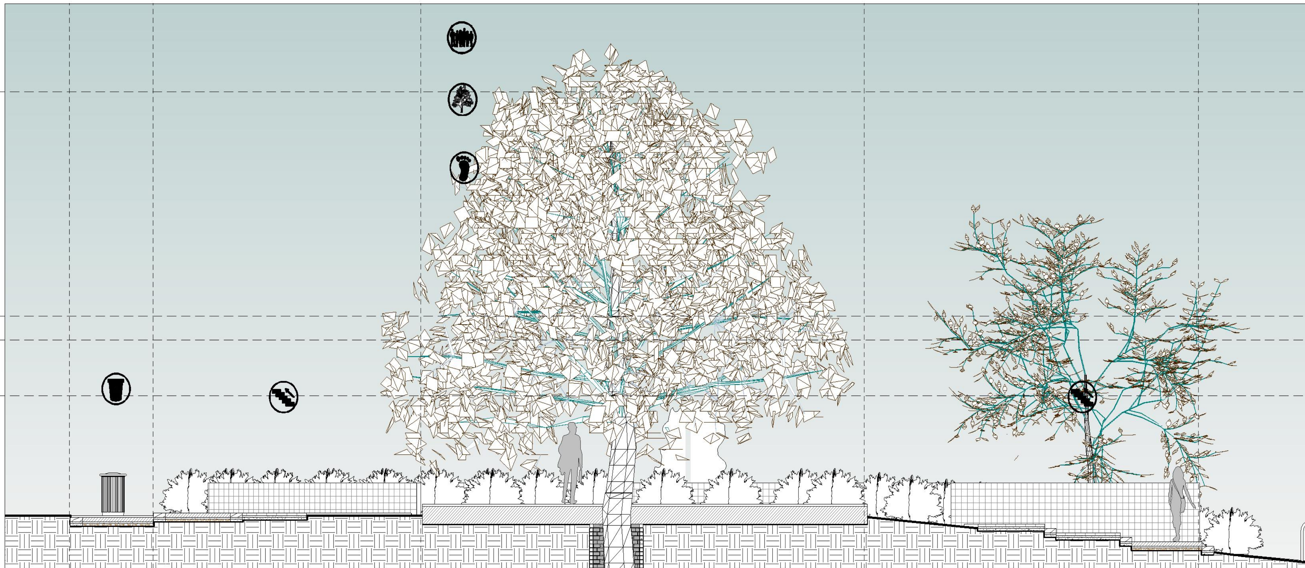
3 Corte Detalle Plazoleta Arbol 1 : 50
