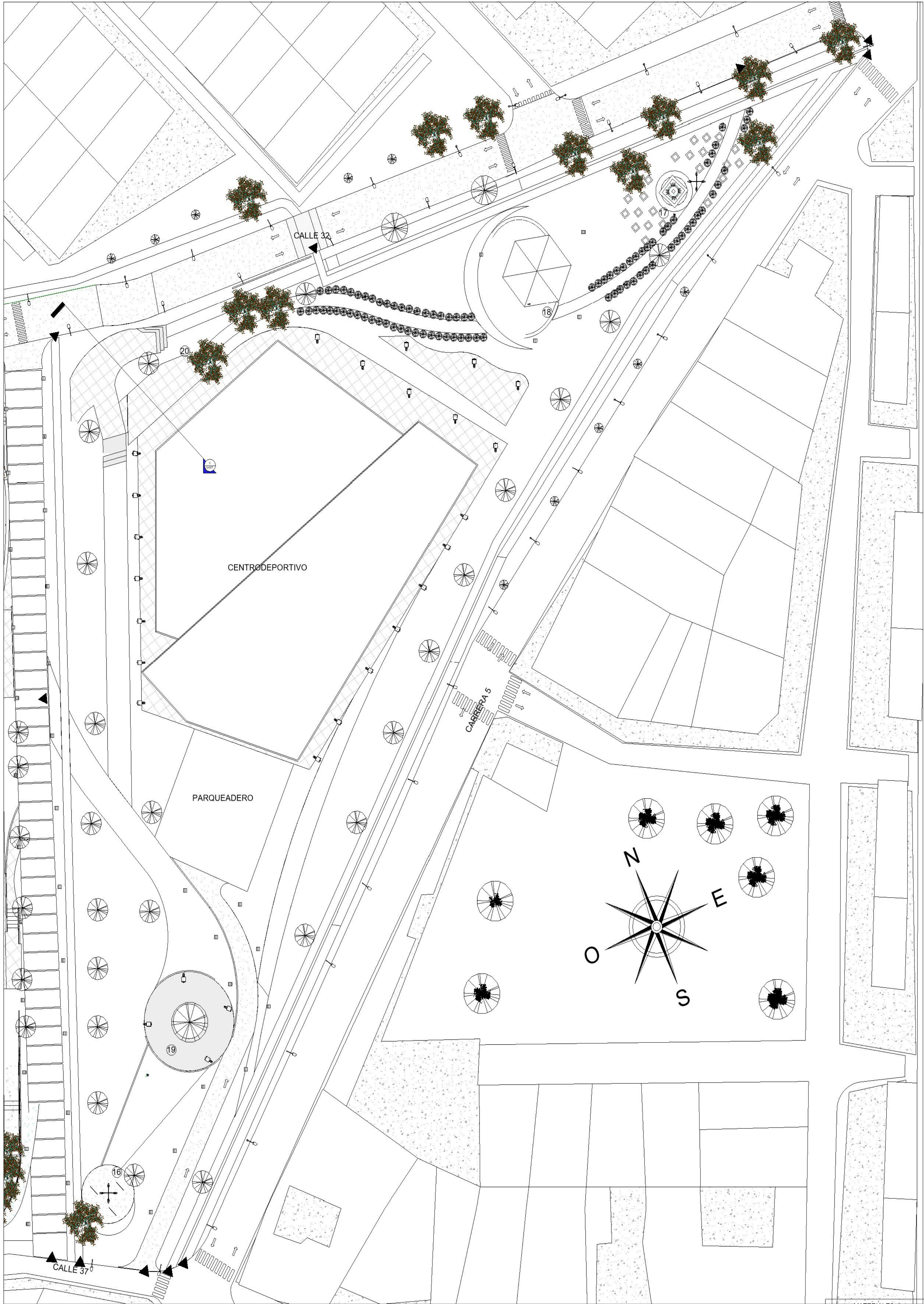
1 Planta plan parcial unidad 3 1 : 350
