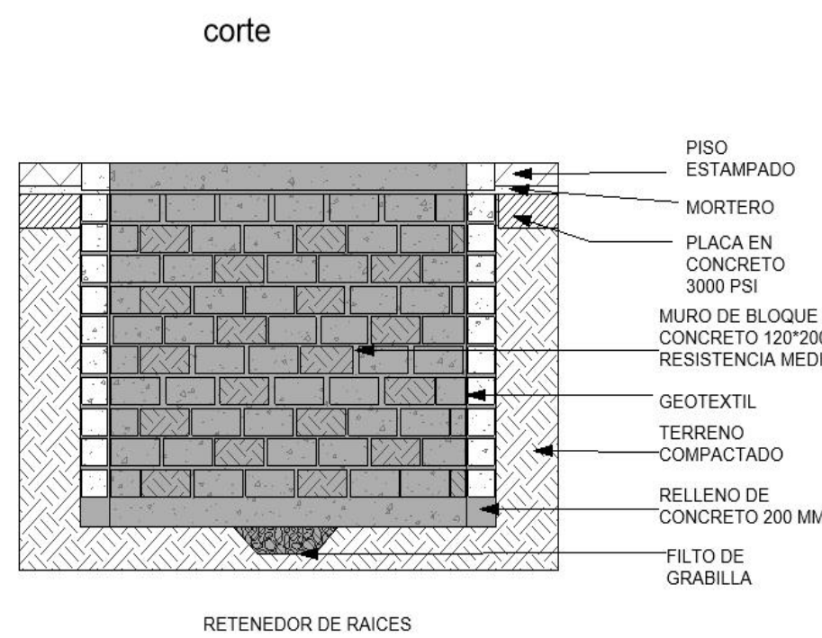
Contenedor de raices 1 : 20
