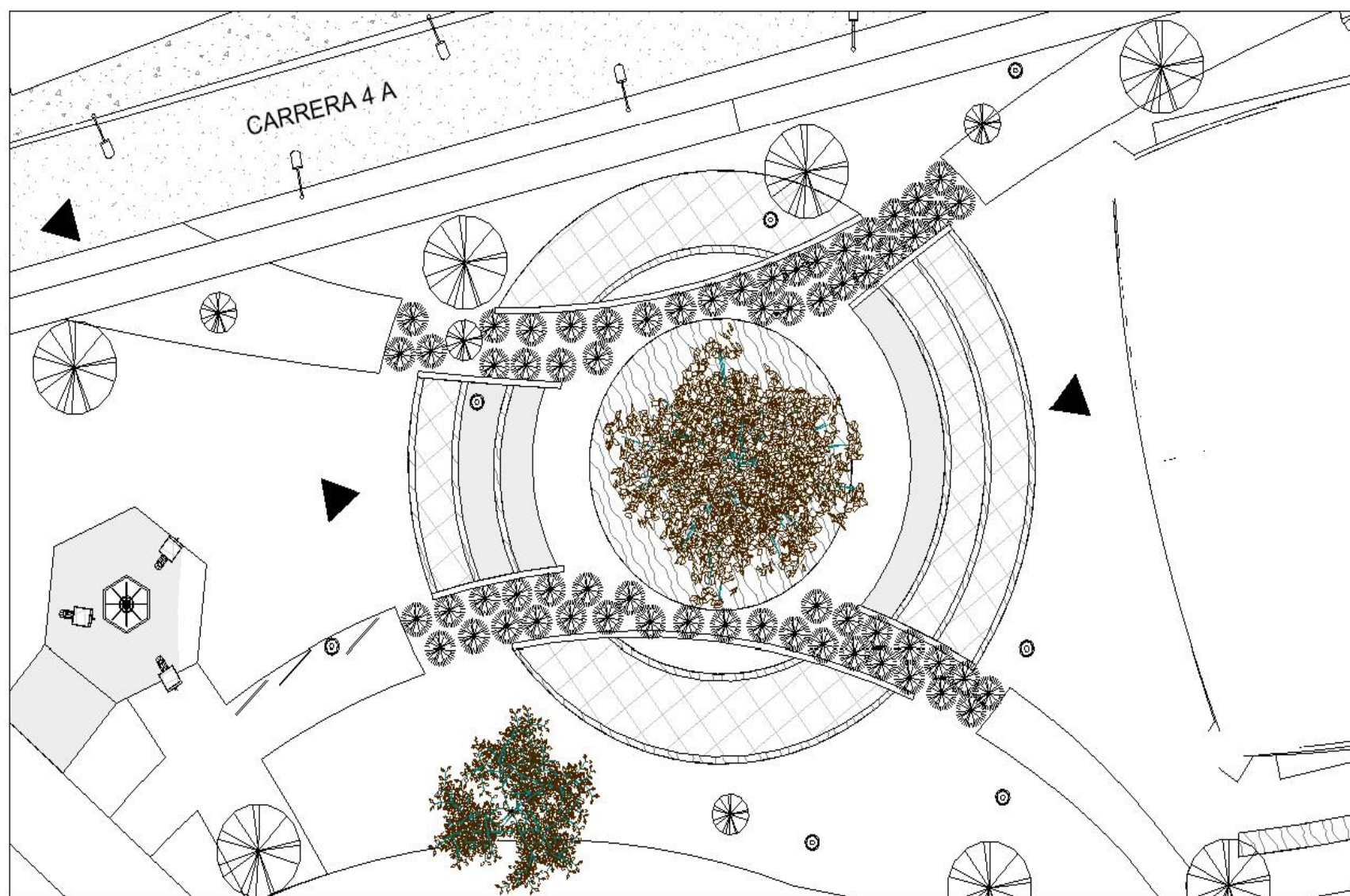
4 Planta plan parcial unidad 5 plaza arbol 1 : 250
