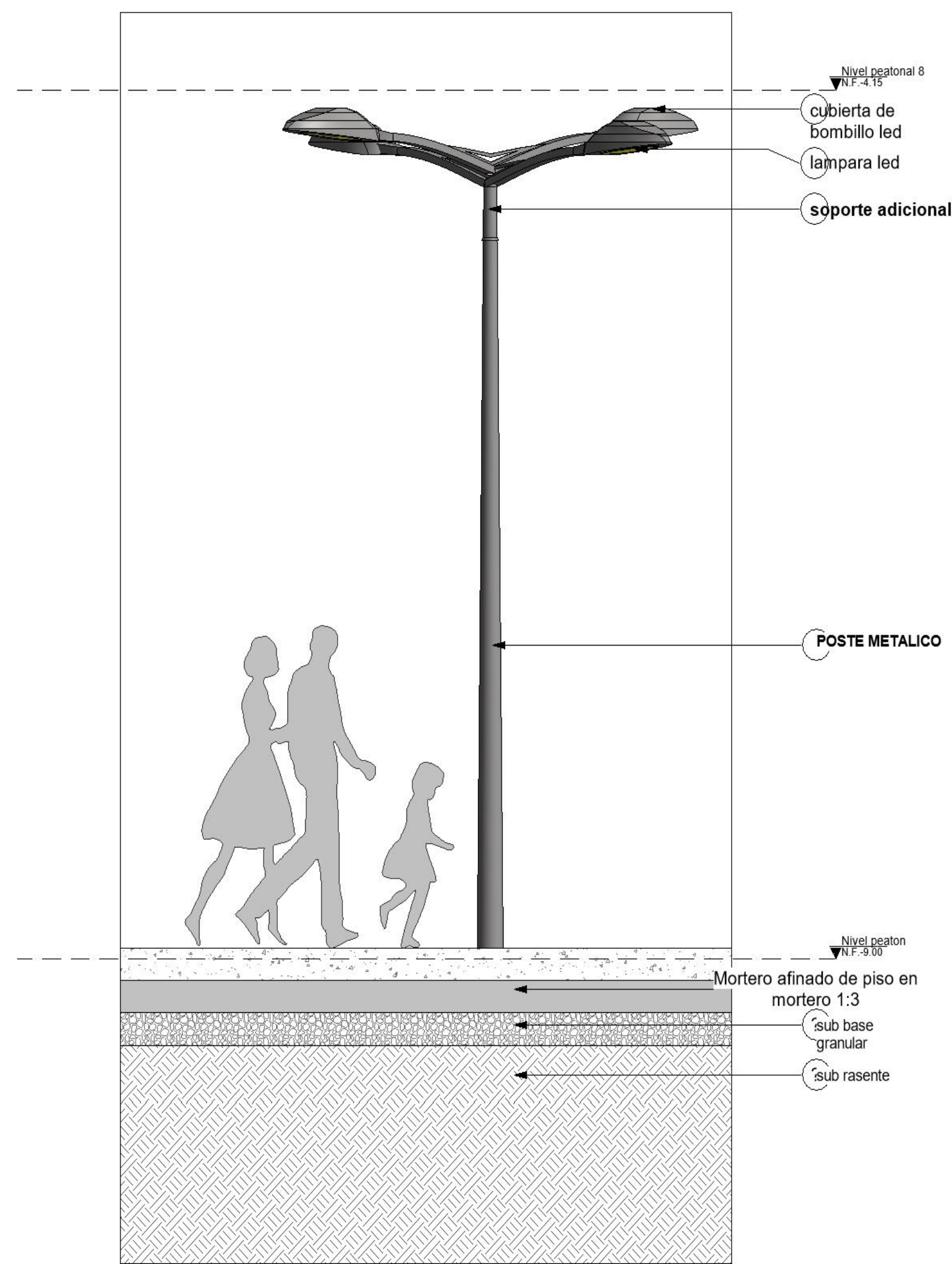
2 CORTE DETALLE PLAZOLETA 1 : 25
