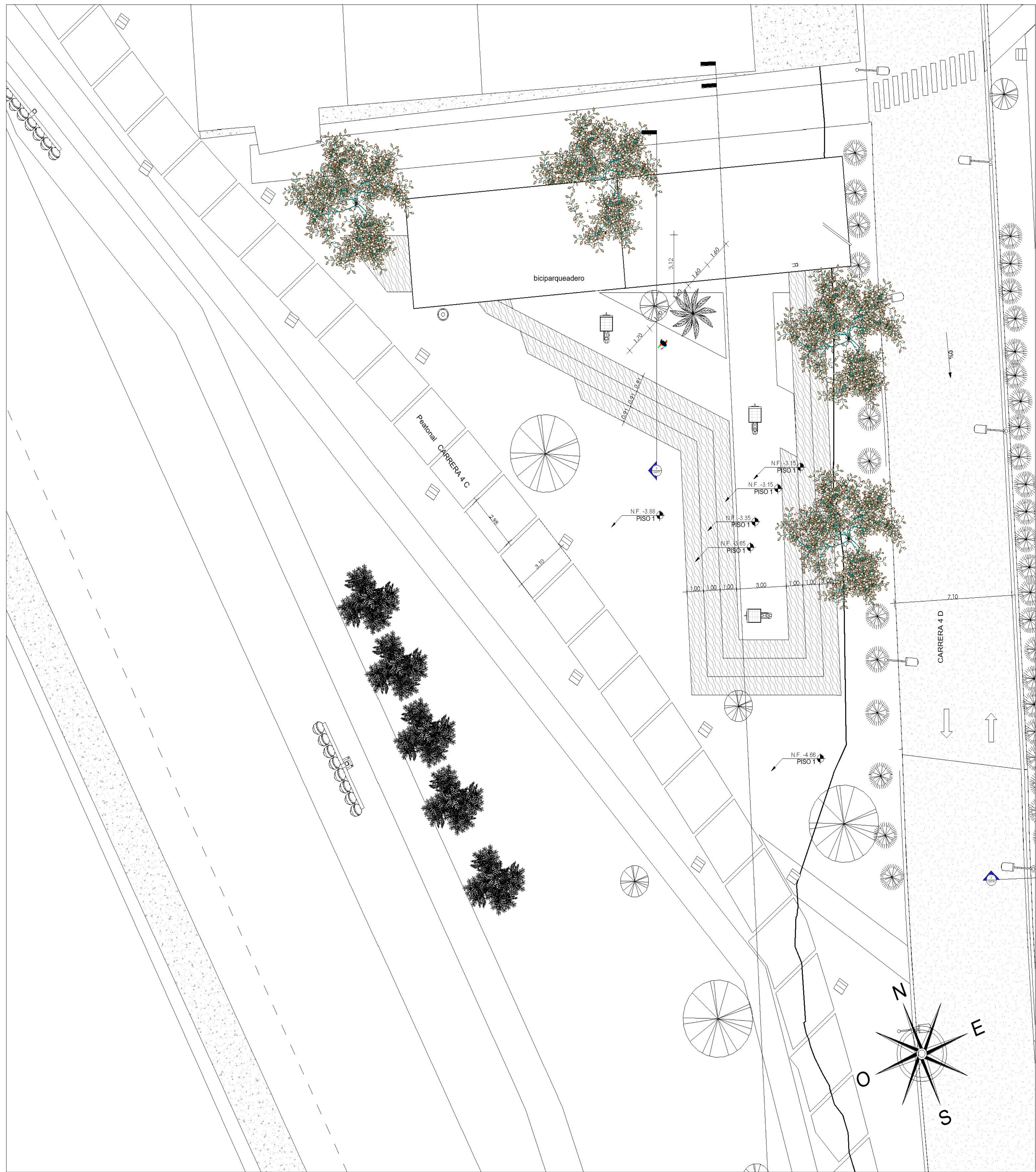
1 Planta detalle biciparqueo unidad 2 1 : 100
