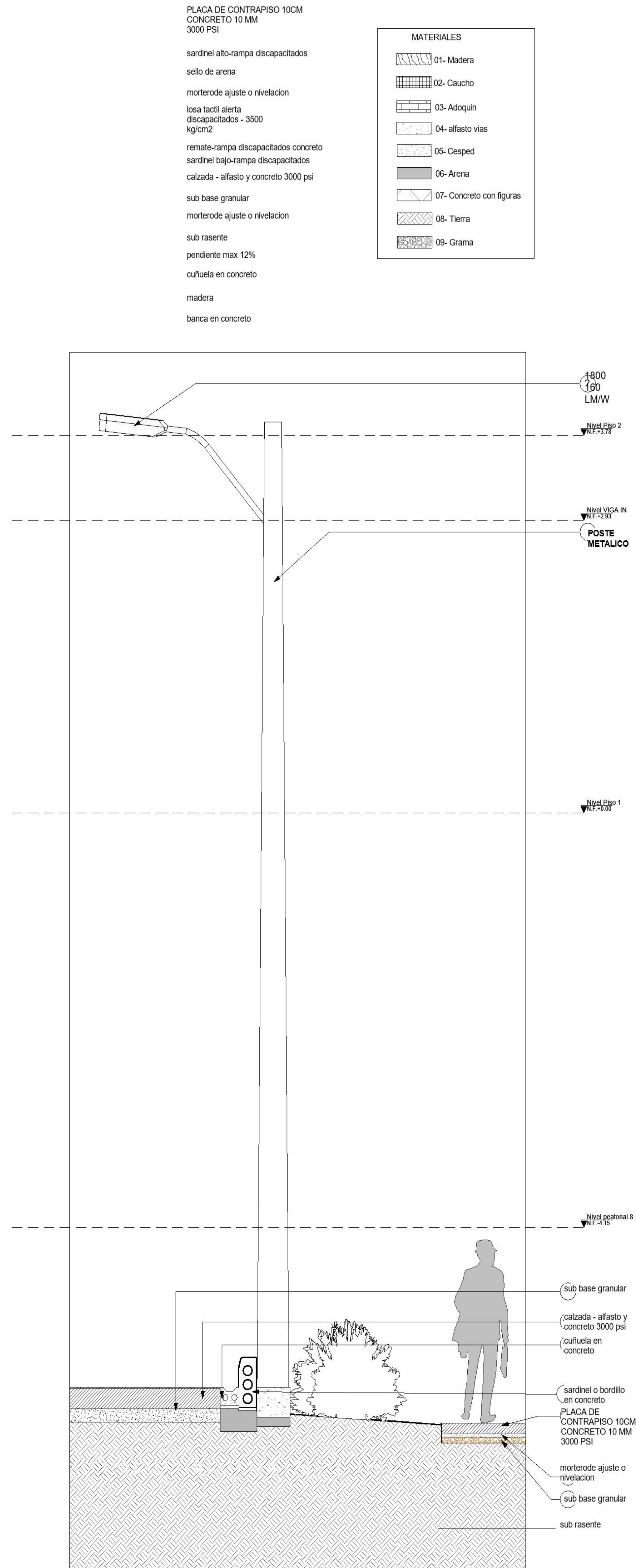
3 iluminacion vial 1 : 25
