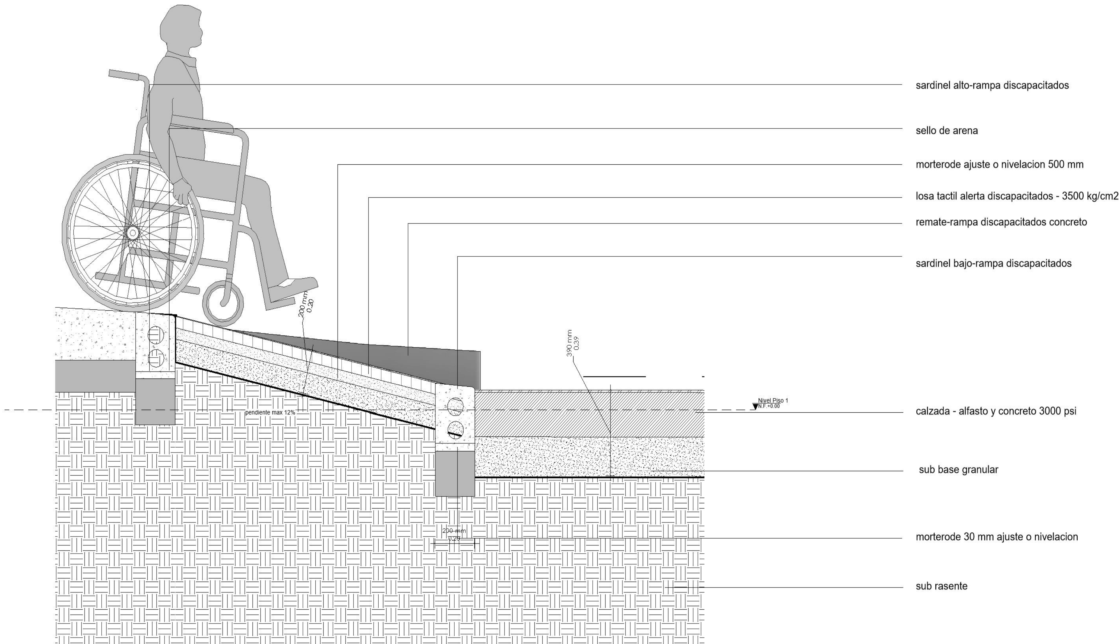
3 detalle desnivel anden 1 : 10
