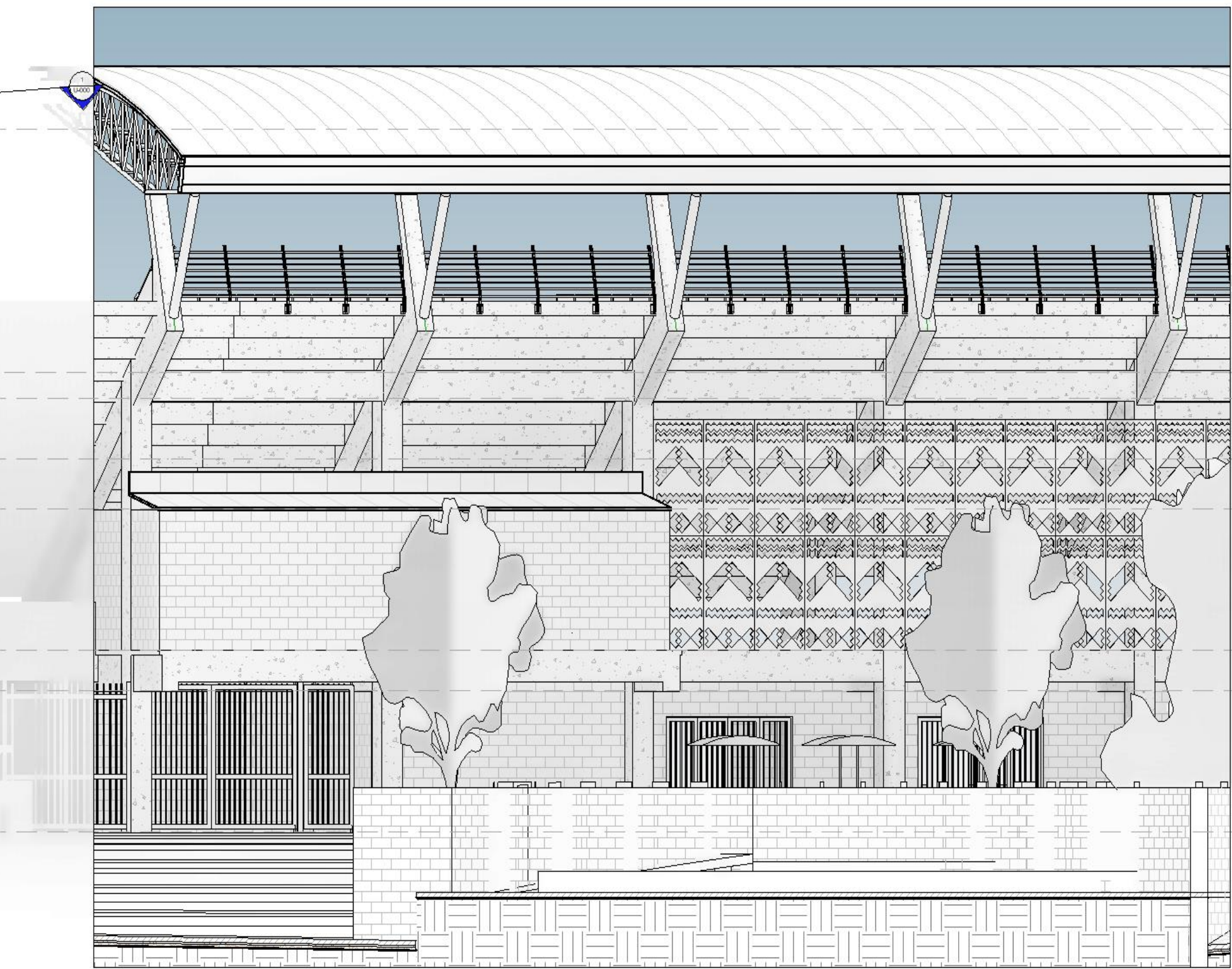
2 CORTE DE PLAZOLETA jorge alfaro 1 : 100
