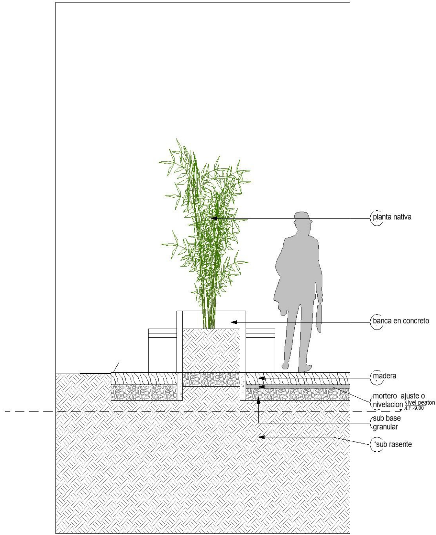
2 Detalle matera 1 : 25
