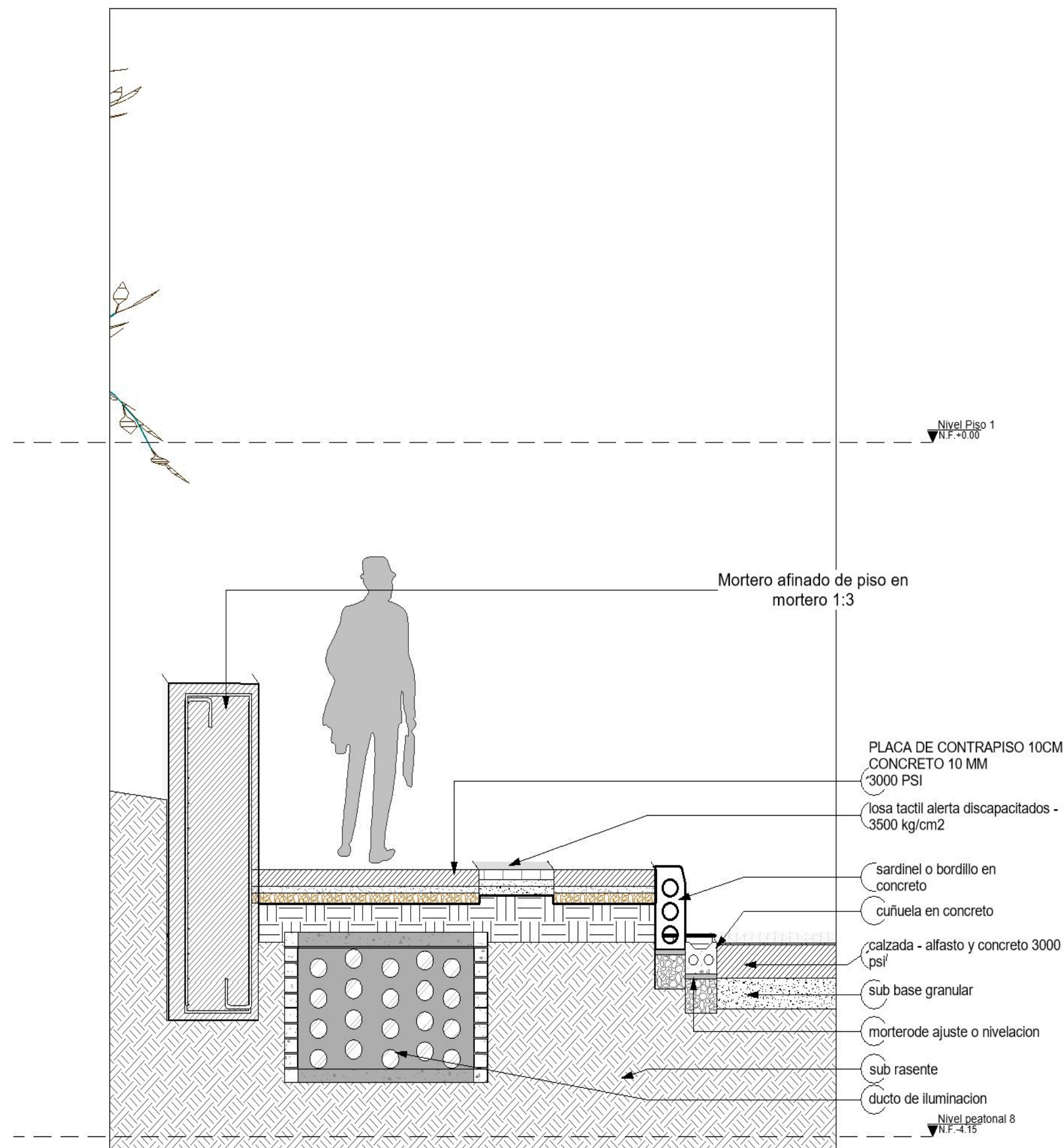
5 anden para videntes 1 : 25
