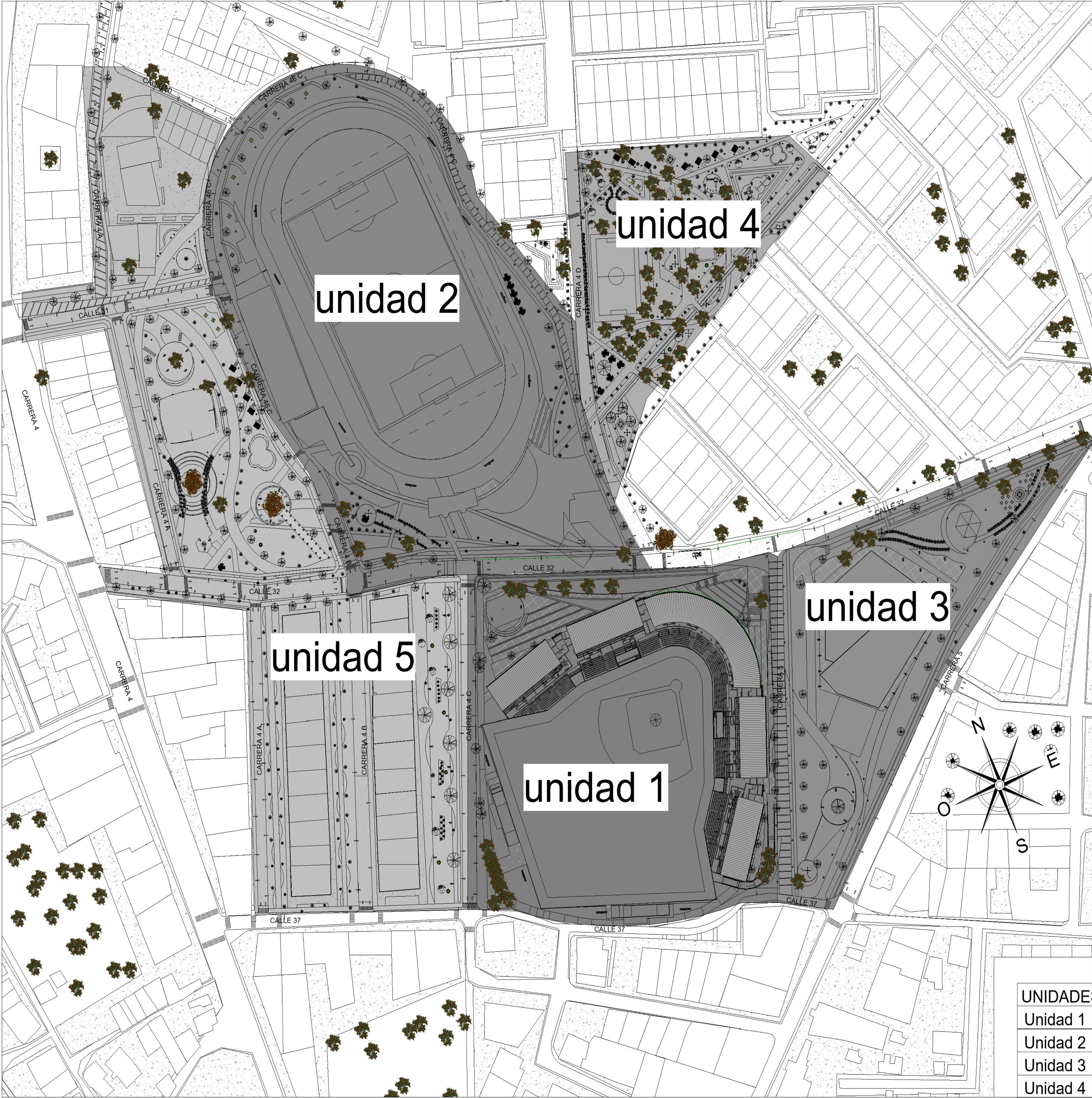
1 Planta plan parcial 1 : 800
