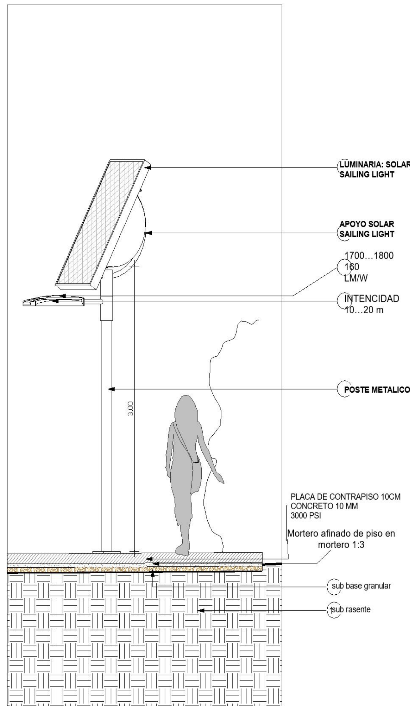
4 iluminacion plazoletas 1 : 25
