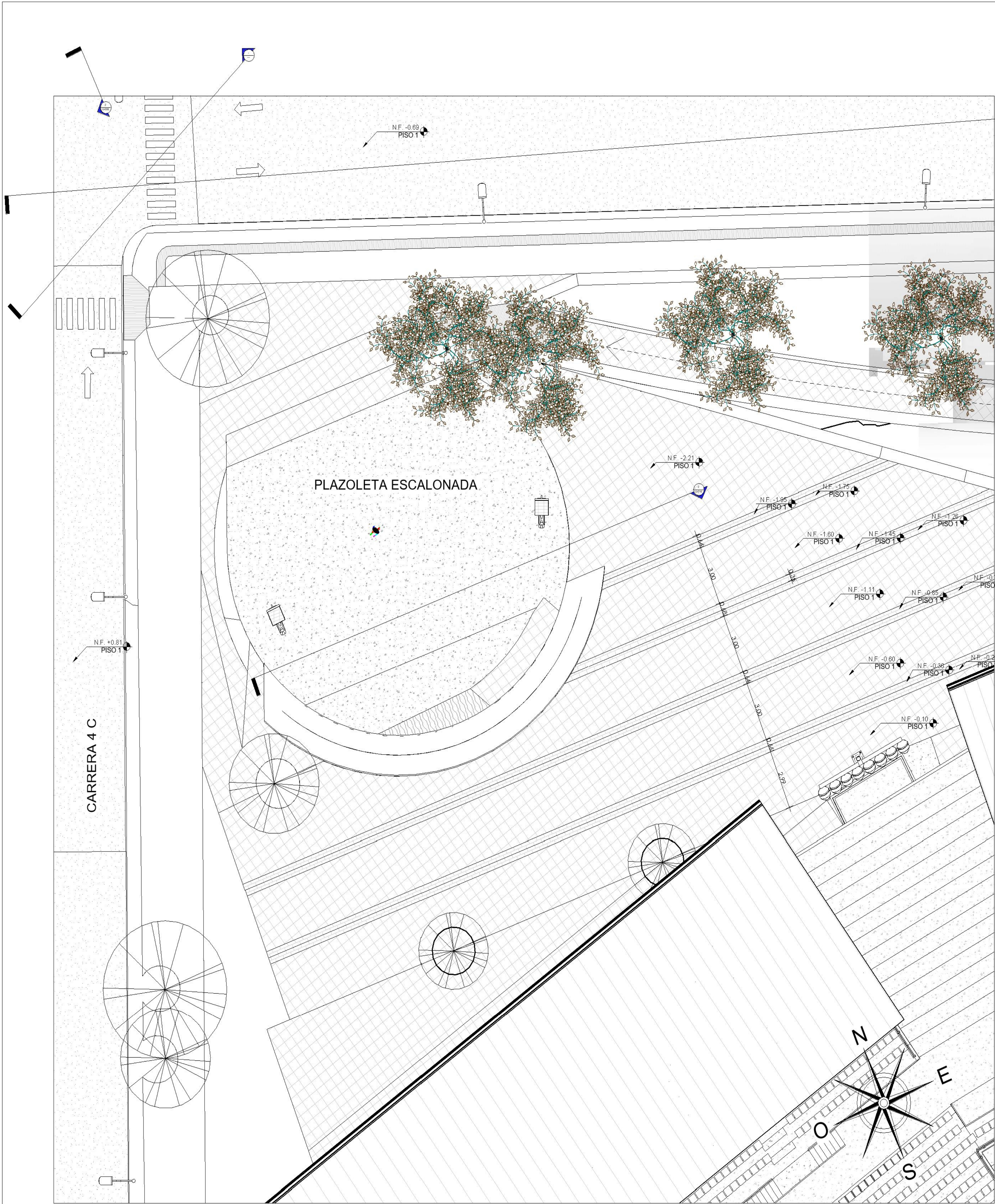
1 Planta detalle plazoleta jorge alfaro unidad 1 1 : 100
