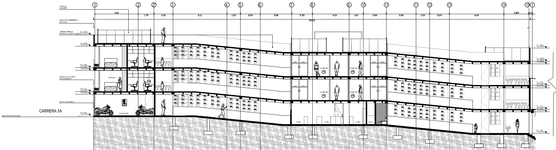
P16 CORTE 2 ESCALA 1:75
