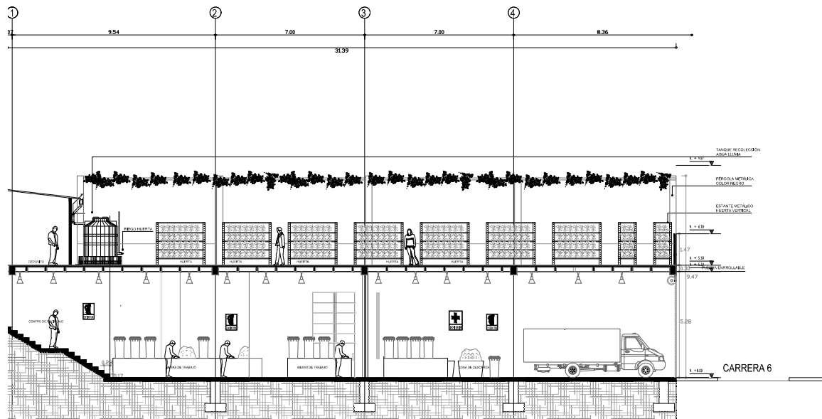
P17 CORTE 2 CONTINUACION ESCALA 1:75
