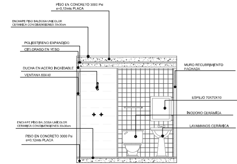
P11 DETALLE BAÑO ESCALA 1:130
