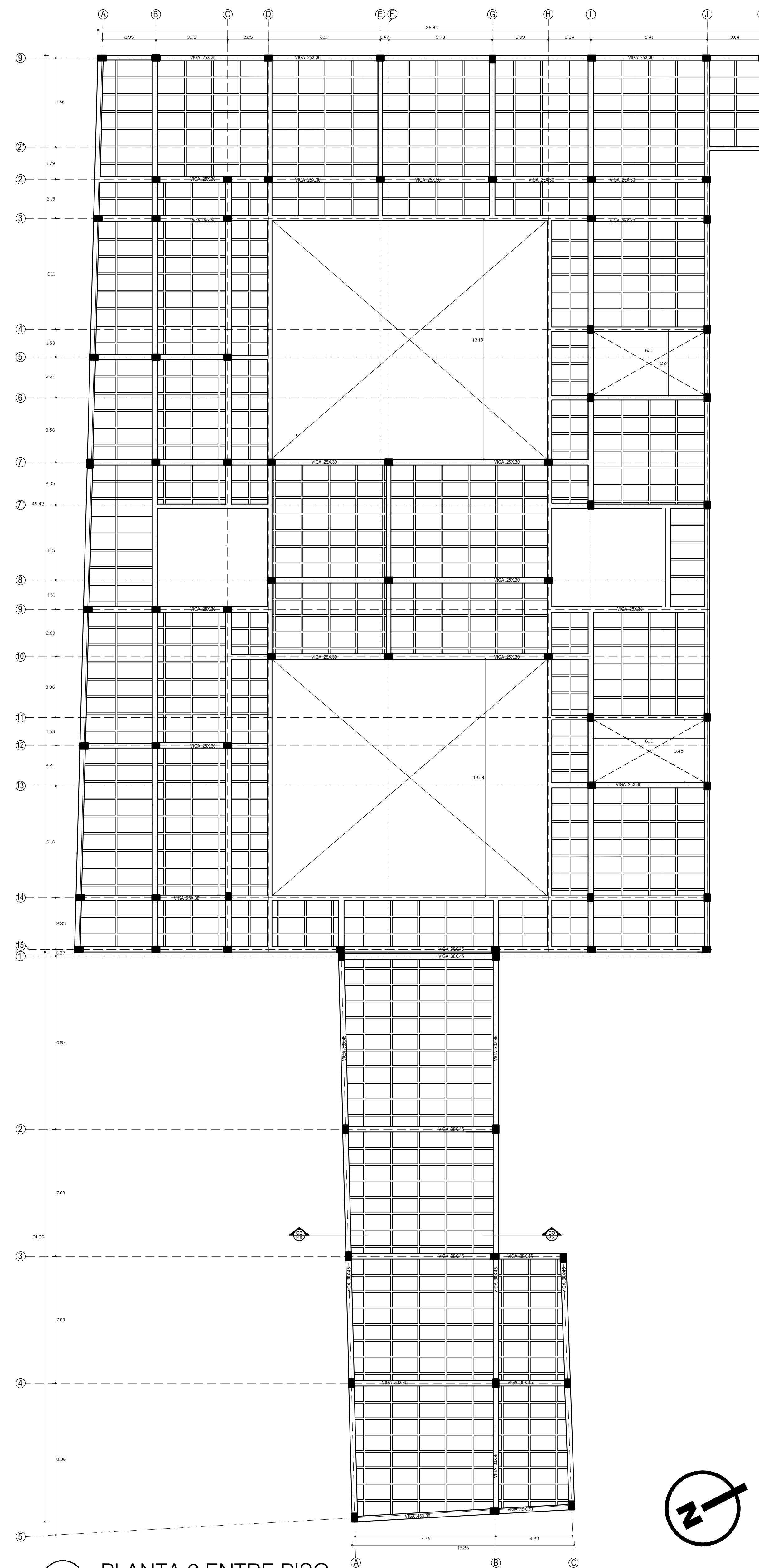
P23 PLANTA 2 ENTRE PISO ESCALA 1:150
