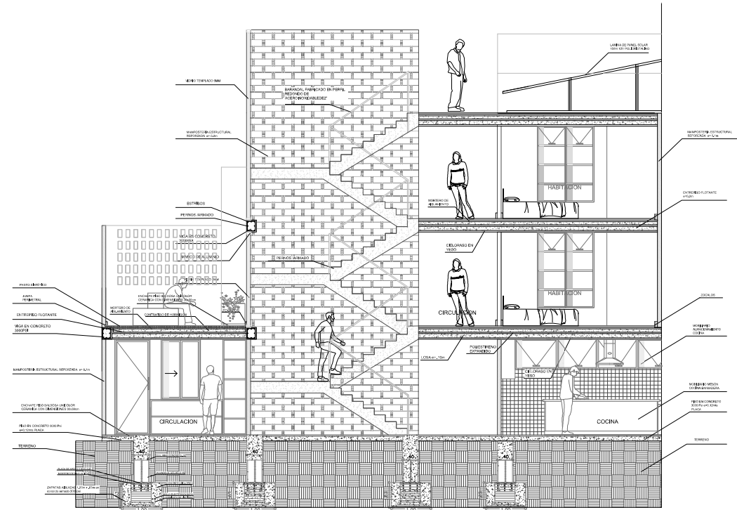
P13 CORTE FACHADA ESCALA 1:40
