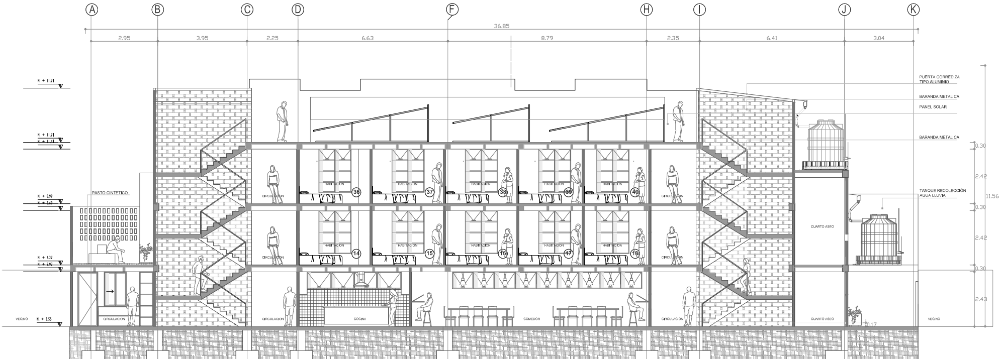
P15 CORTE 1 ESCALA 1:50
