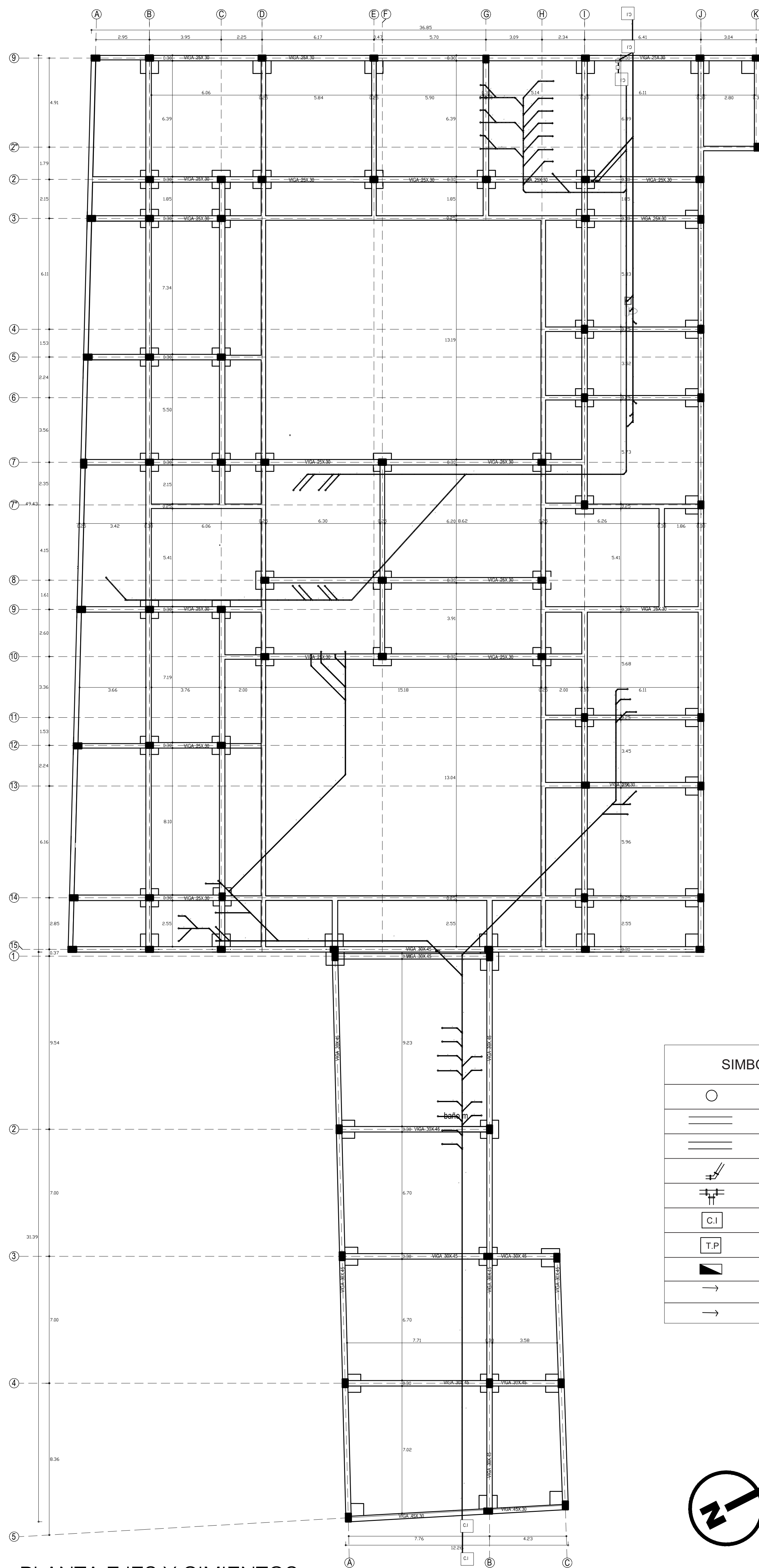
P22 PLANTA EJES Y CIMIENTOS ESCALA 1:150
