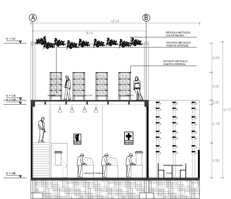
P19 CORTE 3 ESCALA 1:50
