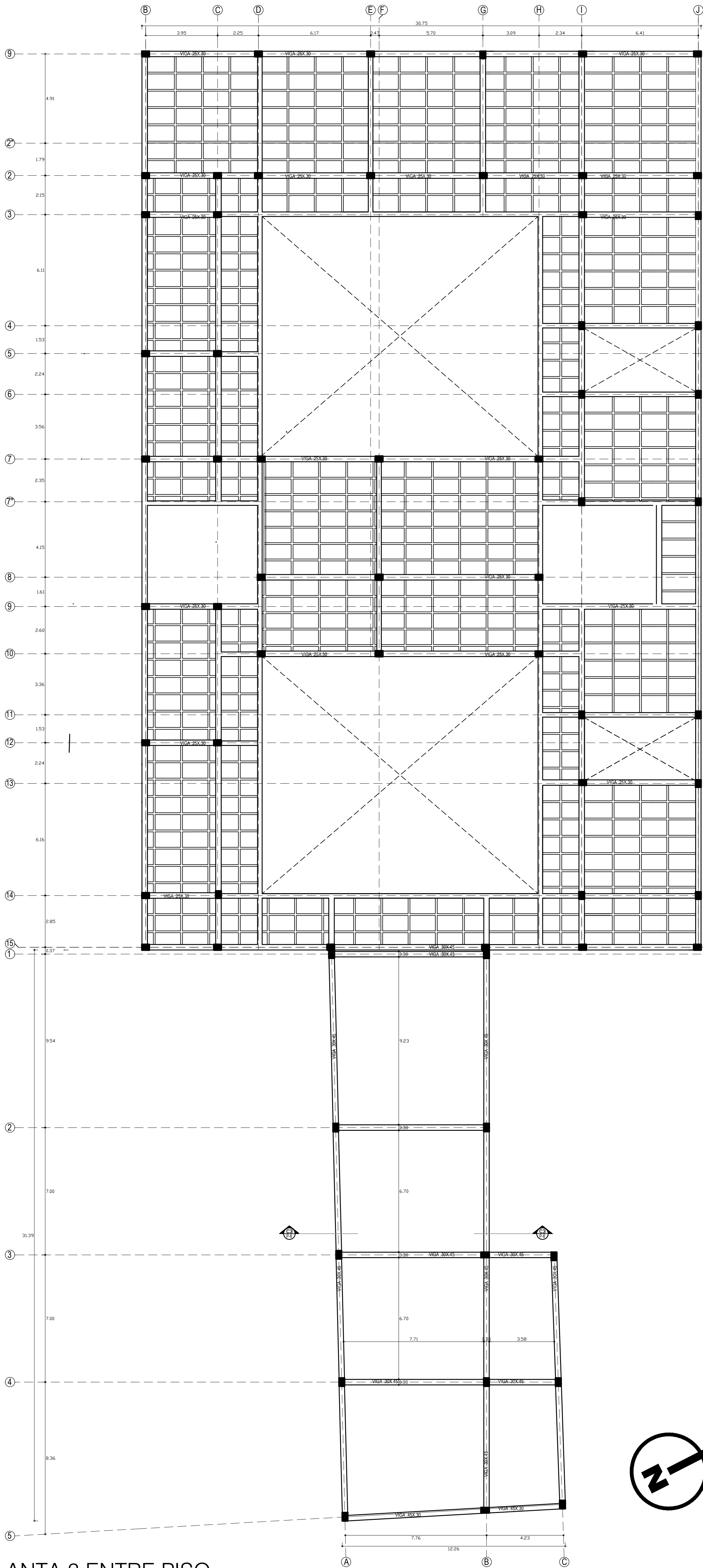
P24 PLANTA 3 ENTRE PISO ESCALA 1:150
