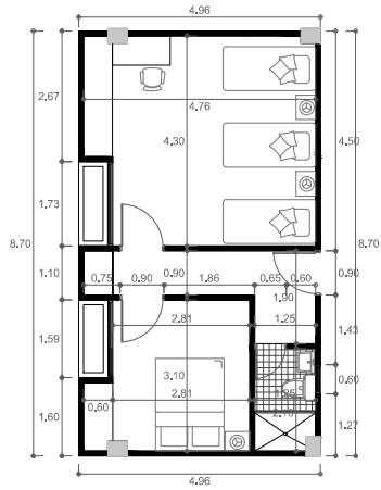
P7 PLANTA TIPOLOGIA 2 ESCALA 1:150
