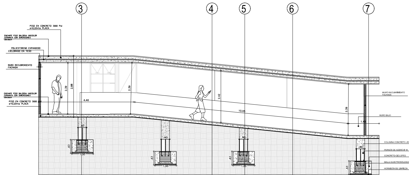
P21 DETALLE RAMPA ESCALA 1:30
