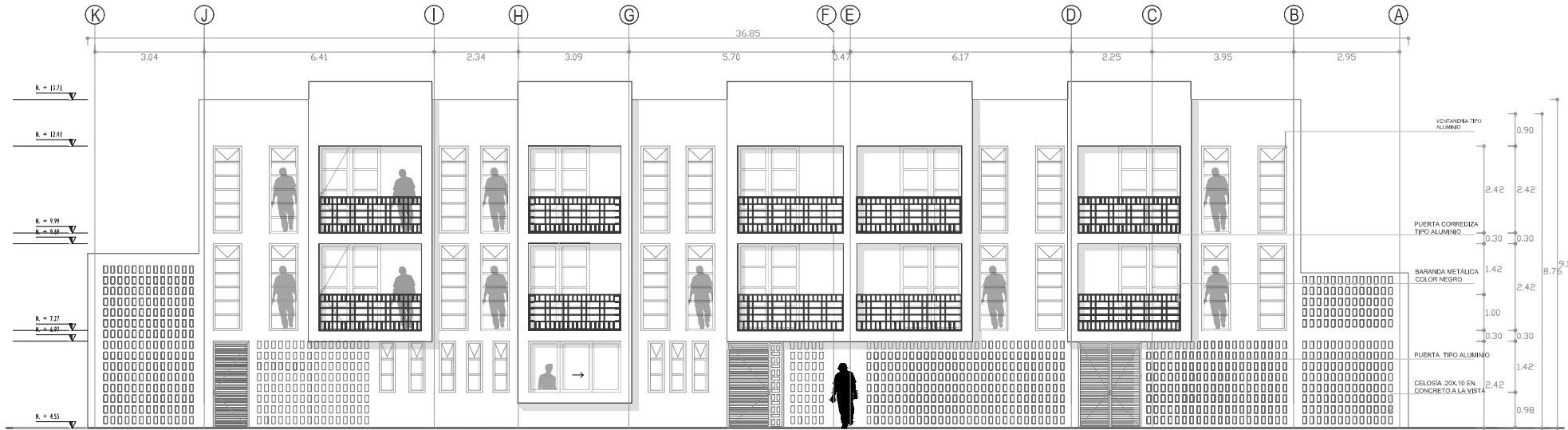
P14 FACHADA 1 CARRERA 5A ESCALA 1:50
