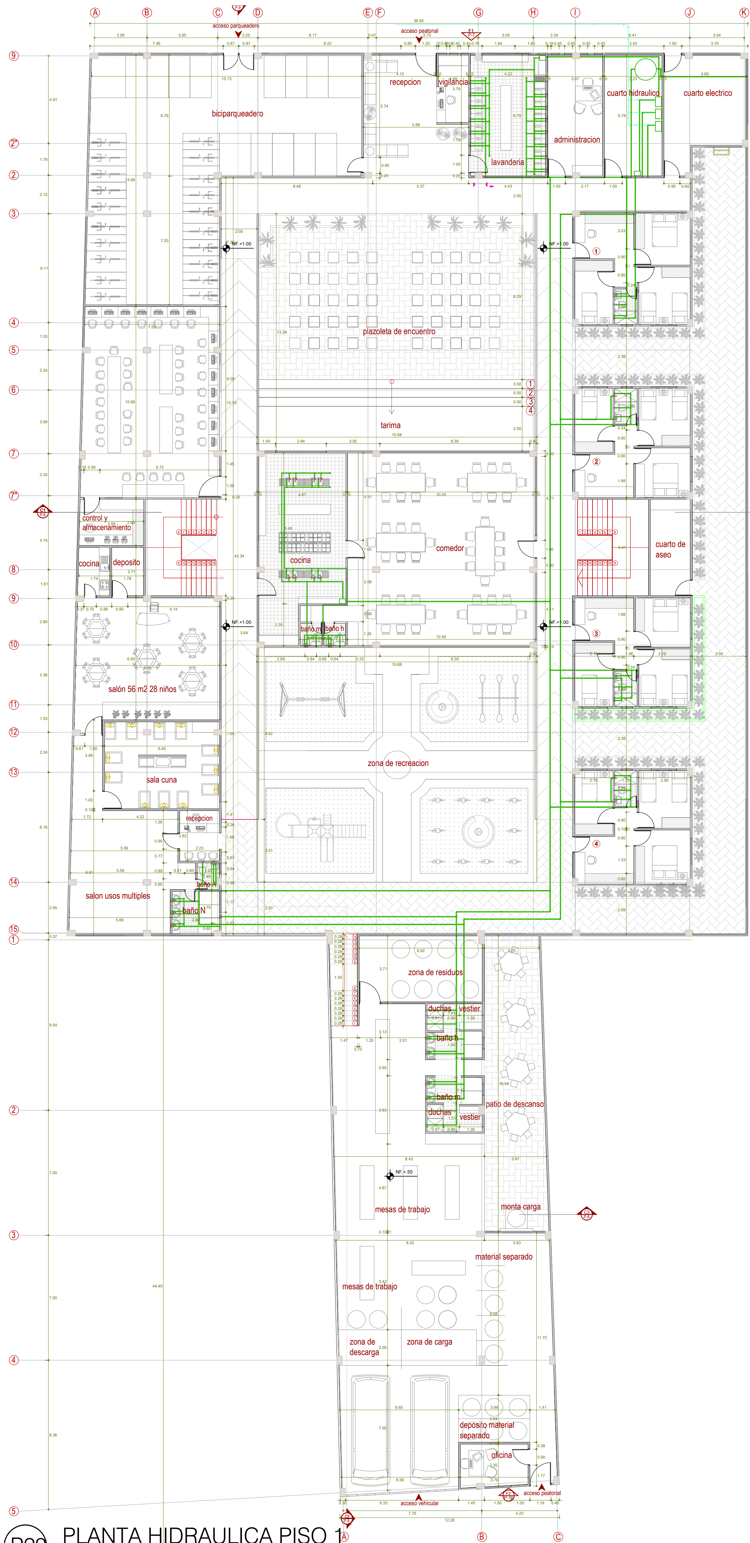
P29 PLANTA HIDRAULICA PISO 1 ESCALA 1:150
