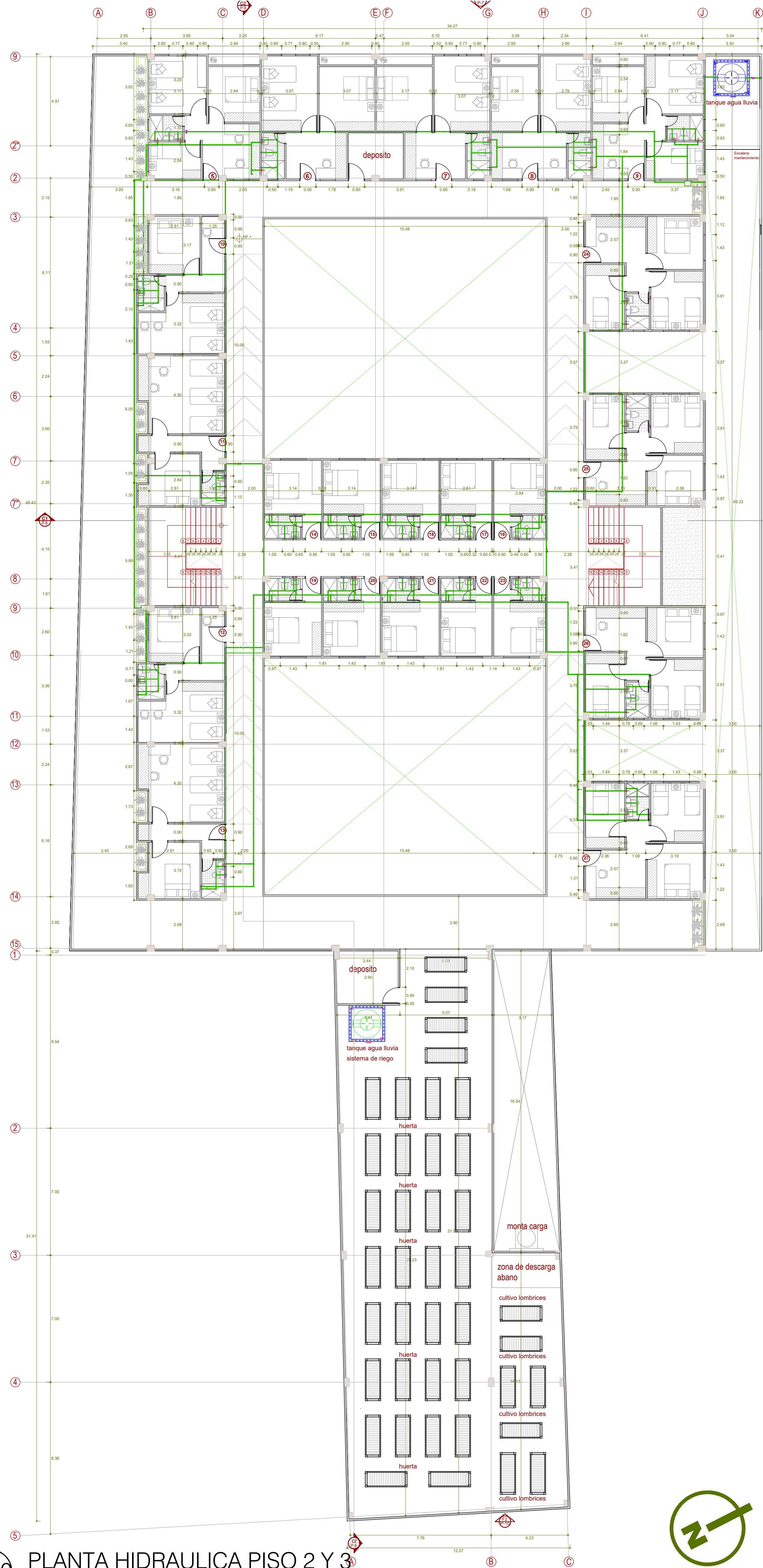
P30 PLANTA HIDRAULICA PISO 2 Y 3 ESCALA 1:150
