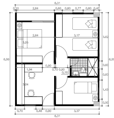
P12 PLANTA TIPOLOGIA 5 ESCALA 1:150
