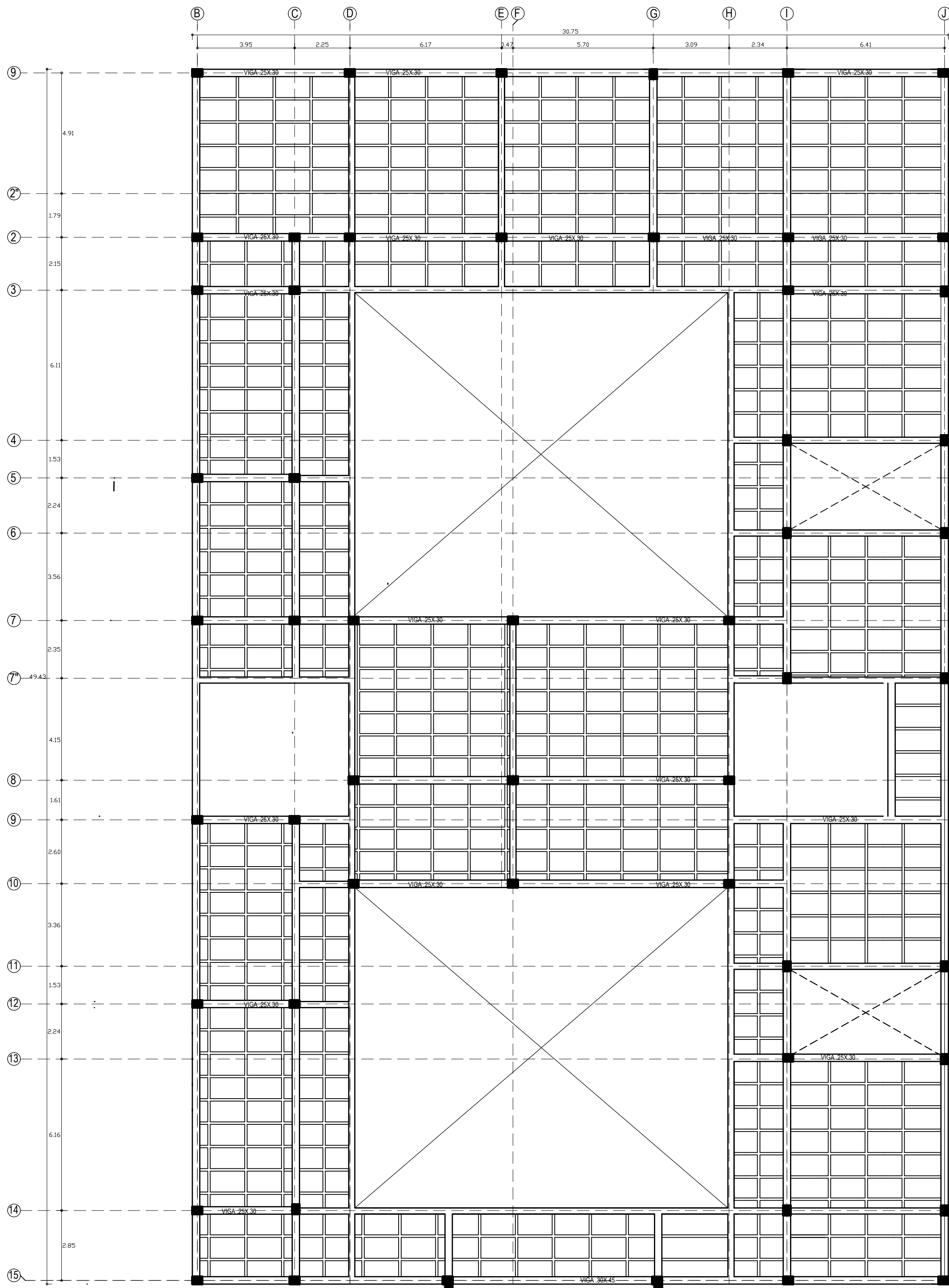
P25 PLANTA CUBIERTA ESCALA 1:150
