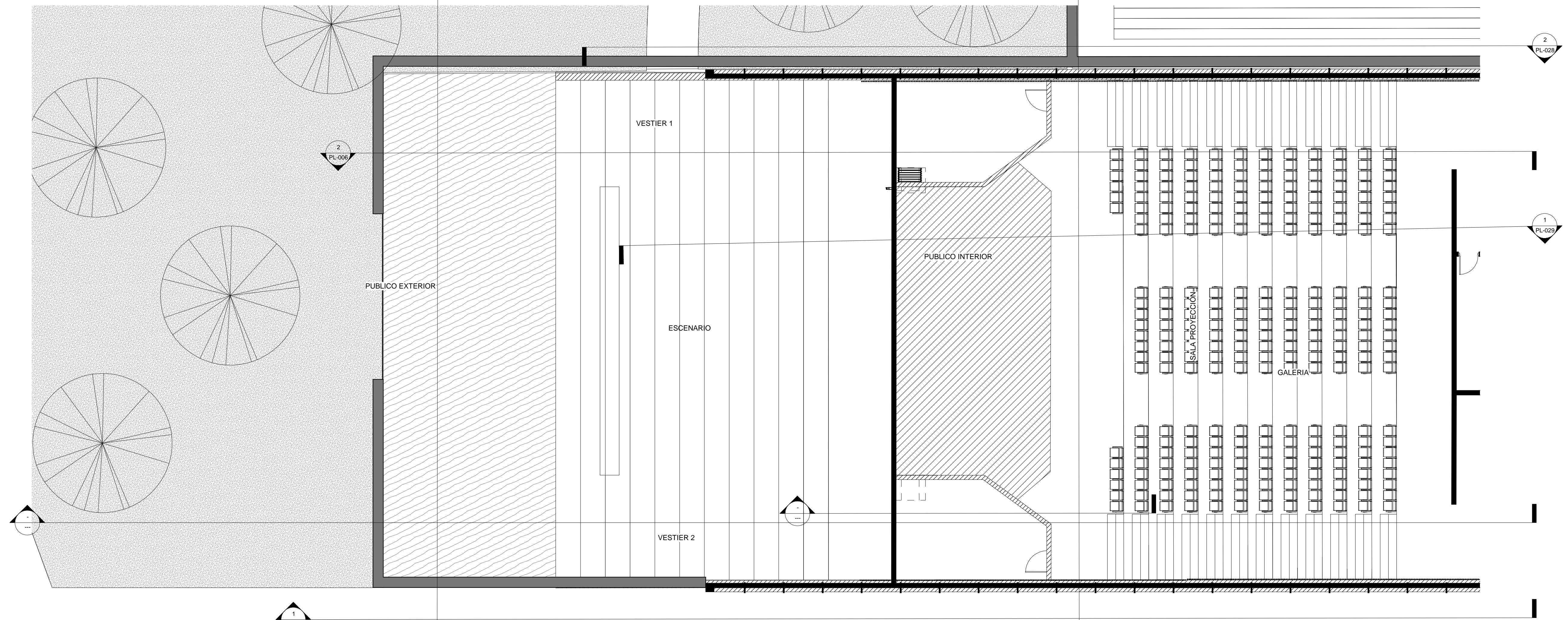
1 PLANTA AUDIOTRIO PISO 1 1 : 100
