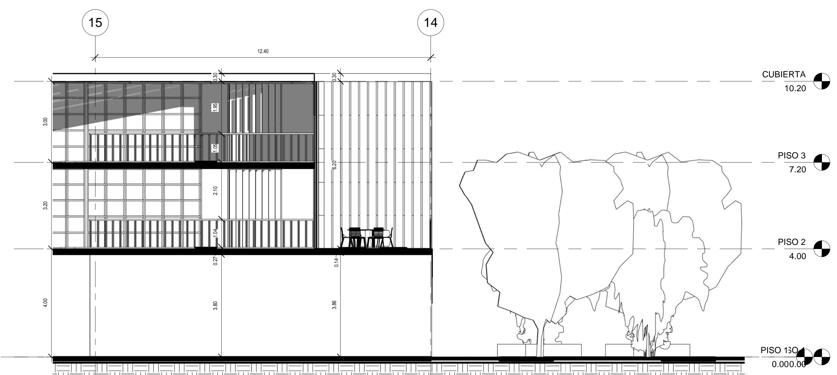
3 CORTE TRANSVERSAL 5 PRIMARIA Y SECUNDARIA 1 : 75
