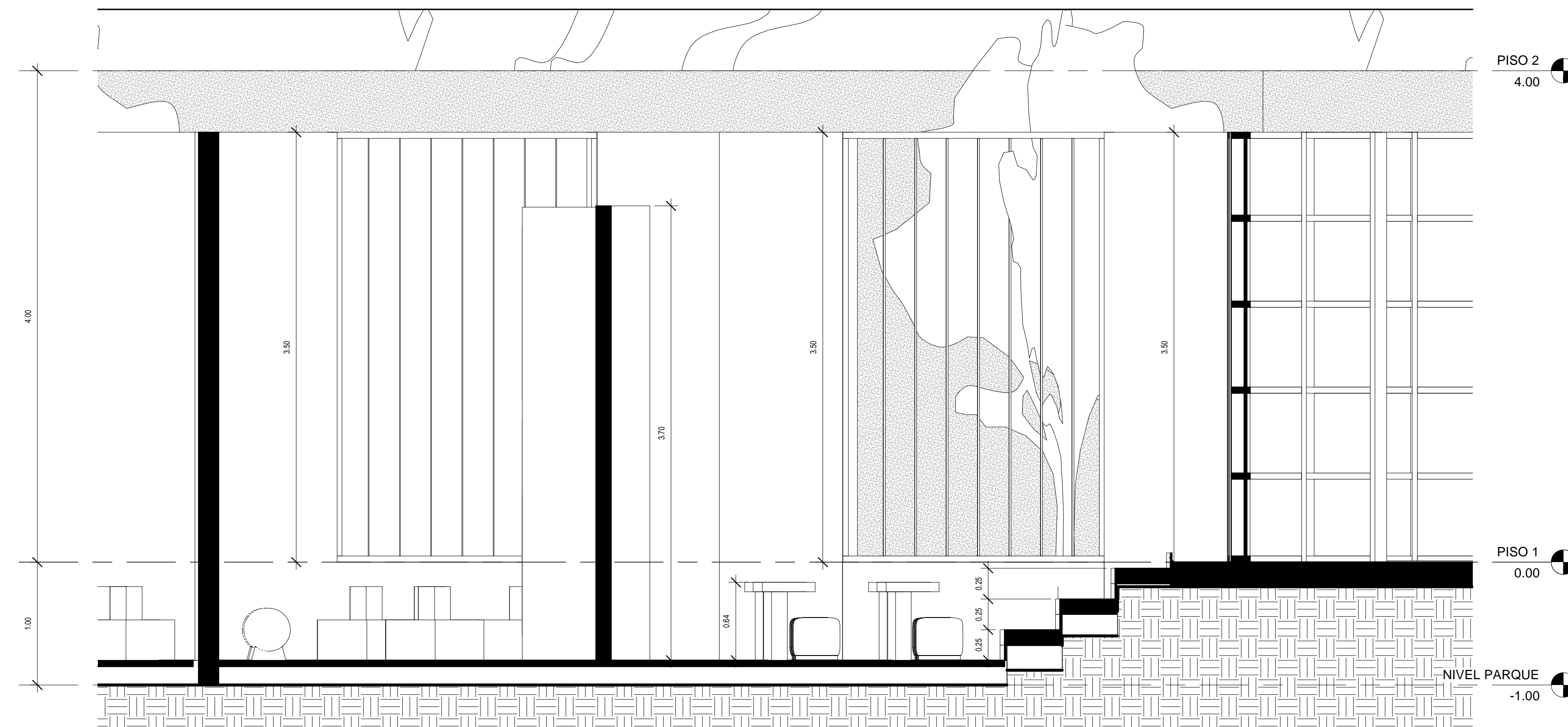
1 CORTE 1 AULA TRANSICION 1 : 25
