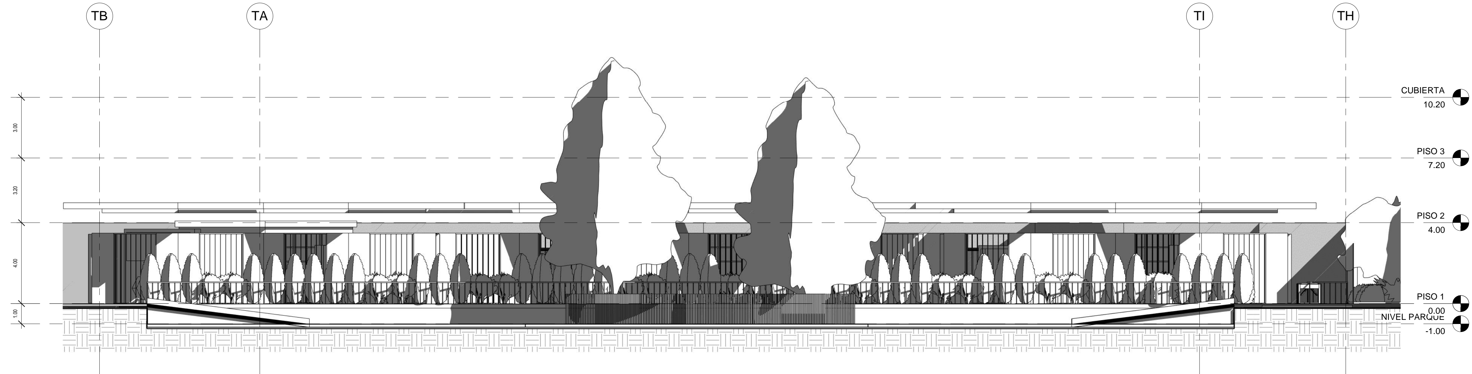
2 CORTE LONGITUDINAL TRANSICION 1:100
