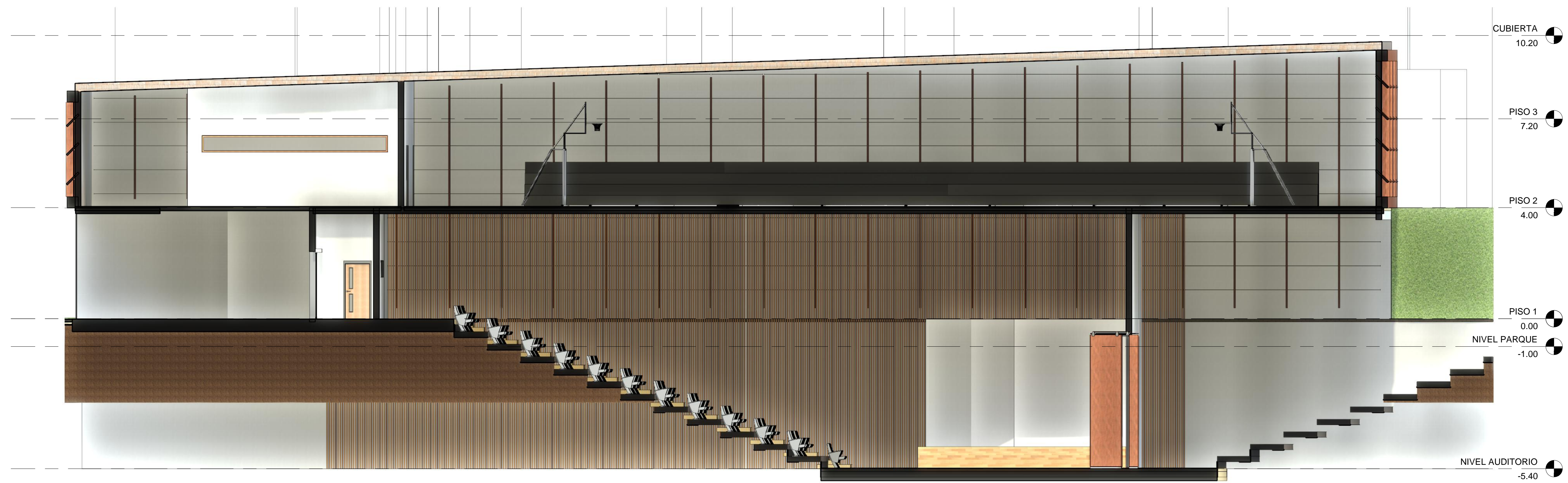
1 CORTE LONGITUDINAL AUDITORIO 1 : 75
