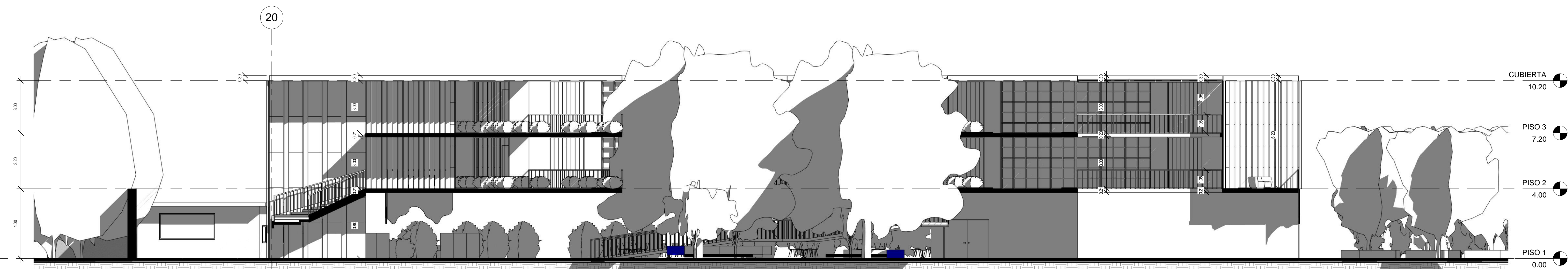
3 CORTE TRANSVERSAL 2 PRIMARIA Y SECUNDARIA 1 : 100
