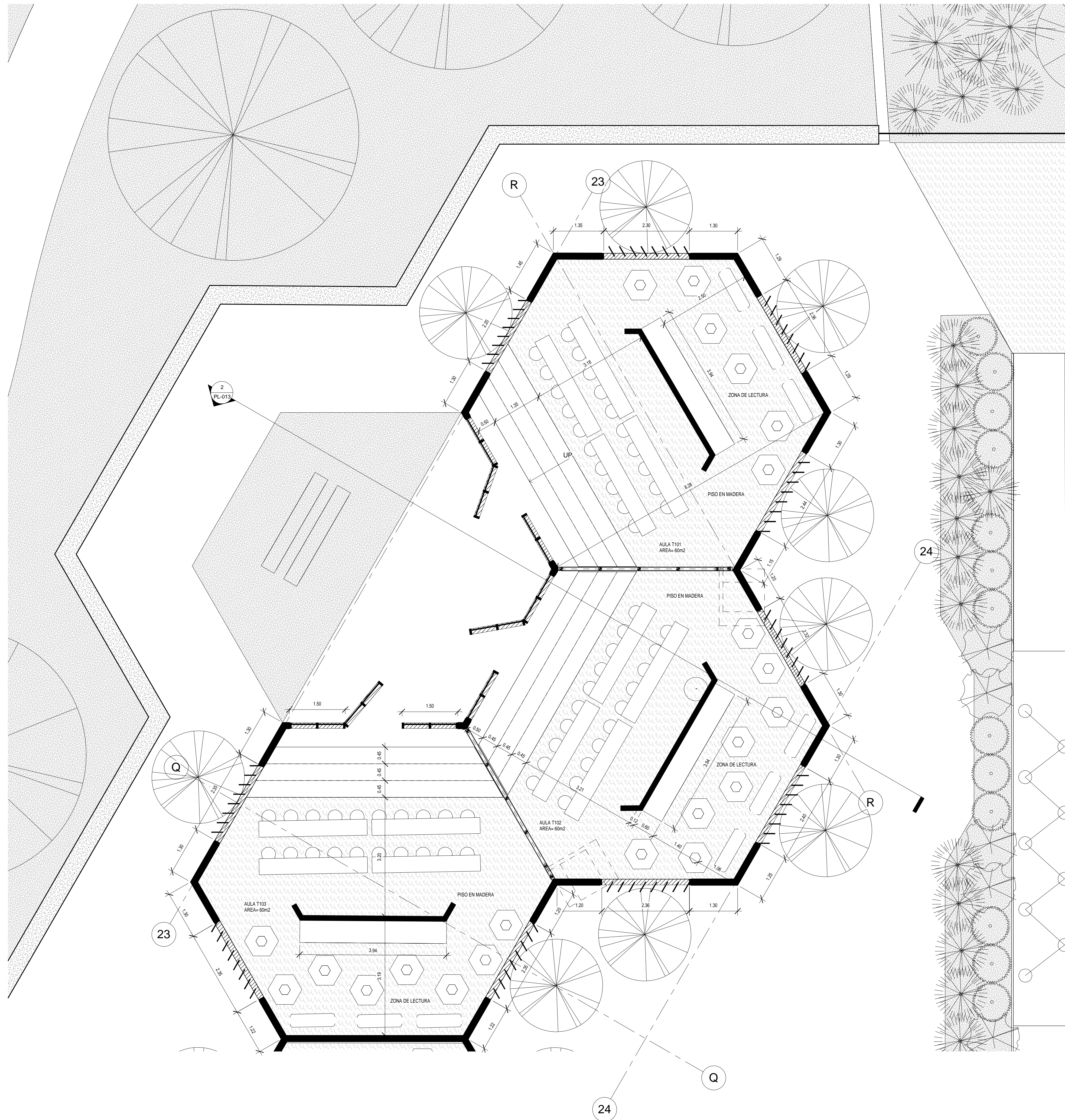
1 GRUPO DE 3 AULAS SIN AGRUPAR 1 : 50
