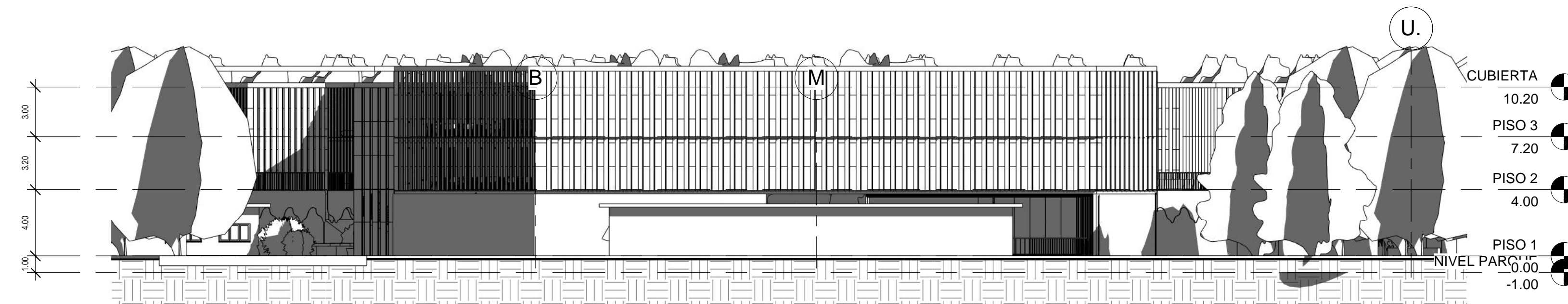
4 FACHADA SUR 1 : 200
