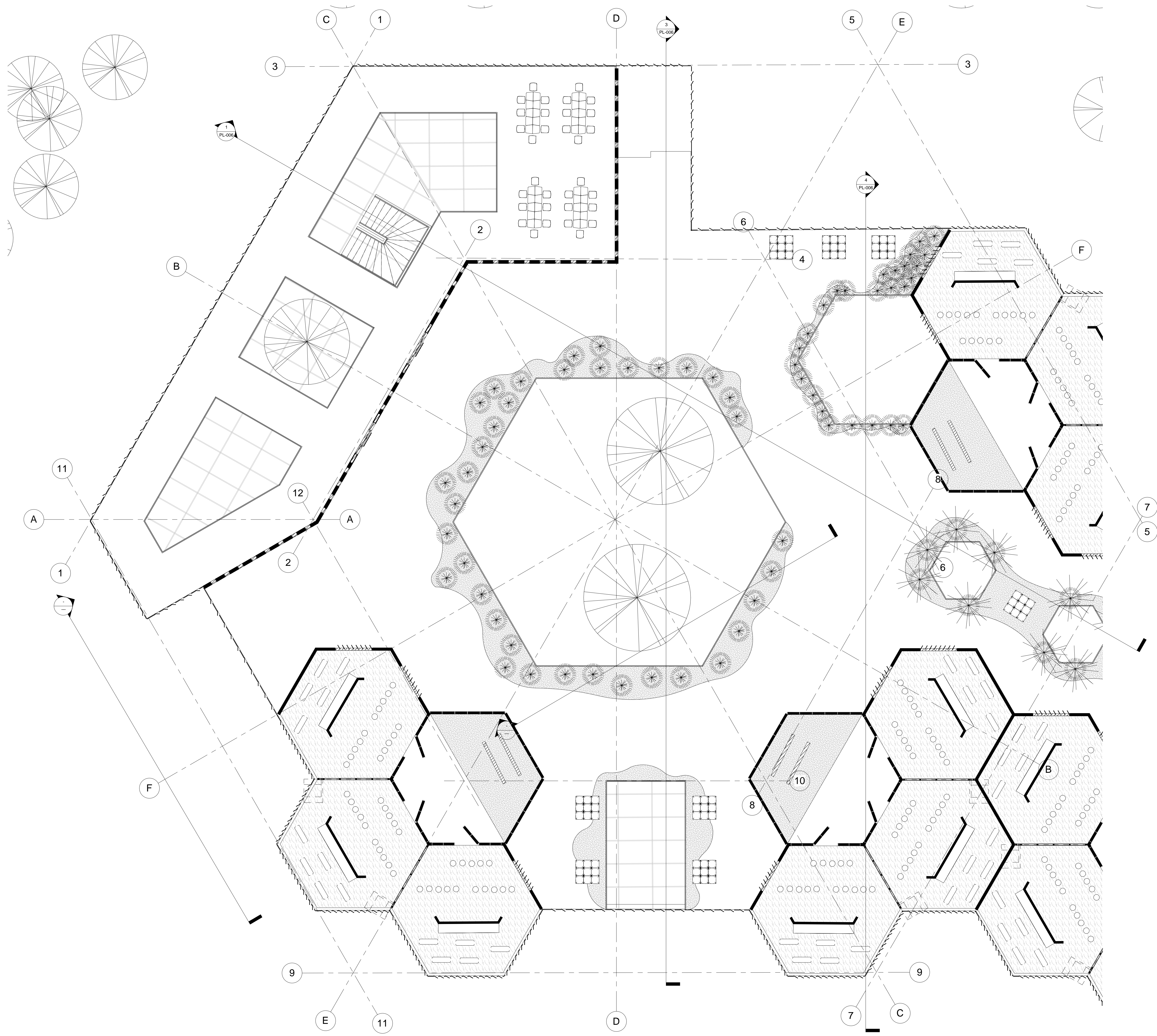
1 PLANTA PRIMARIA PISO 3 1 : 100
