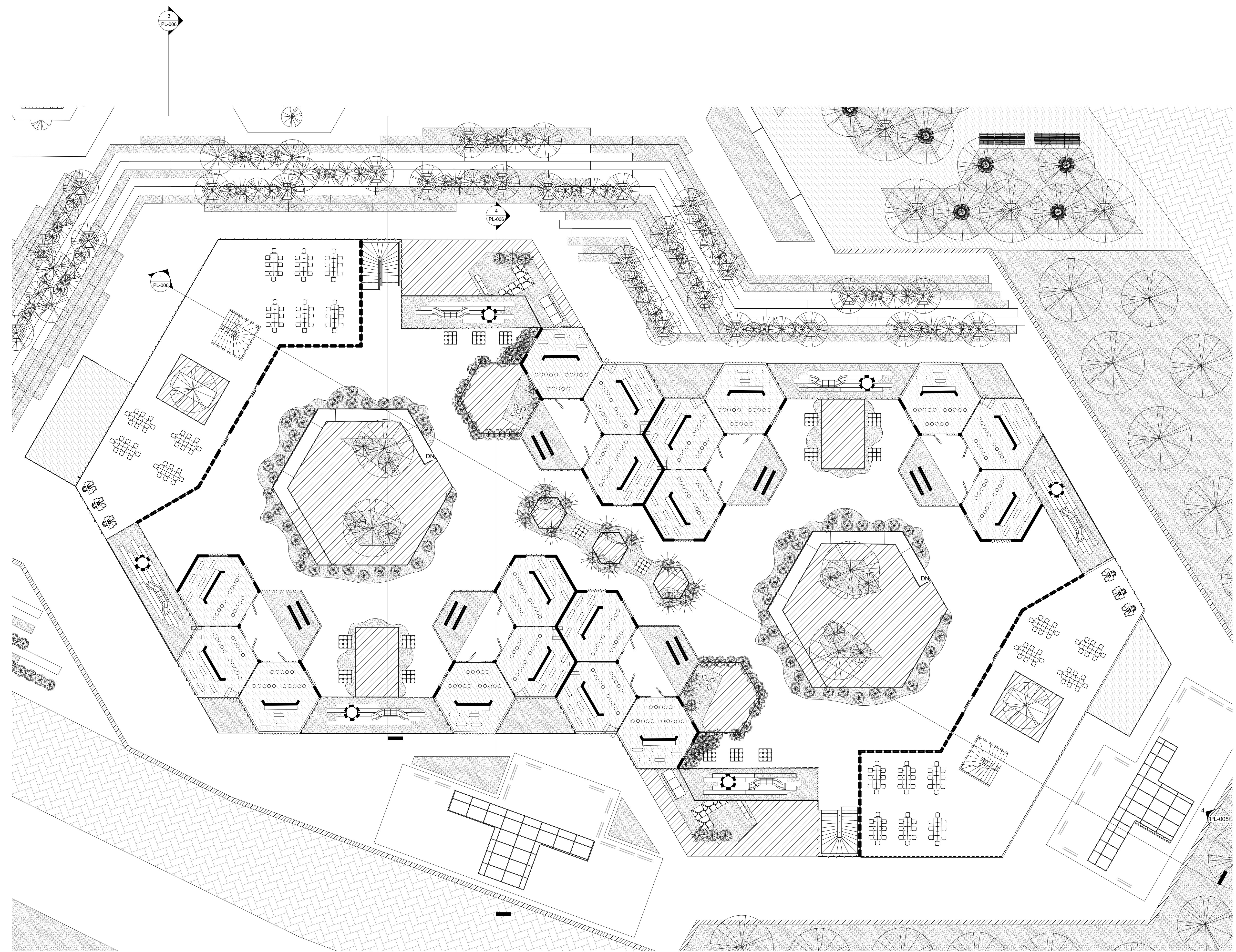
1 PLANTA PRIMARIA-SEGUNDARIA PISO 2 1:200
