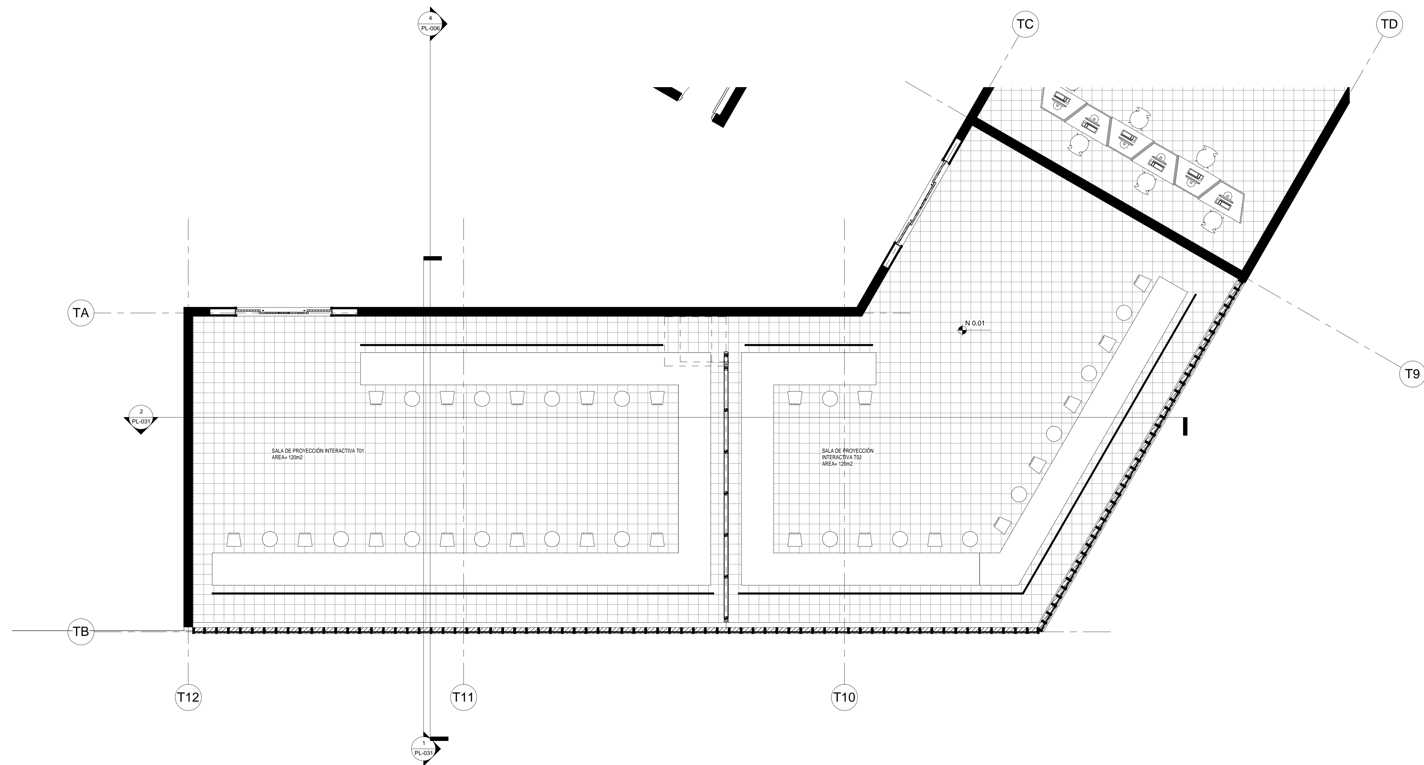
1 PLANTA SALA DE PROYECCION INTERACTIVA 1 : 50
