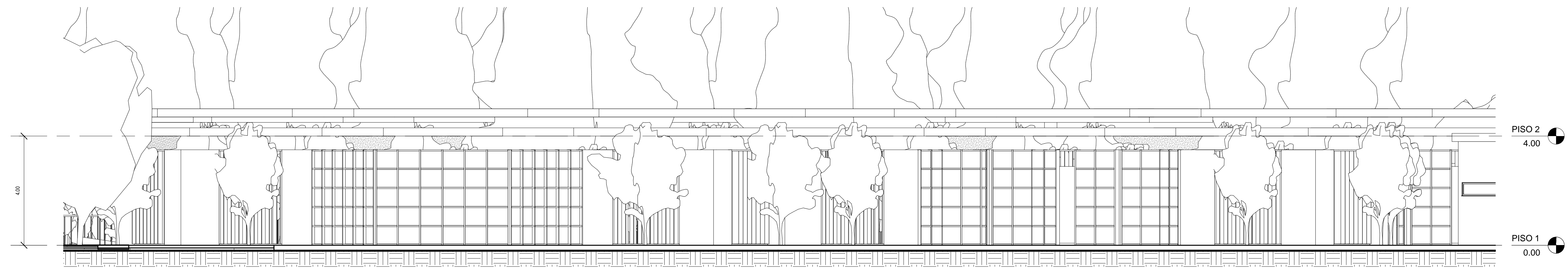
1 FACHADA 1 TRANSICION 1 : 75
