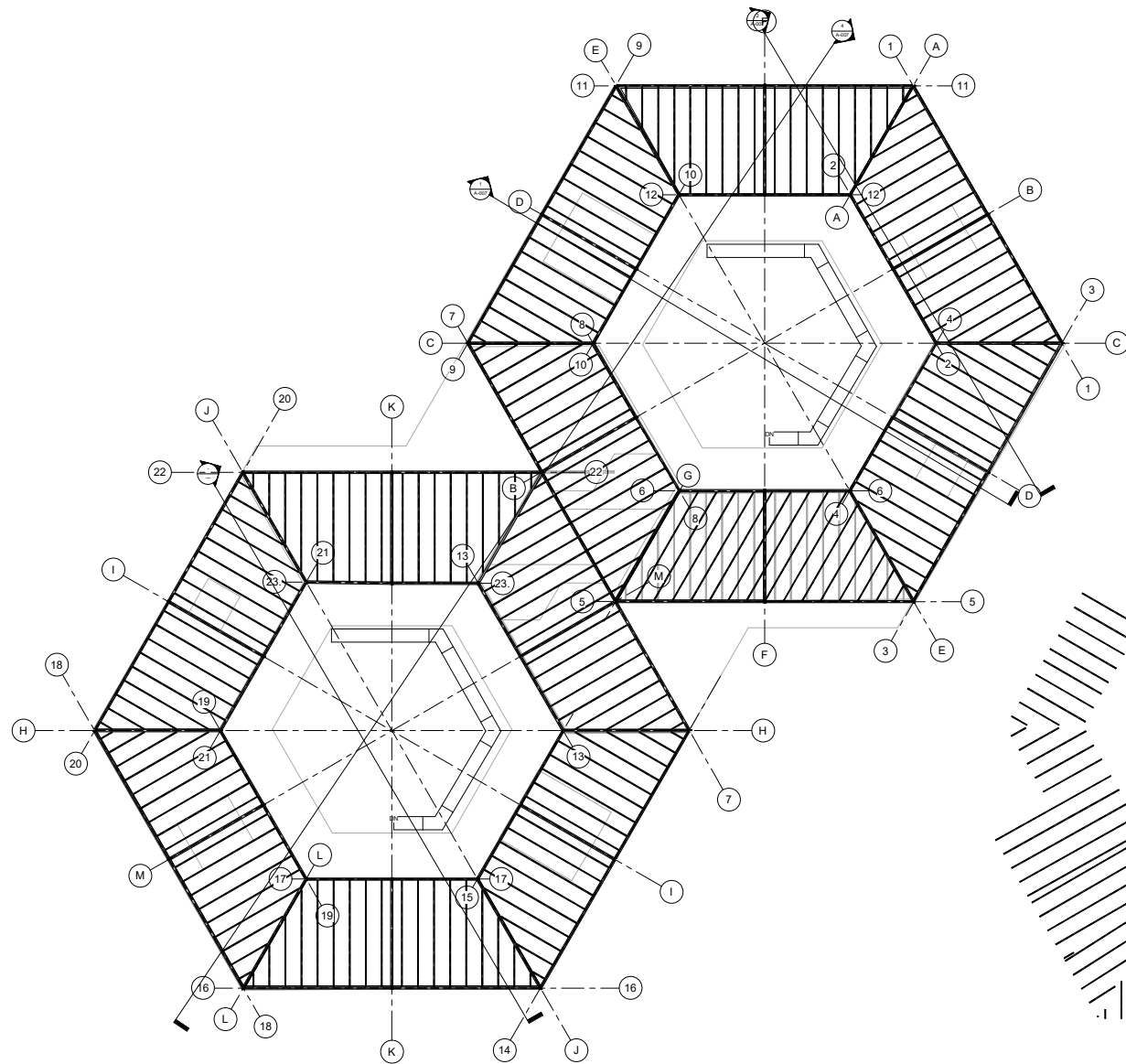
1 ESTRUCTURA NIVEL 3 1 : 200
