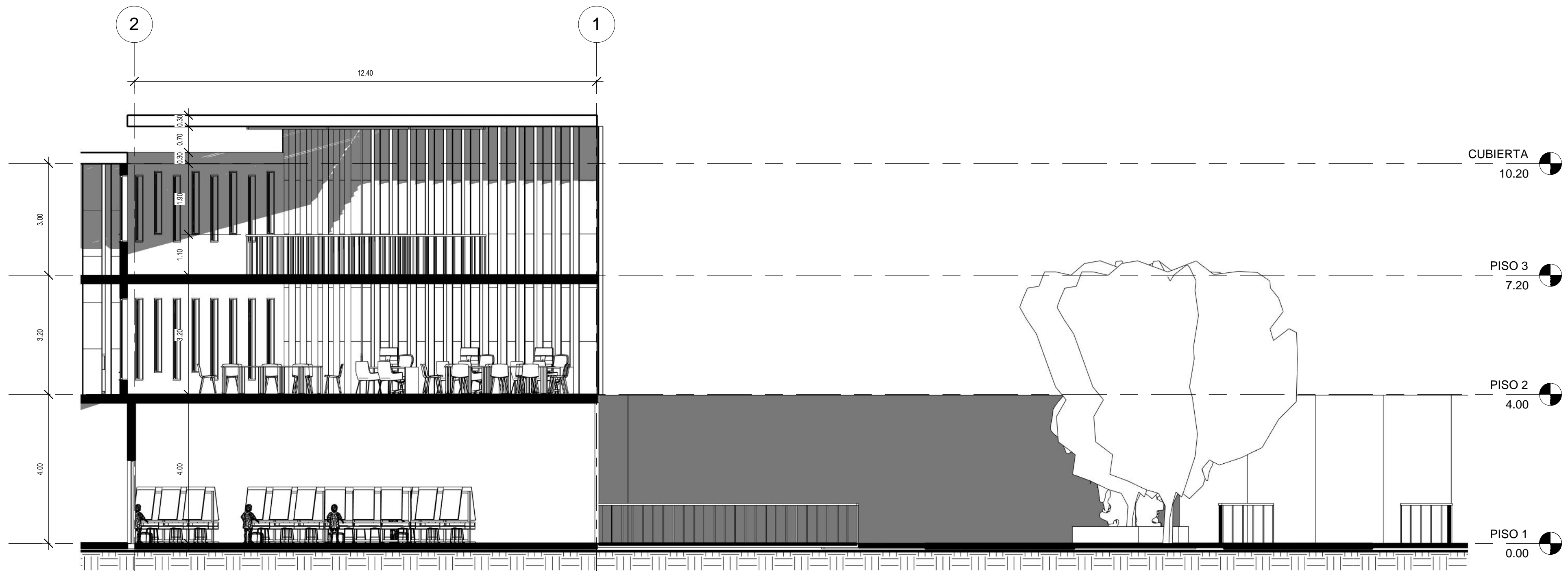
2 CORTE TRANSVERSAL 4 PRIMARIA Y SECUNDARIA 1 : 75
