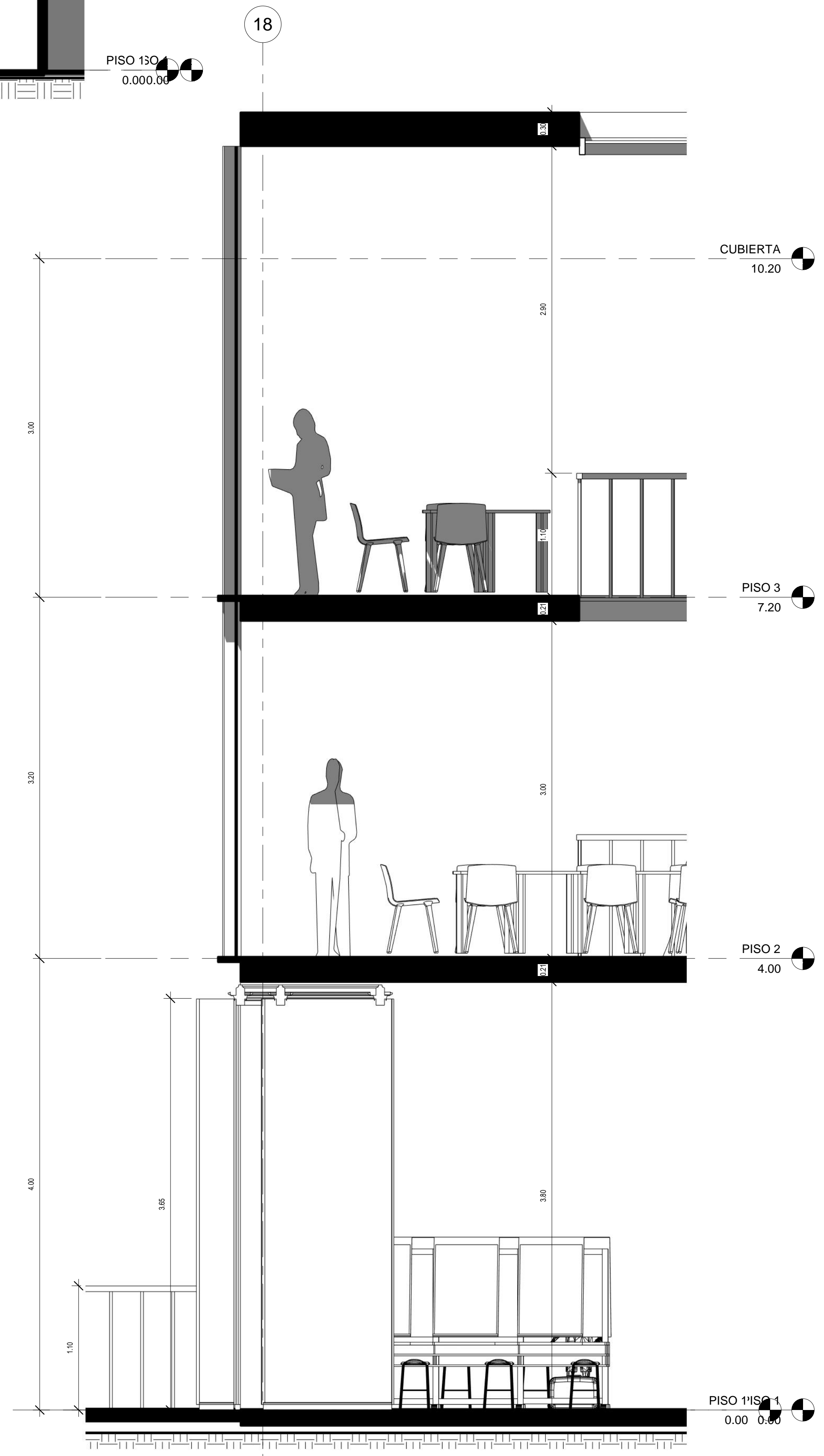
4 CORTE FACHADA 1 : 25
