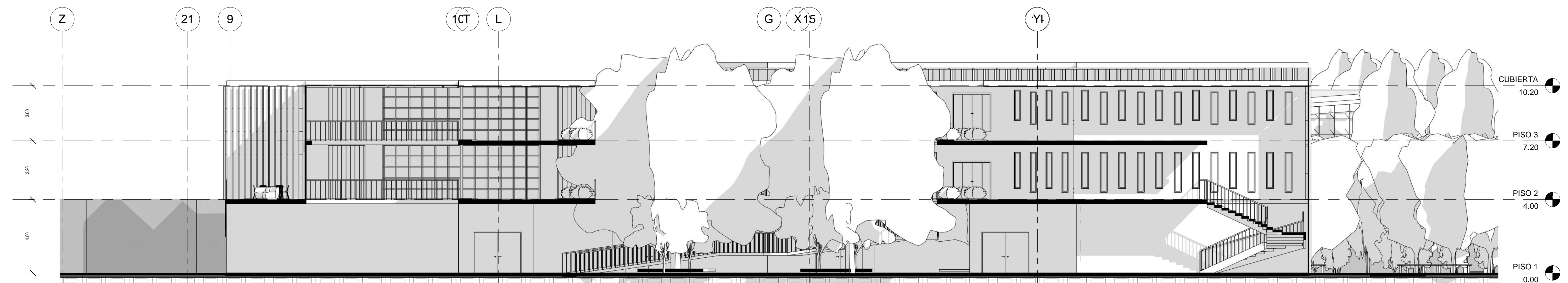
1 CORTE TRANSVERSAL 1 PRIMARIA Y SECUNDARIA 1 : 100
