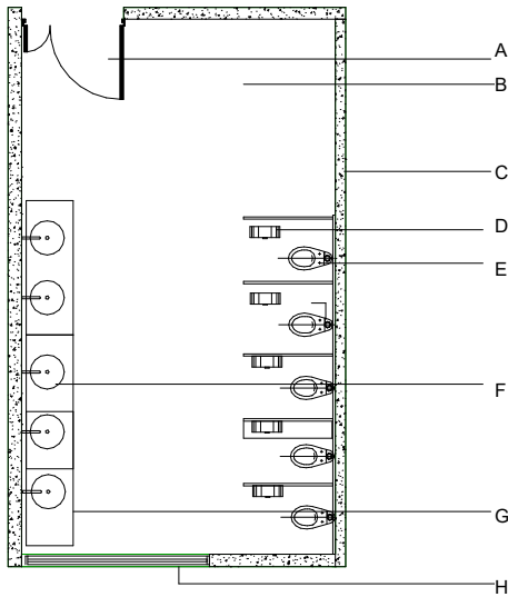
PLANTA BAÑO HOMBRES
