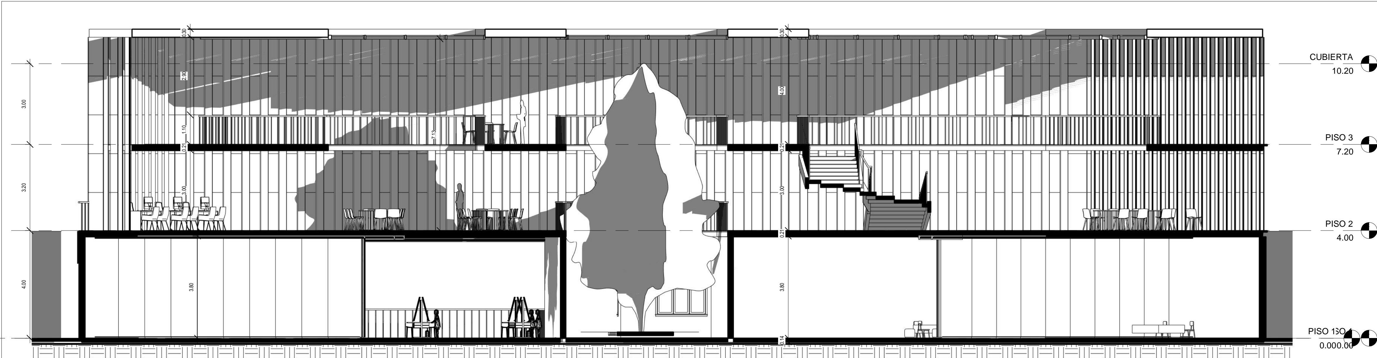
1 CORTE TRANSVERSAL 3 PRIMARIA Y SECUNDARIA 1 : 75
