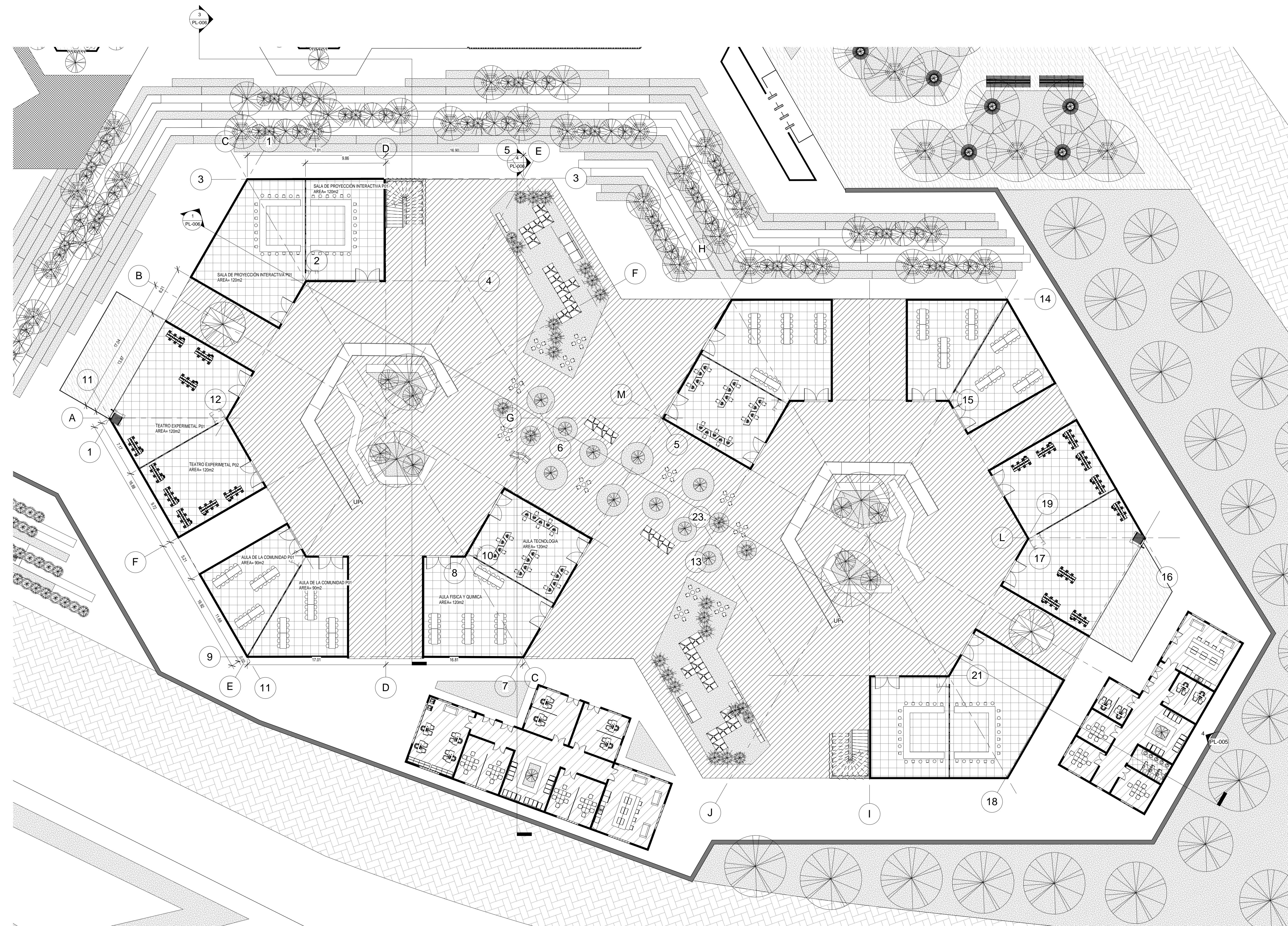
1 PLANTA PRIMARIA-SECUNDARIA PISO 1 1 : 200
