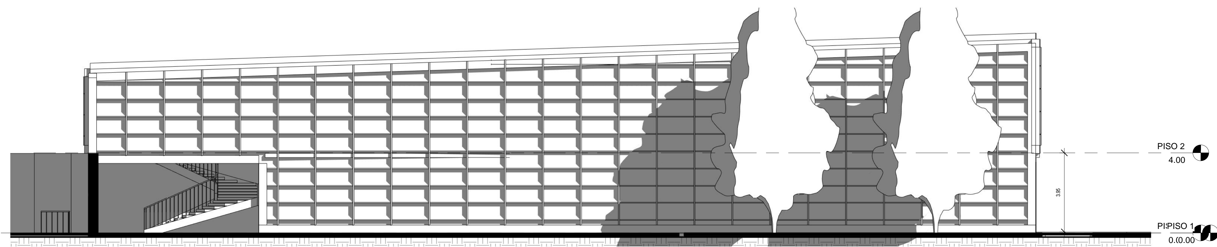
2 FACHADA ORIENTAL AUDITORIO 1:100
