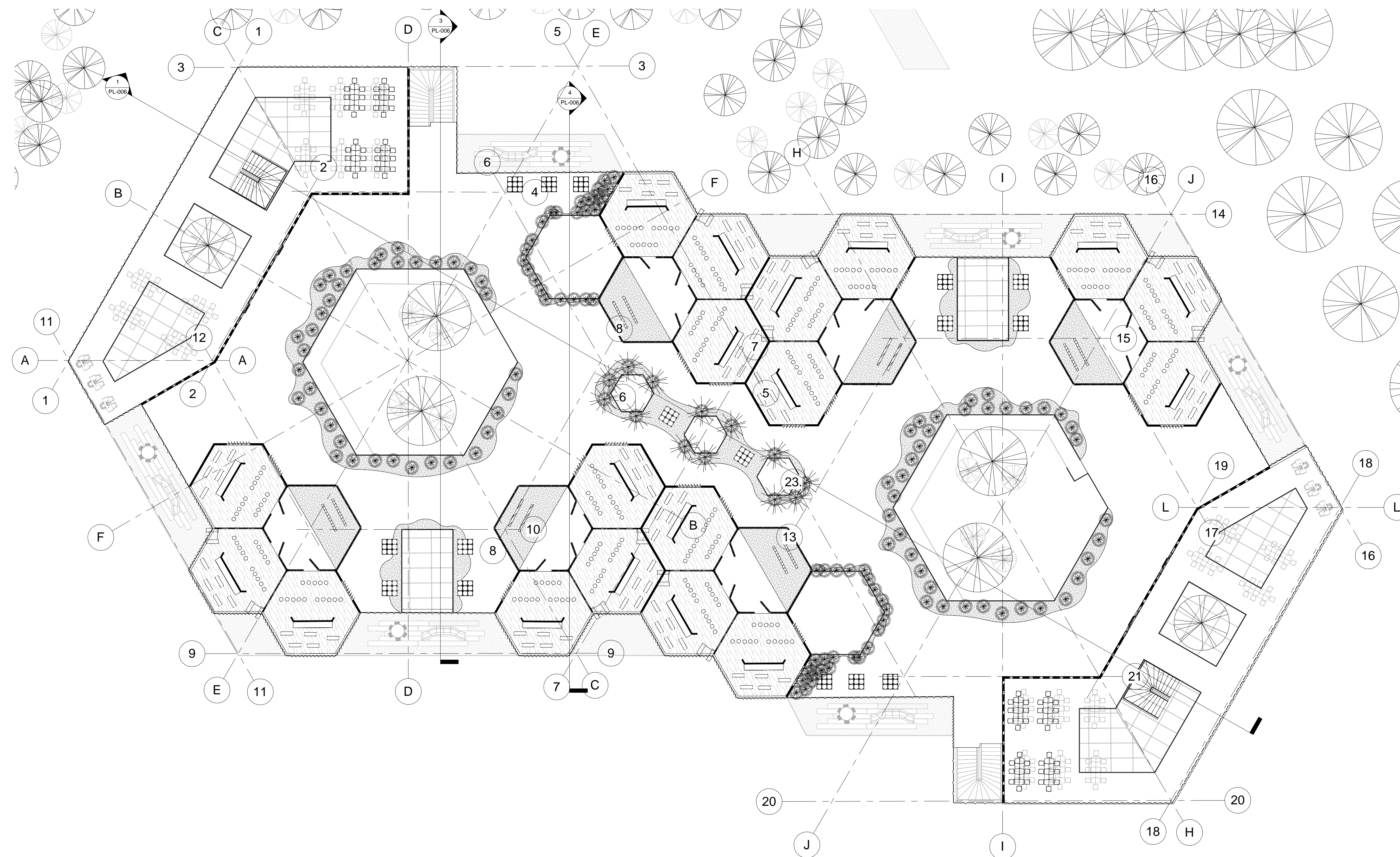
1 PLANTA PRIMARIA-SECUNDARIA PISO 3 1 : 200
