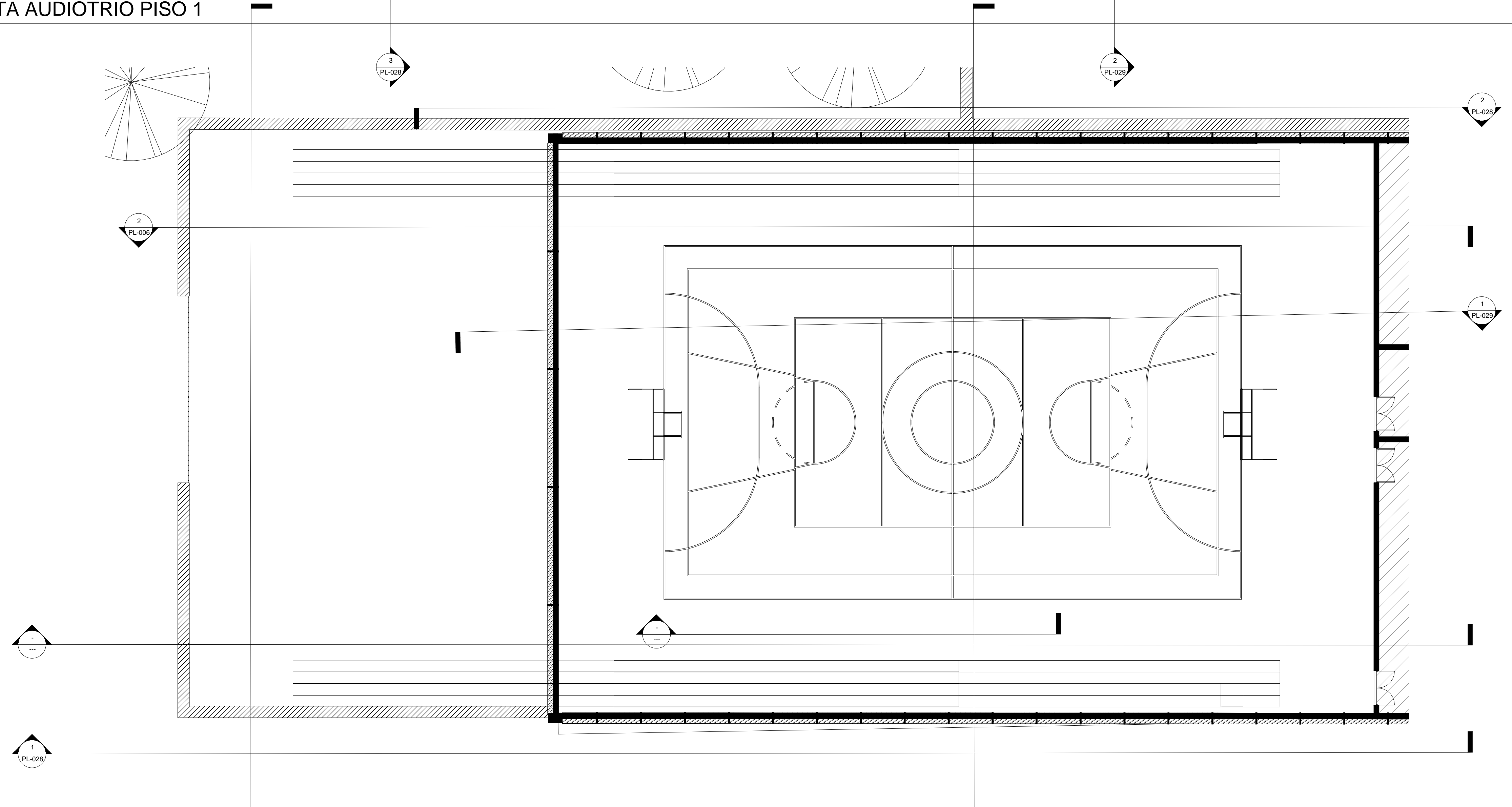
2 PLANTA CANCHA PISO 2 1 : 100
