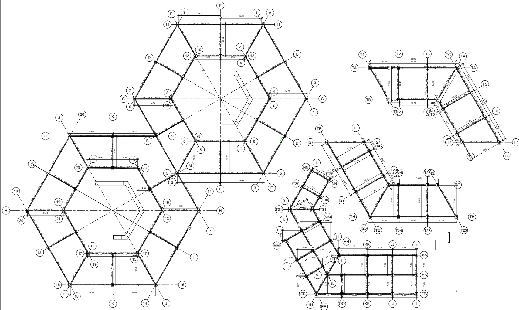
1 ESTRUCTURA NIVEL 1 1 : 230
