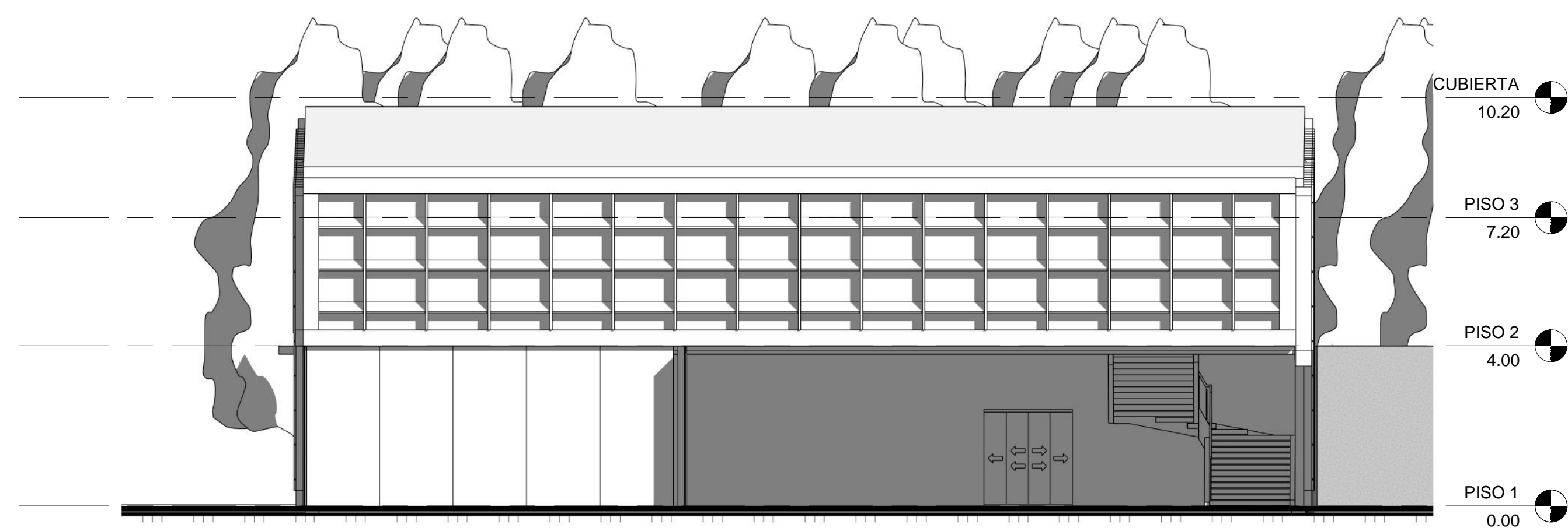
4 FACHADA SUR AUDITORIO 1:100
