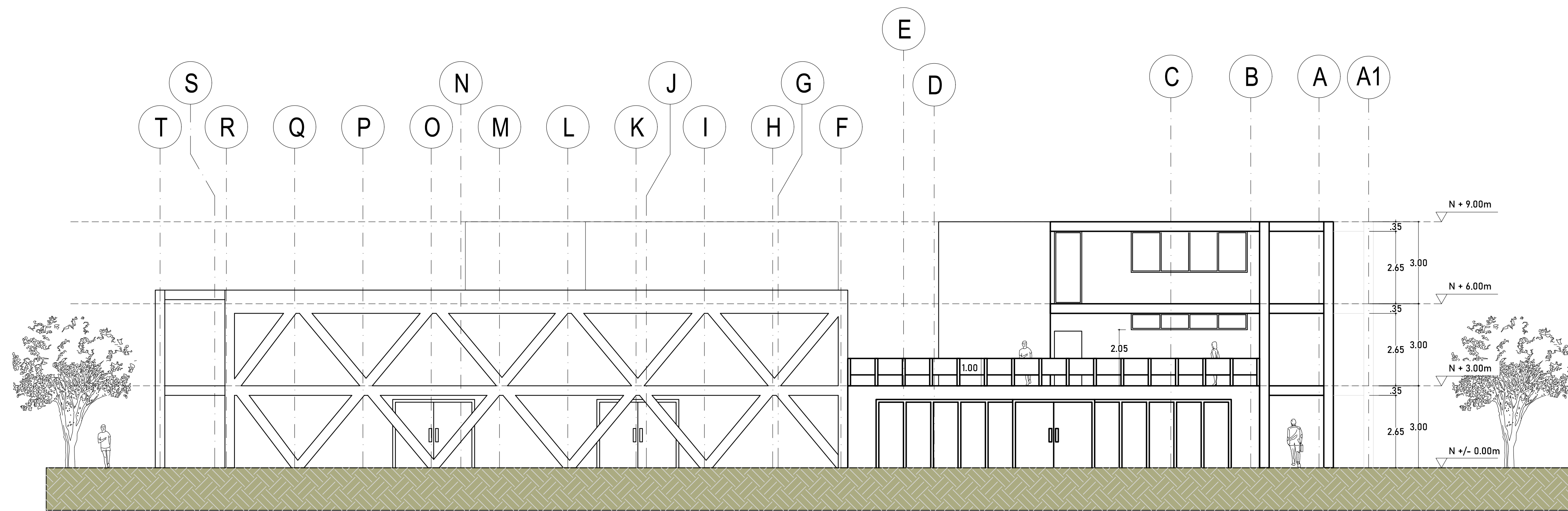
F1 FACHADA LATERAL IZQUIERDA Esc 1:100
