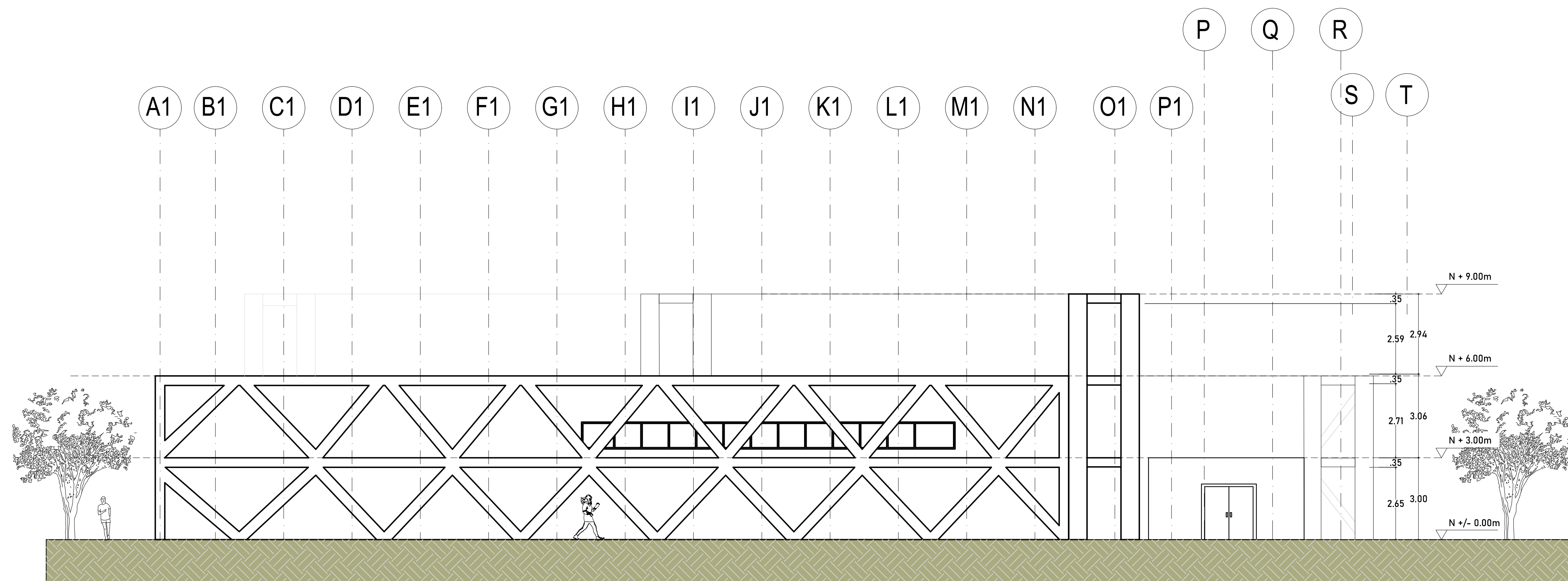
F3 FACHADA LATERAL DERECHA Esc 1:100
