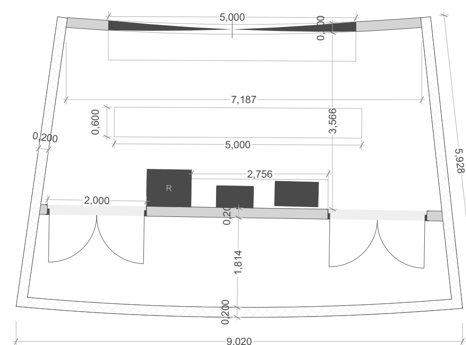
P18 ALMACEN COMIDAS 1 1:75
