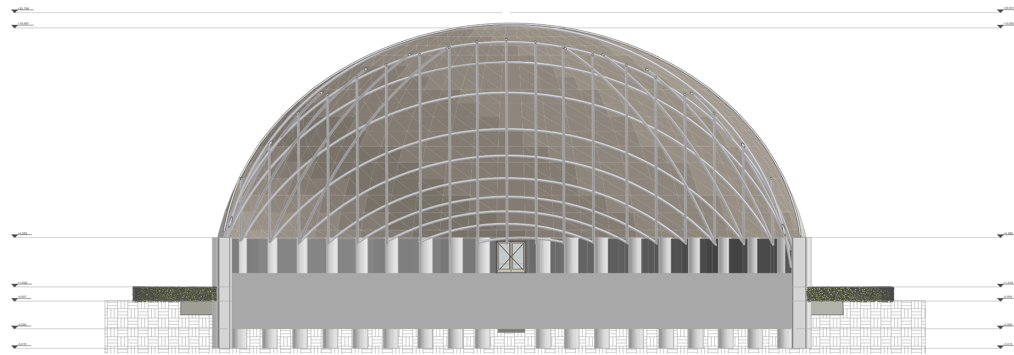
A-06 ALZADO TARIMA 1 P1 1:250
