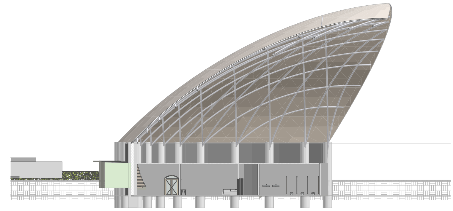
A-05 CORTE TARIMA 1 P1 1:250
