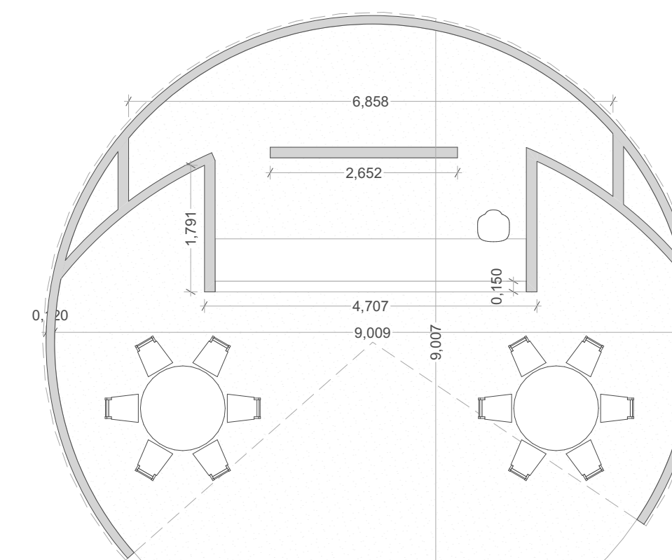
P19 ALMACEN COMIDAS 2 1:75
