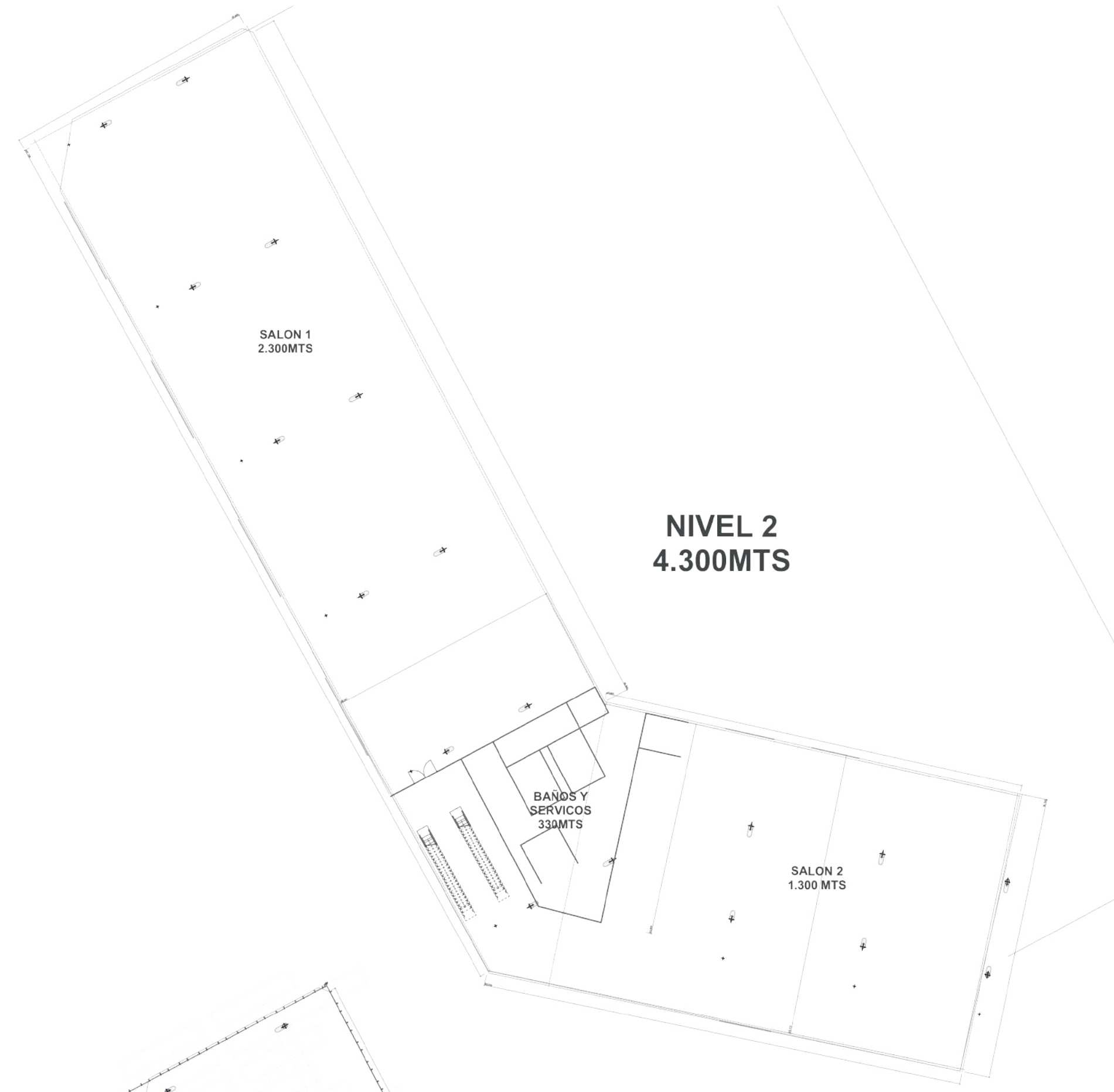
P2 SEGUNDO NIVEL 1:500
