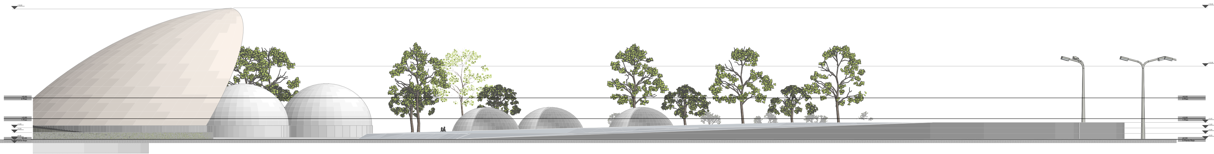
A-03 ALZADO NORTE TARIMA 2 P1 1:300
