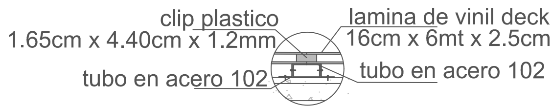
U DETALLE 1 ESC__ 1:8
