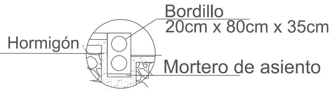
U DETALLE 2 ESC__ 1:20
