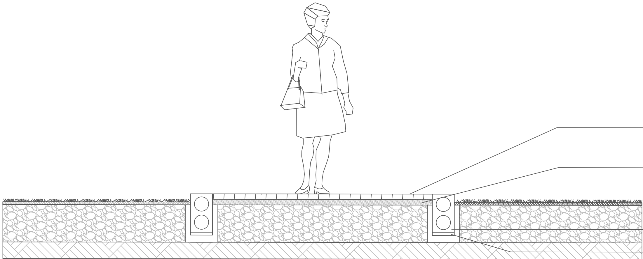
U CORTE A-A' ESC_1:20
