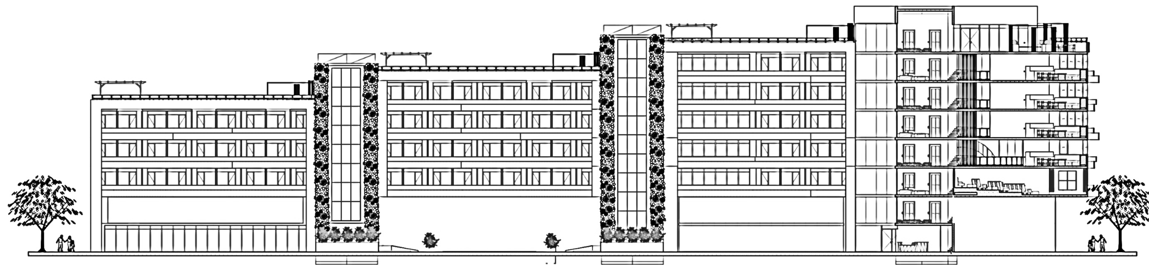
FACHADA SUR ESC 1:200
