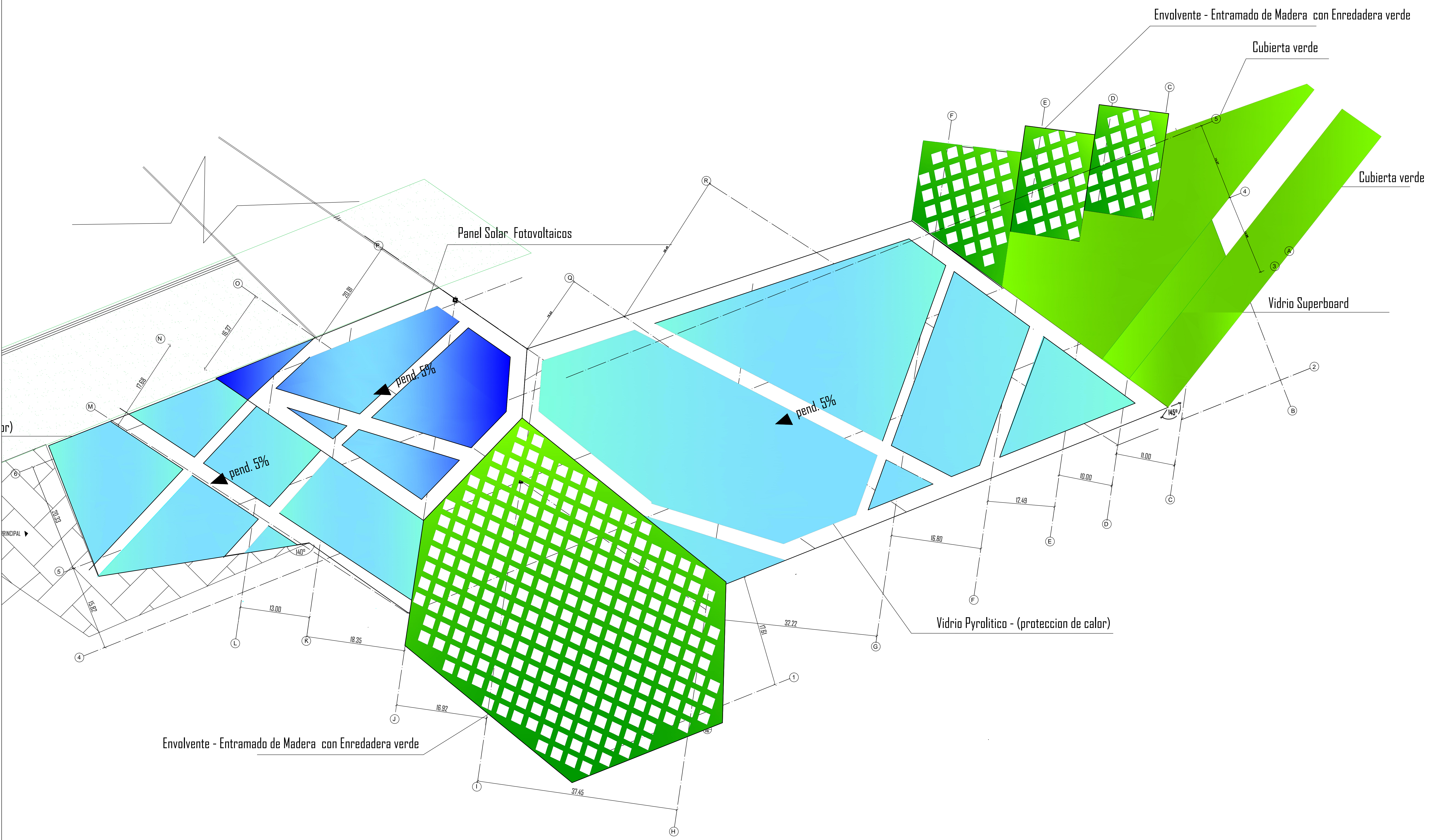
A6 PLANTA CUBIERTAS ASAMBLEAS ESCALA 1:300
