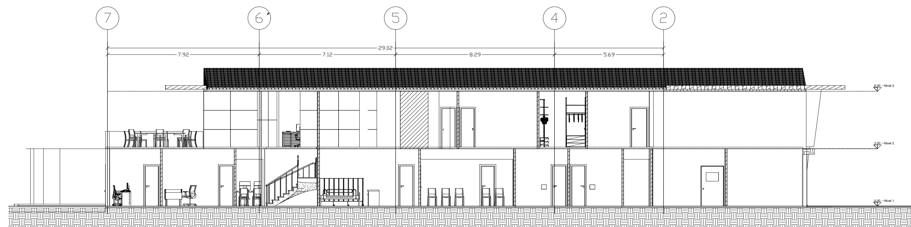
A-O CORTE LONGITUDINAL A-000 ESCALA 1:100 ESCALA GRAFICA: 1/100 0 1 2 3 4 5 (m.)
