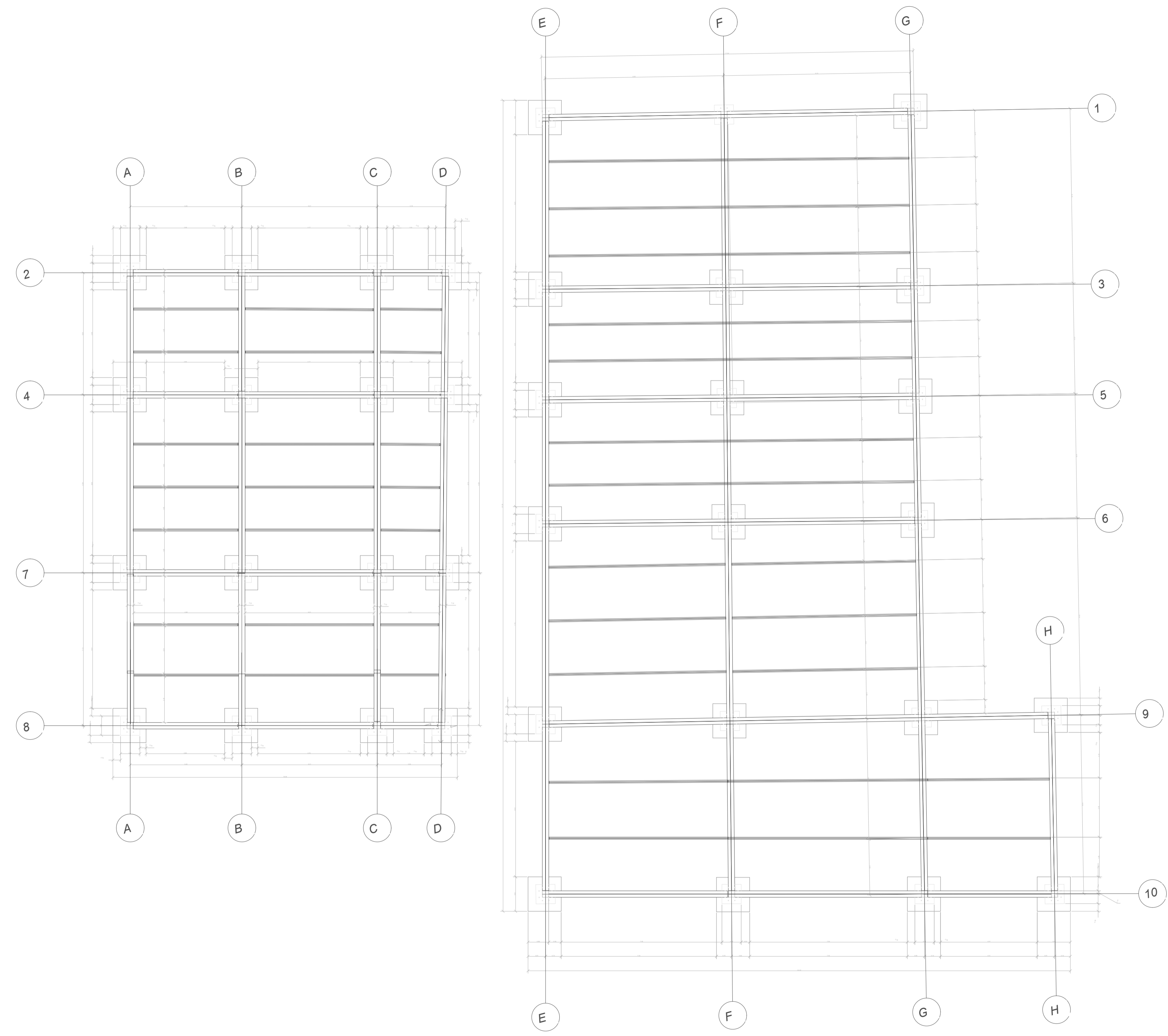
A-O A-000 EJES Y CIMIENTOS ESCALA 1:100
