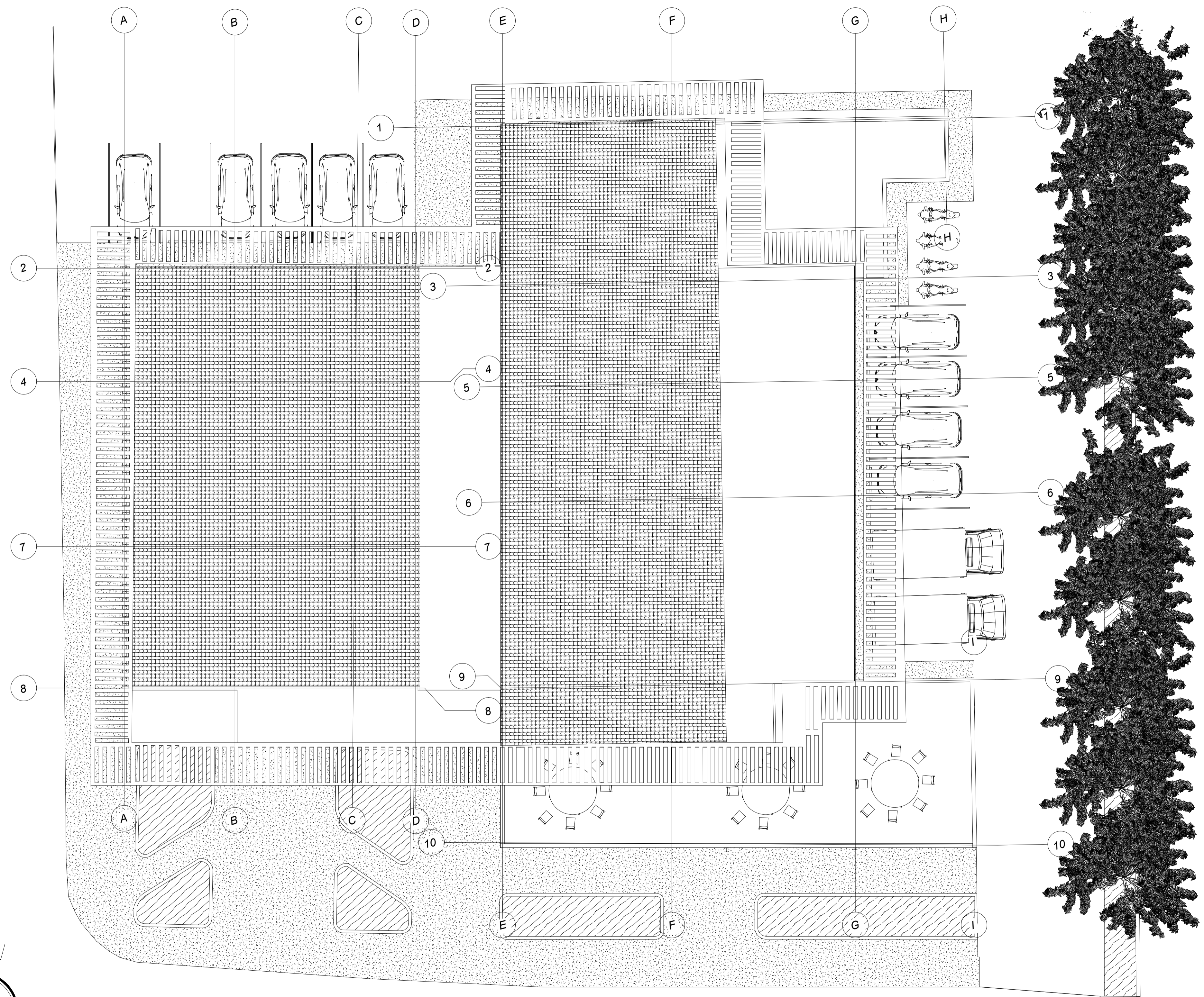
P-4 CUBIERTA A-004 ESCALA 1:100
