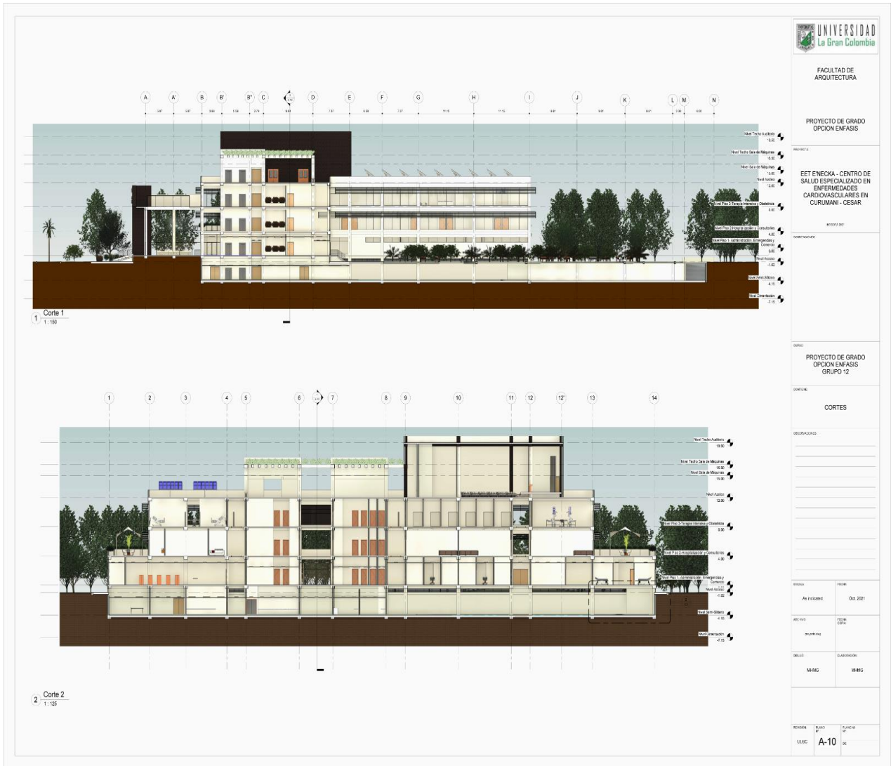
Corte de fachada 2
