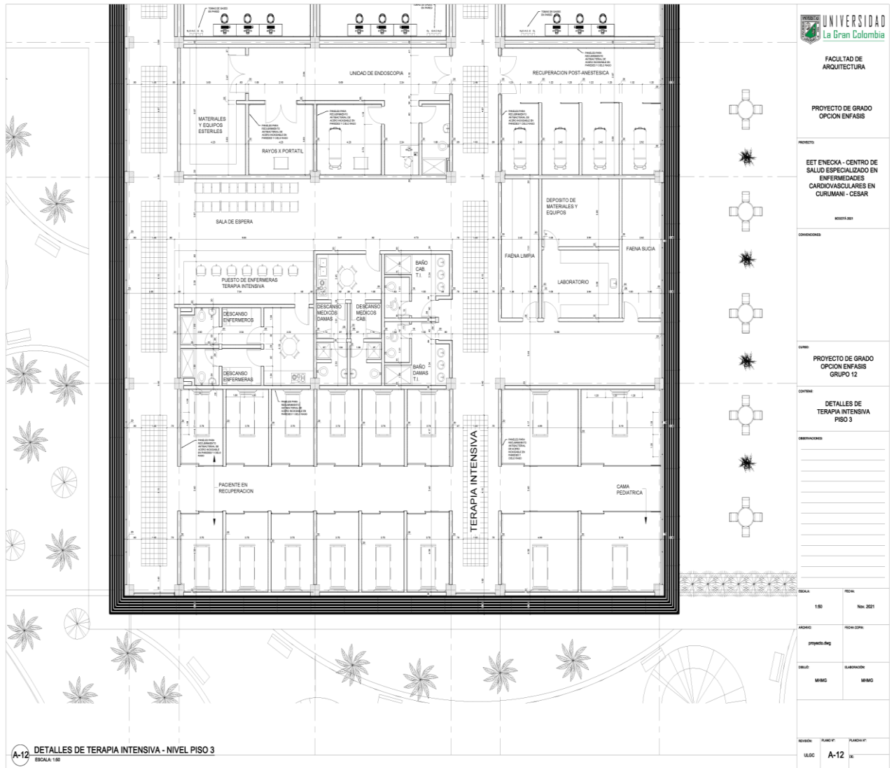
Detalle terapia intensiva
