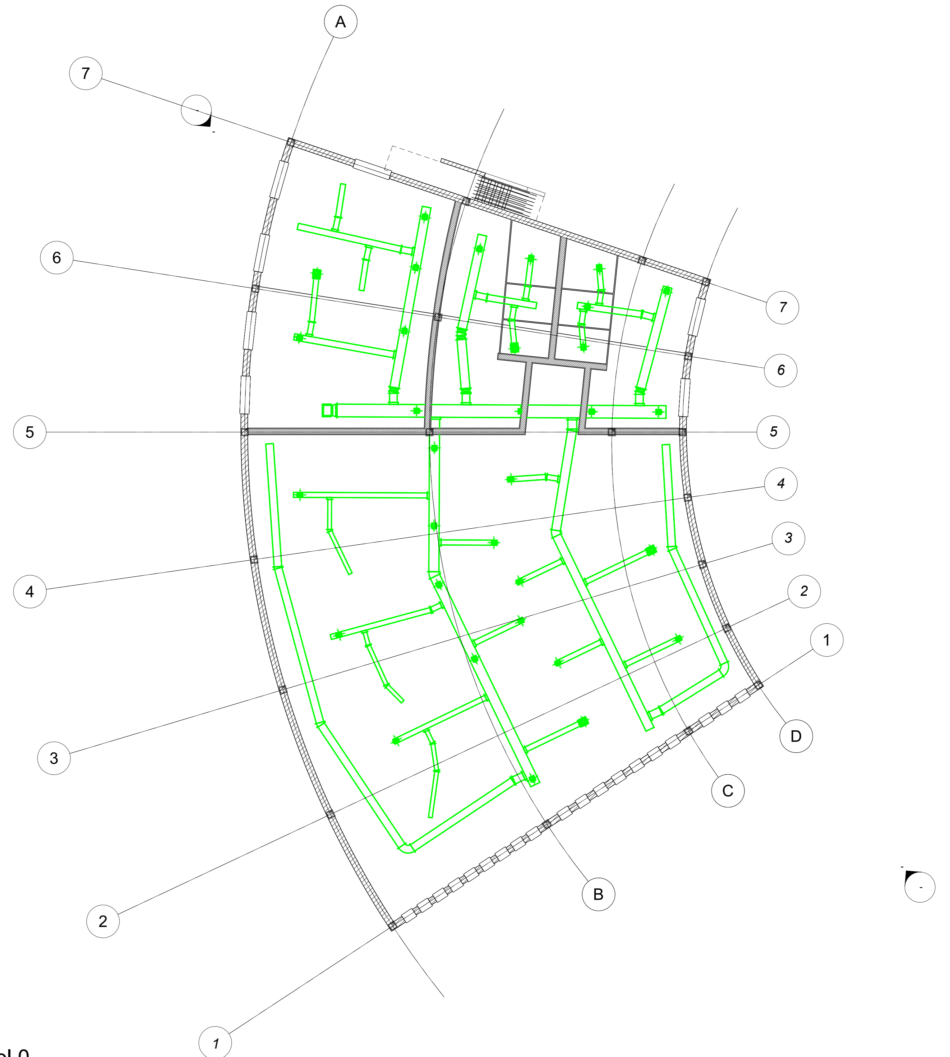
3 Nivel 0 1 : 100
