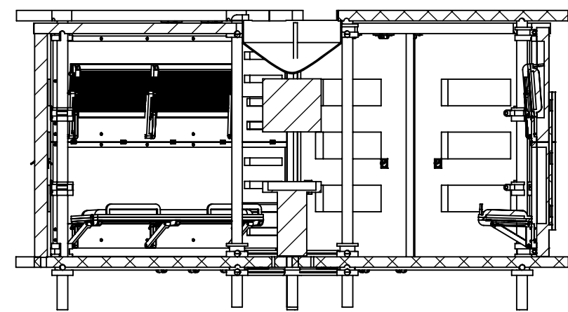
SECCIÓN A-A
