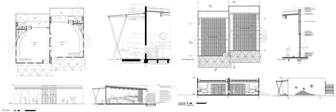
Figura 77 Plantas, Cortes y fachadas Arquitectónicas./Centro de Desarrollo Infantil El Guadual Tomado de: www.archdaily.com/ Centro de Desarrollo Infantil El Guadual
