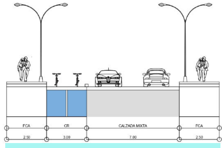
CARRERA 104 - SECCIÓN LONGITUDINAL
