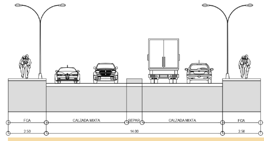
CARRERA 106 - SECCIÓN LONGITUDINAL
