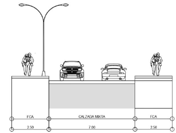
CALLE 13 - SECCIÓN TRANSVERSAL
