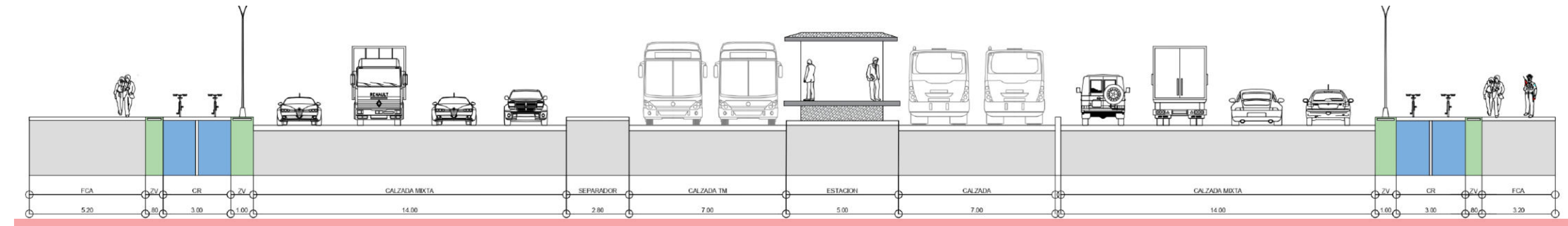
CALLE 13 - SECCIÓN TRANSVERSAL
