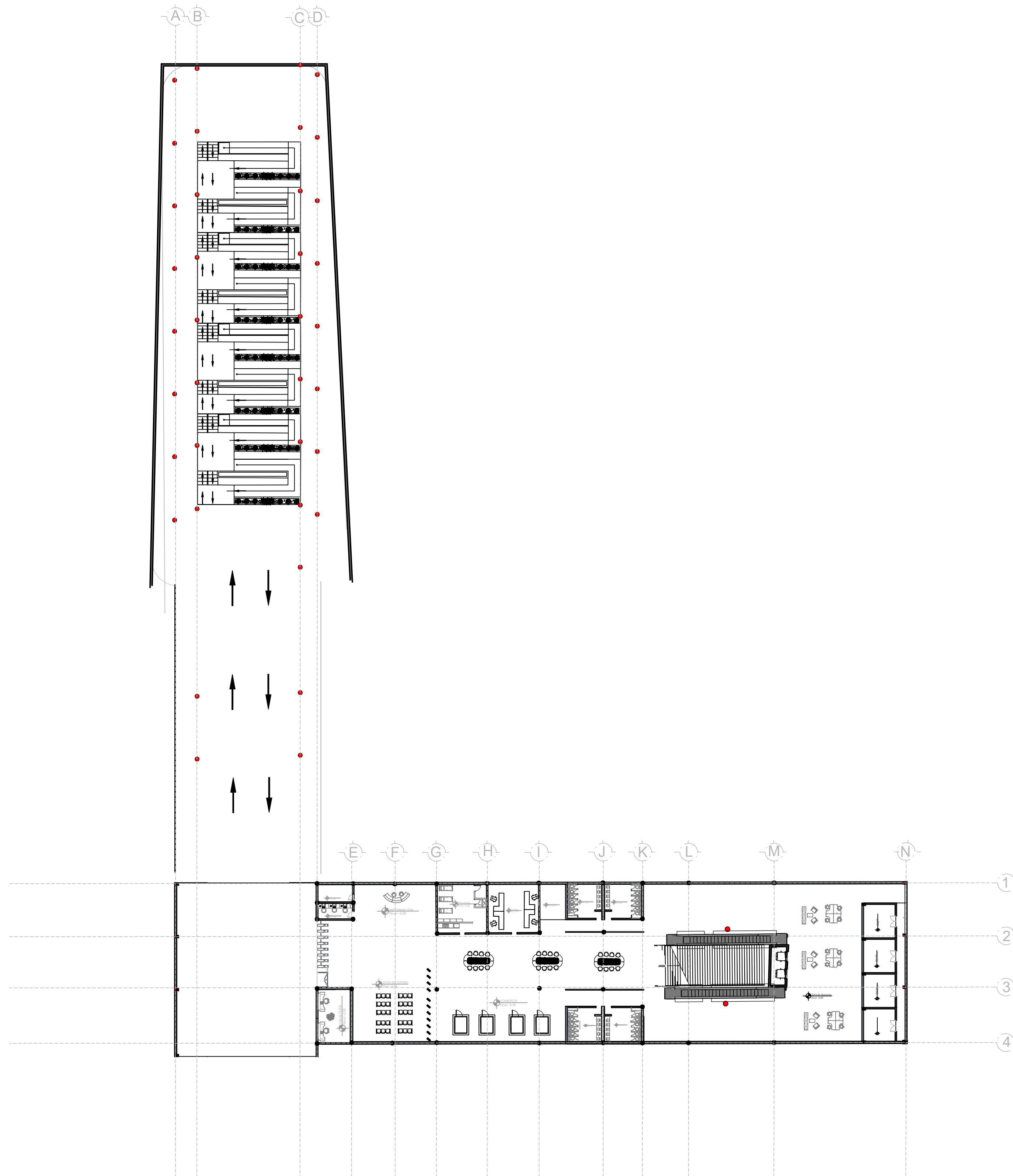
P1 PLANTA NIVEL - 6.00 VOLUMEN 1 ESC 1:250
