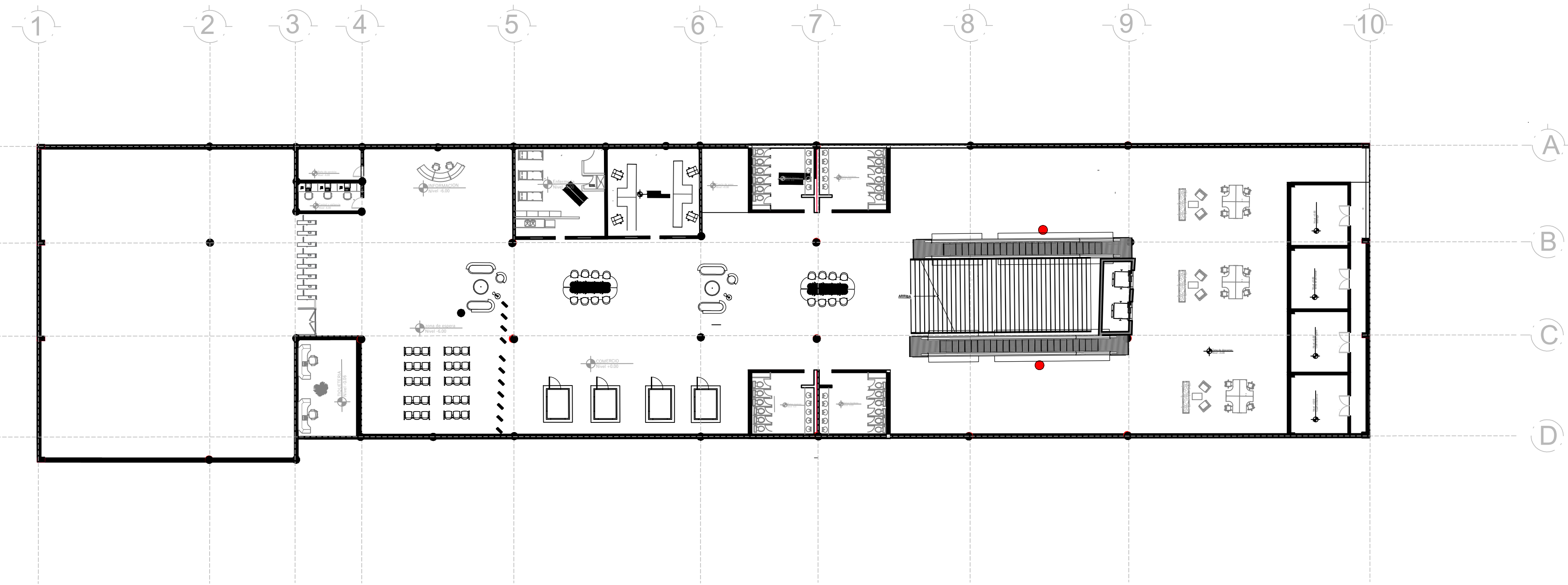
P1 PLANTA NIVEL - 6.00 VOLUMEN 1 ESC 1:250
