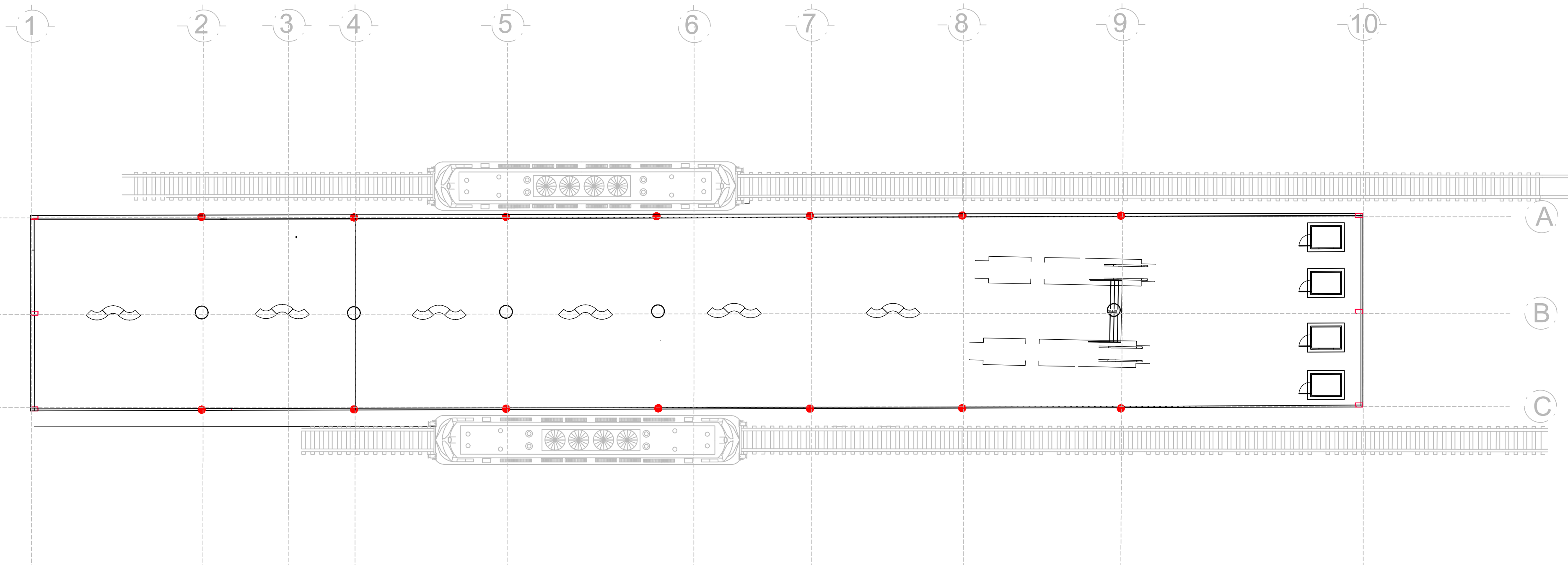
P2 PLANTA NIVEL 0.00 VOLUMEN 1 ESC 1:250
