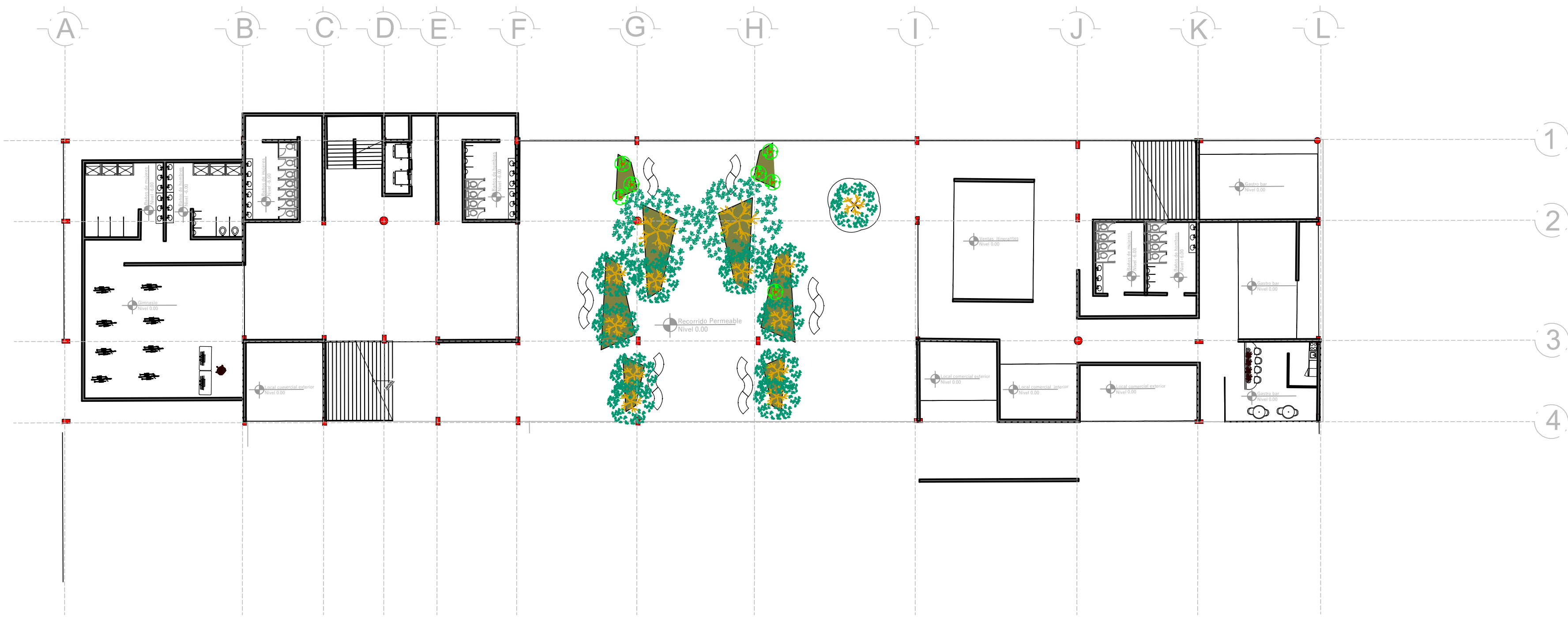
P1 PLANTA NIVEL 0.00 VOLUMEN 2 ESC 1:250
