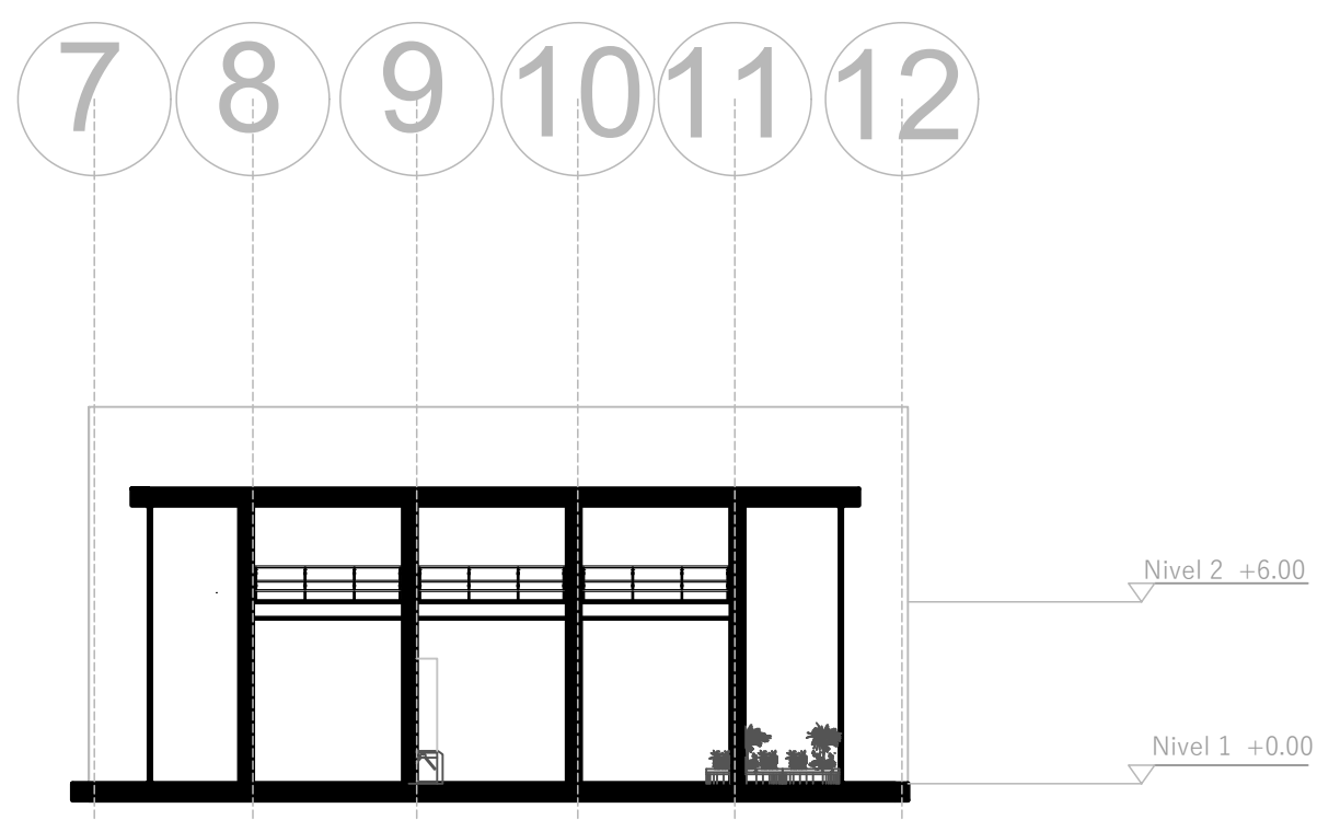
C1 CORTE VOLUMEN 2 ESC 1:250
