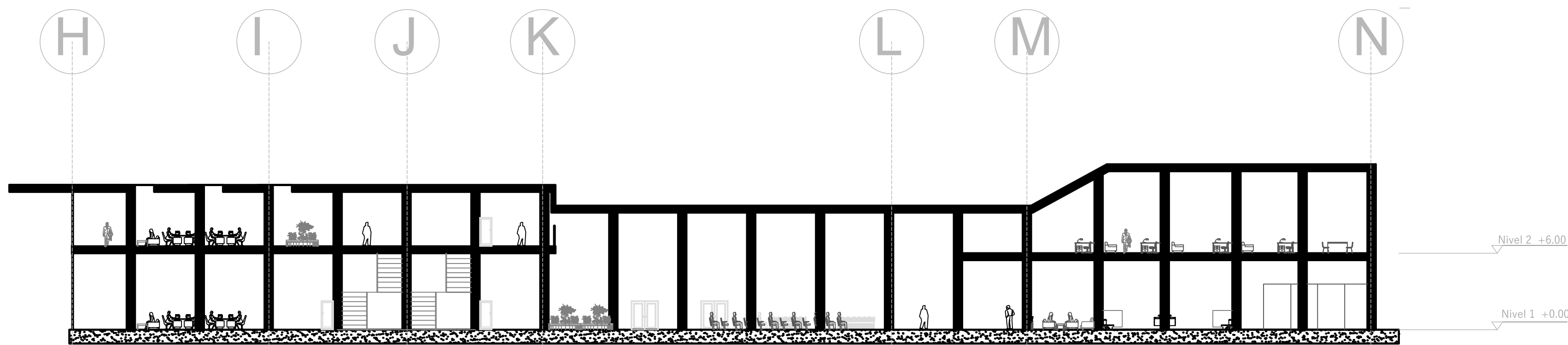
C2 CORTE VOLUMEN 2 ESC 1:250
