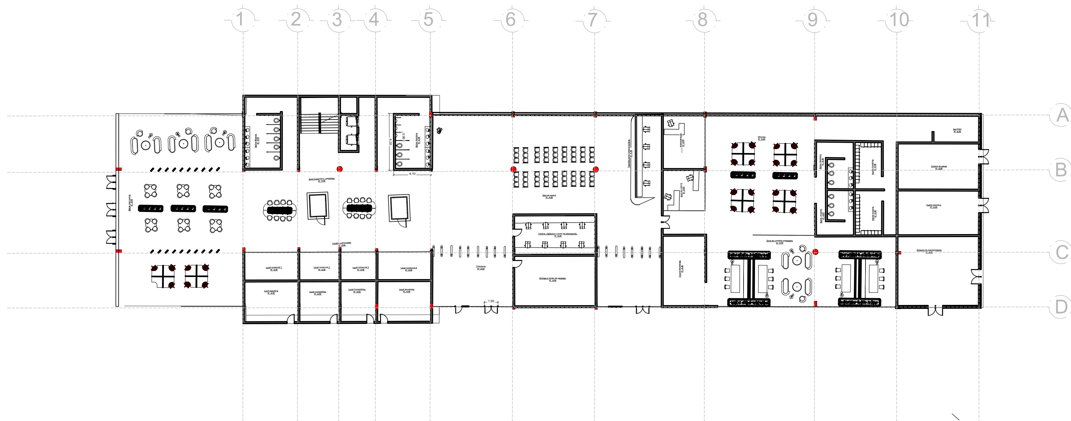
P1 PLANTA NIVEL - 6.00 VOLUMEN 2 ESC 1:250
