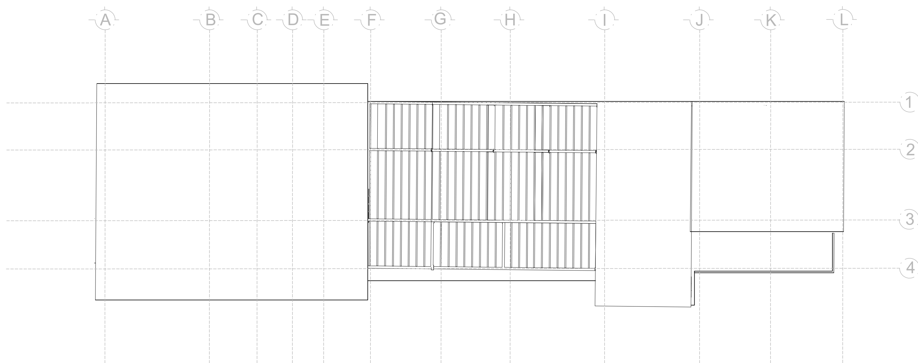
P1 PLANTA CUBIERTA VOLUMEN 1 ESC 1:250
