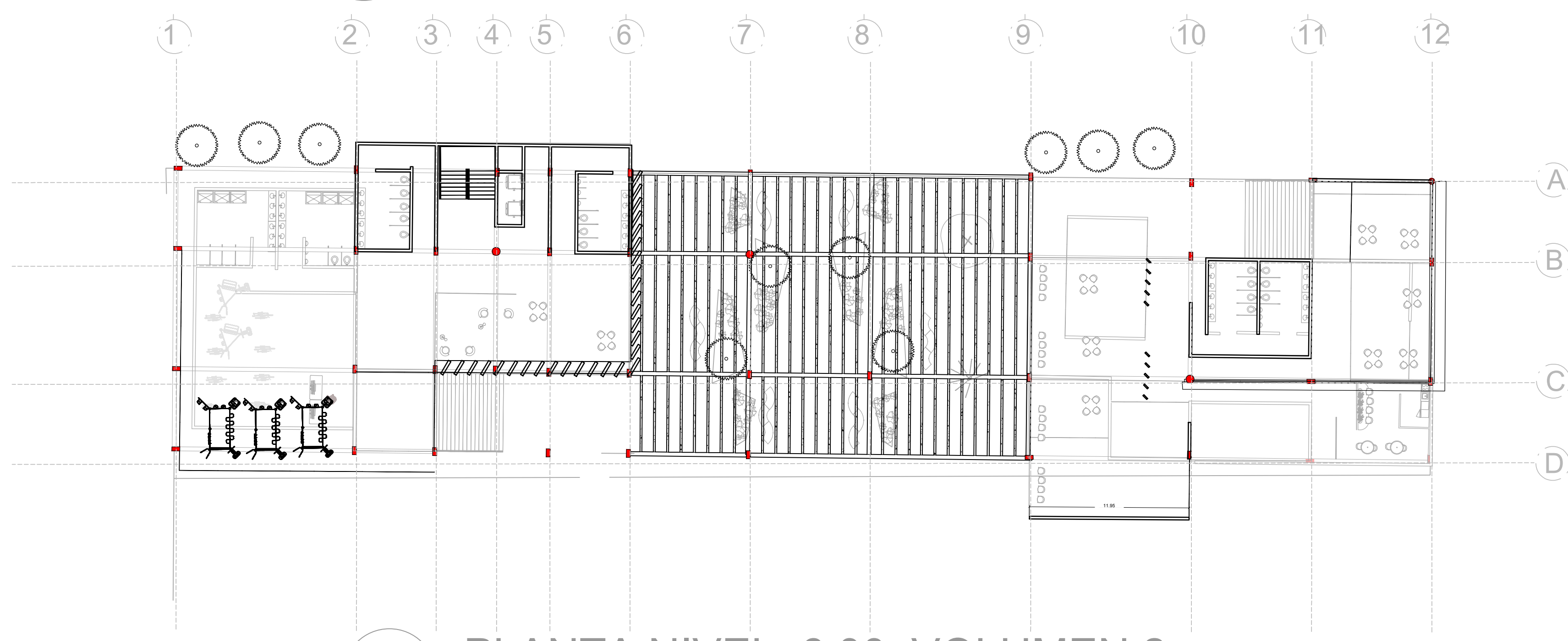
P1 PLANTA NIVEL 6.00 VOLUMEN 2 ESC 1:250
