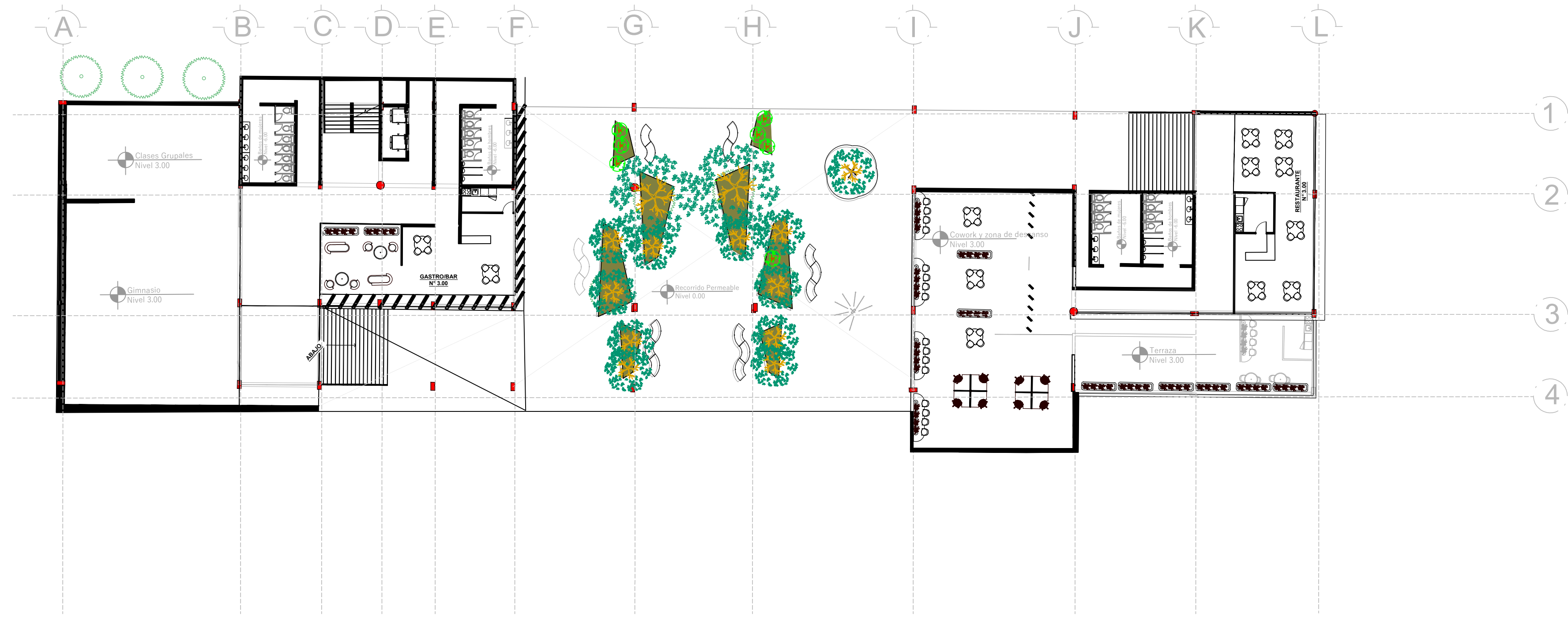
P1 PLANTA NIVEL 3.00 VOLUMEN 2 ESC 1:250
