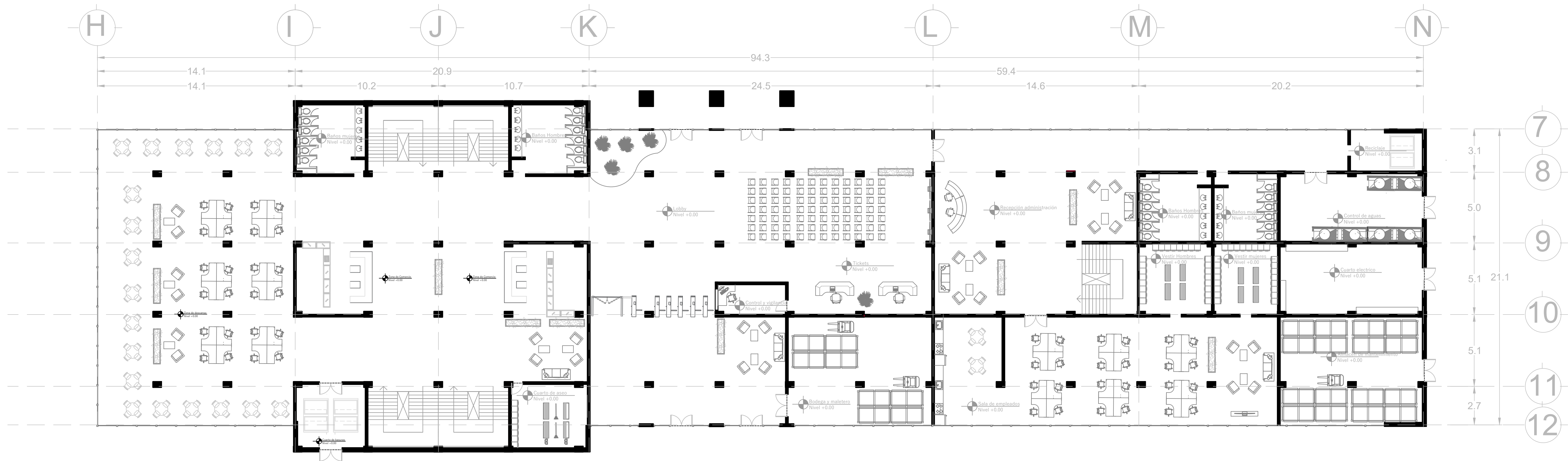
P2 PLANTA NIVEL 1 VOLUMEN 2 ESC 1:150
