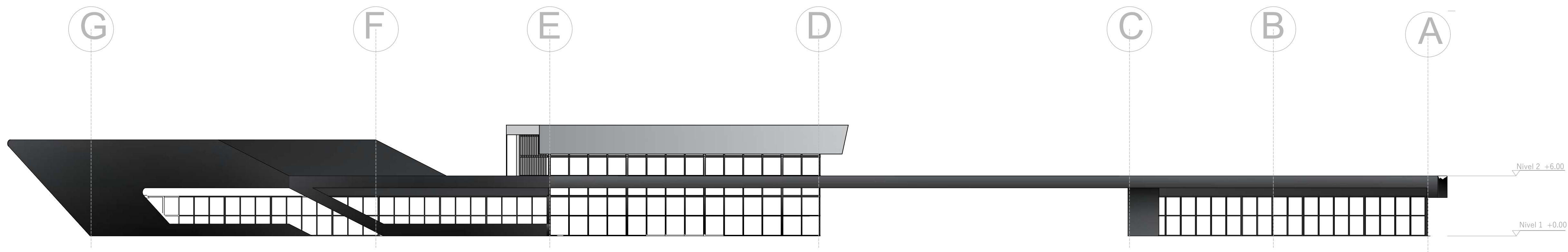
F1 FACHADA FRONTAL VOLUMEN 1 ESC 1:250
