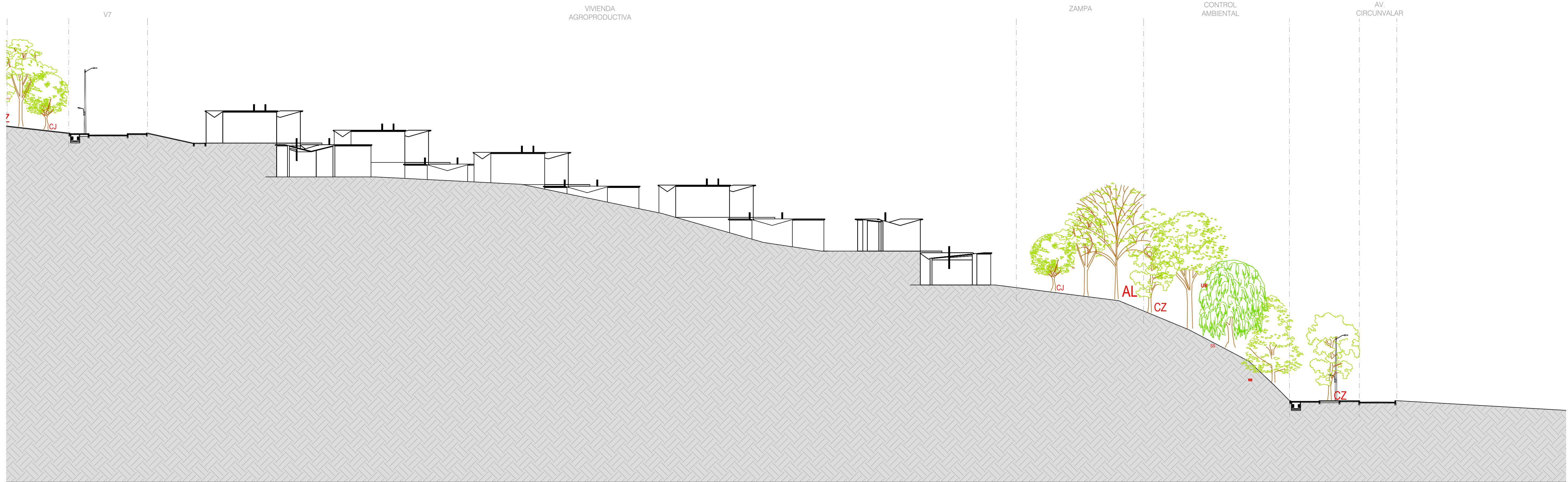
D4 AMPLIACION CORTE B - B1 ESCALA 1:350
