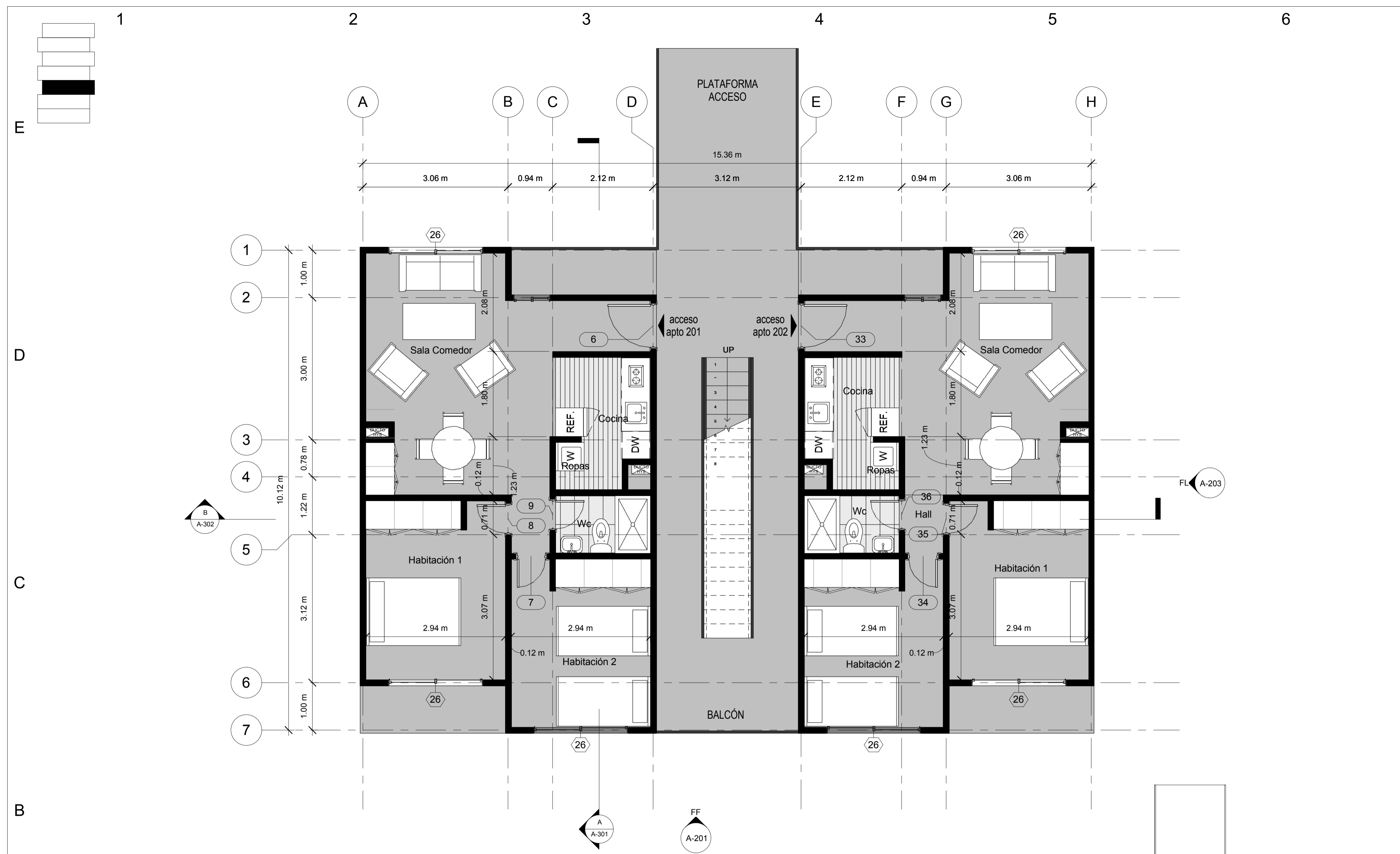
1 Planta 2 Bloque 54 1 : 50
