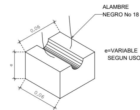
DETALLE DISTANCIADOR EN FORMA DE PANELA (EN CONCRETO) SIN ESCALA
