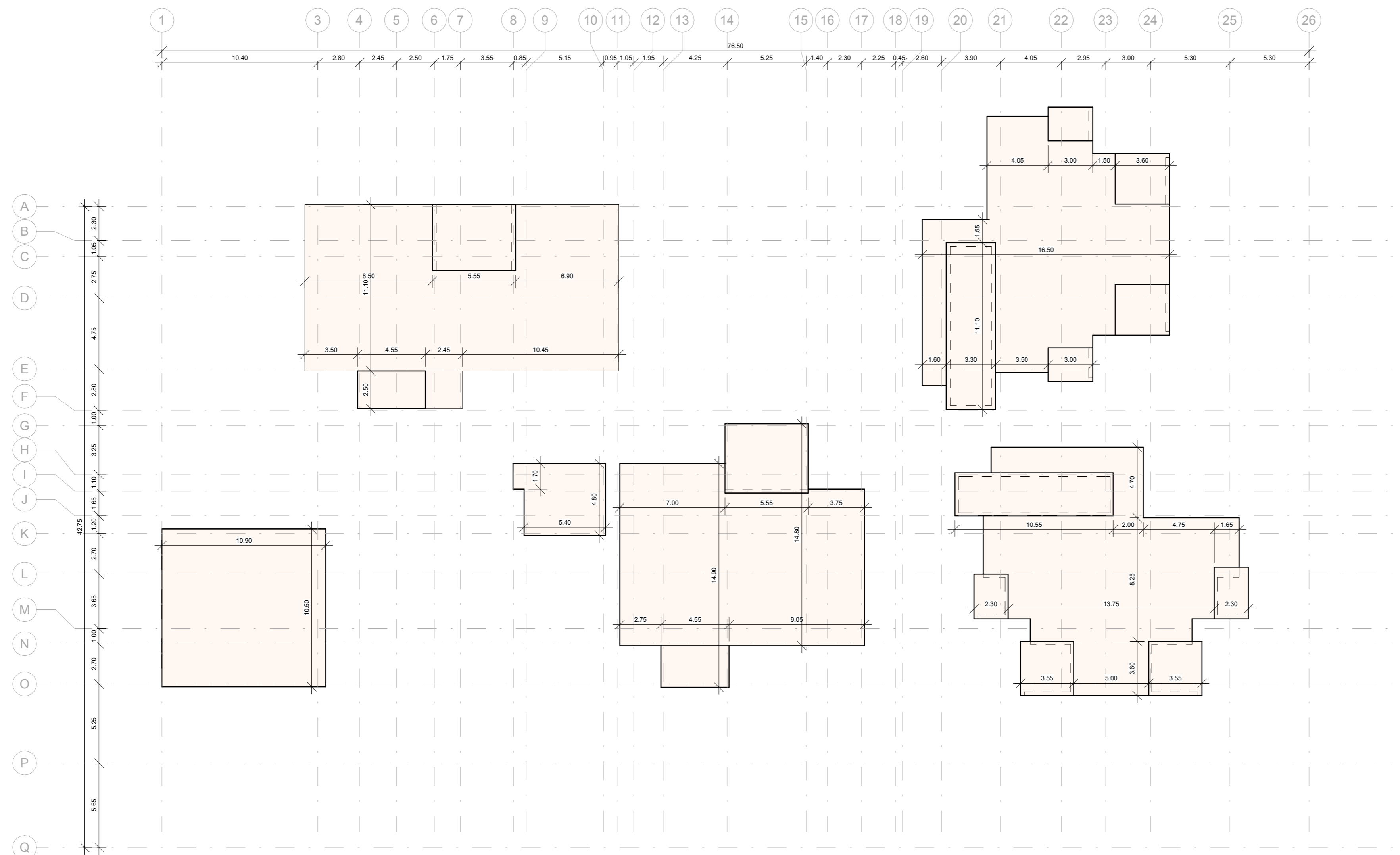
1 CUBIERTA - PLACAS CLT 1 : 200
