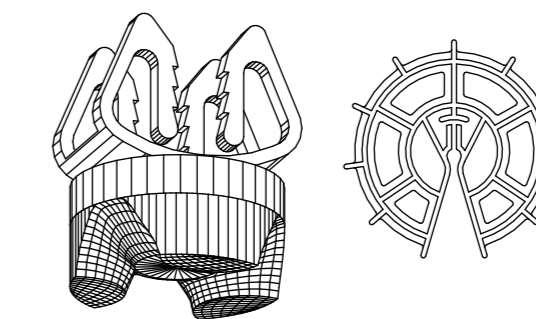
DETALLE DISTANCIADOR EN CONCRETO Y PLÁSTICO SIN ESCALA
