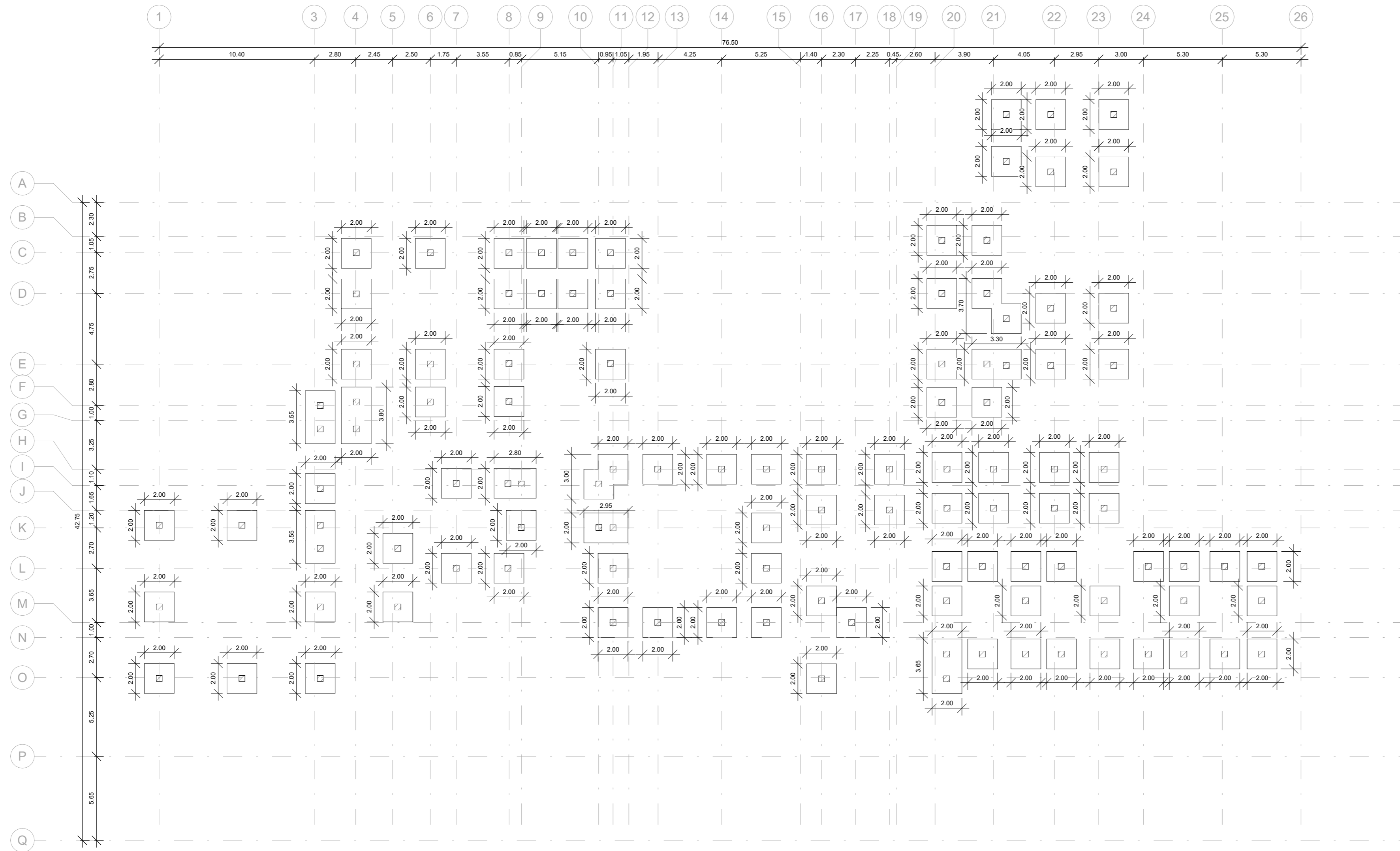
1 LEVEL 0 - LOCALIZACIÓN DE ZAPATAS 1 : 200
