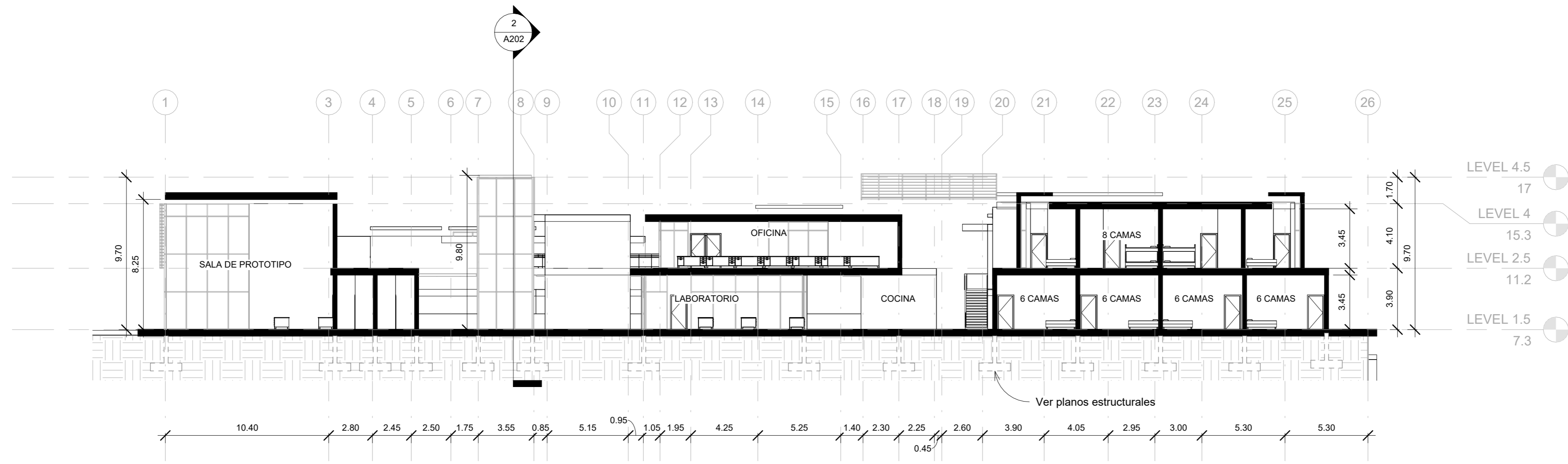
1 SECCIÓN A-A' 1 : 200
