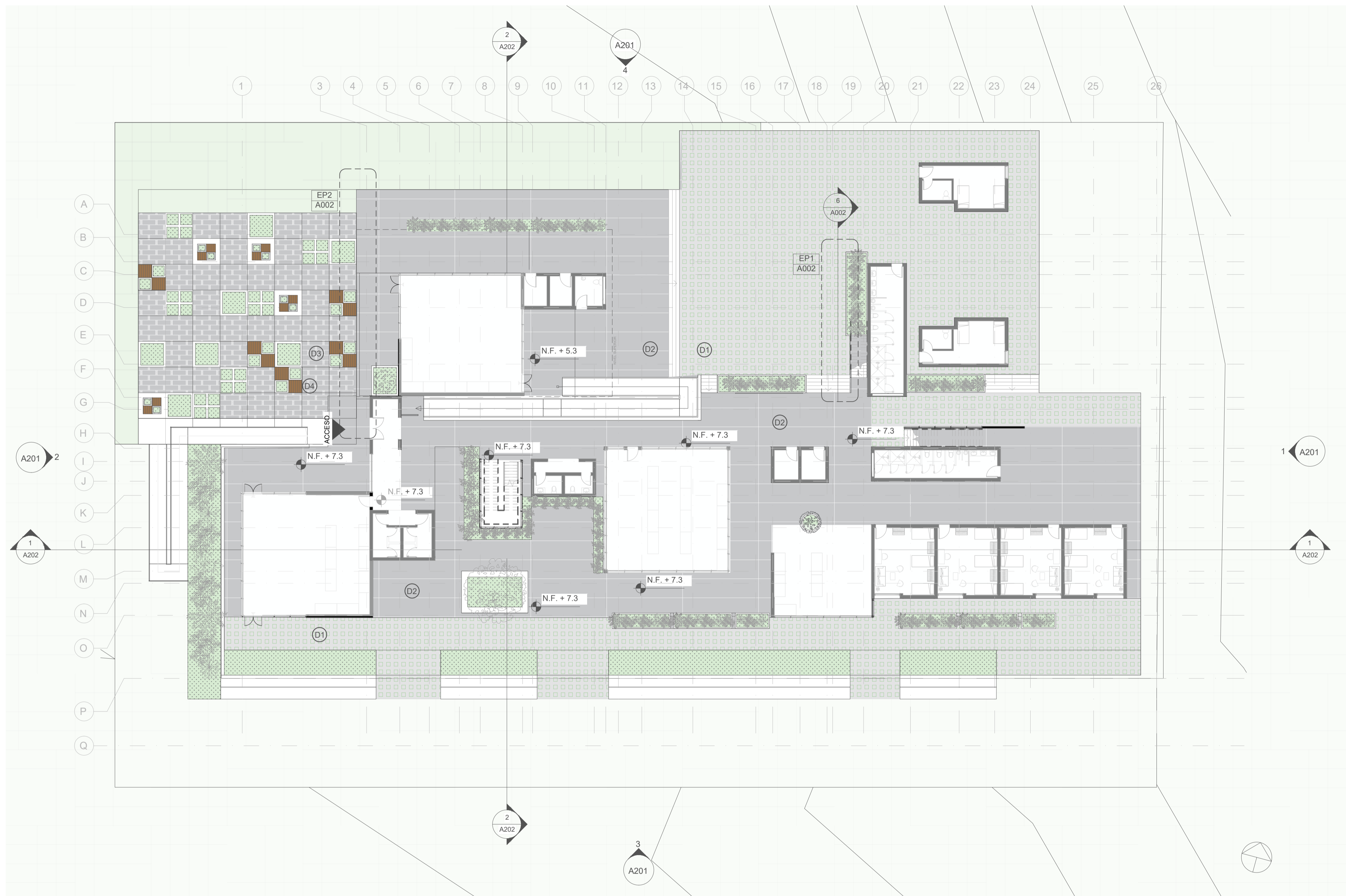
1 IMPLANTACIÓN Y ESPACIO PÚBLICO 1 : 200
