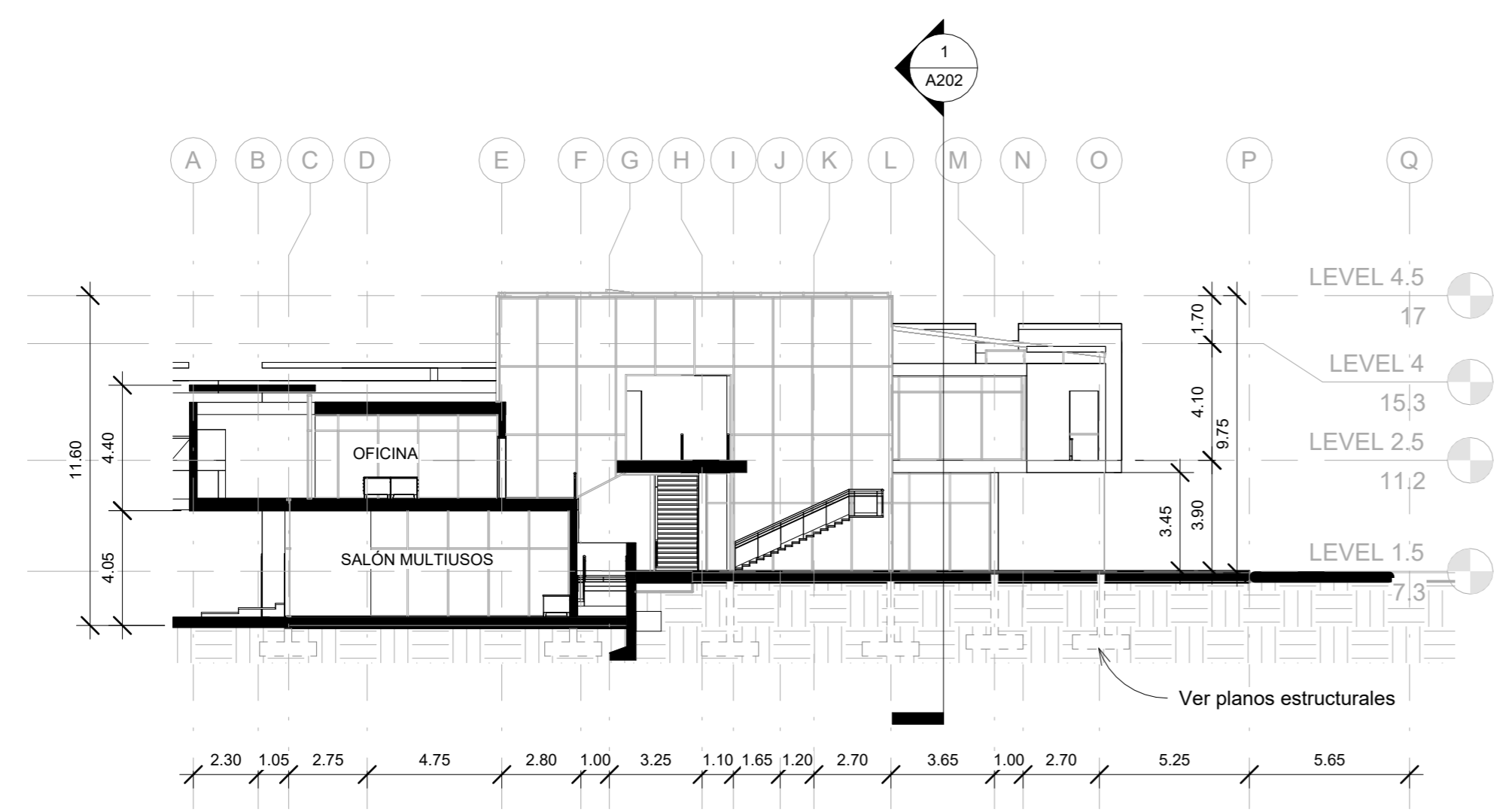
2 SECCIÓN B-B' 1 : 200
