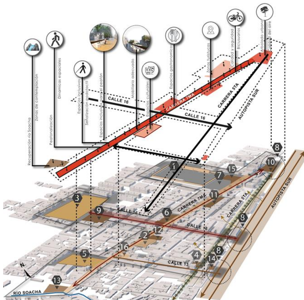
Figura 26. Propuesta conexión nodal. Elaboración propia.
