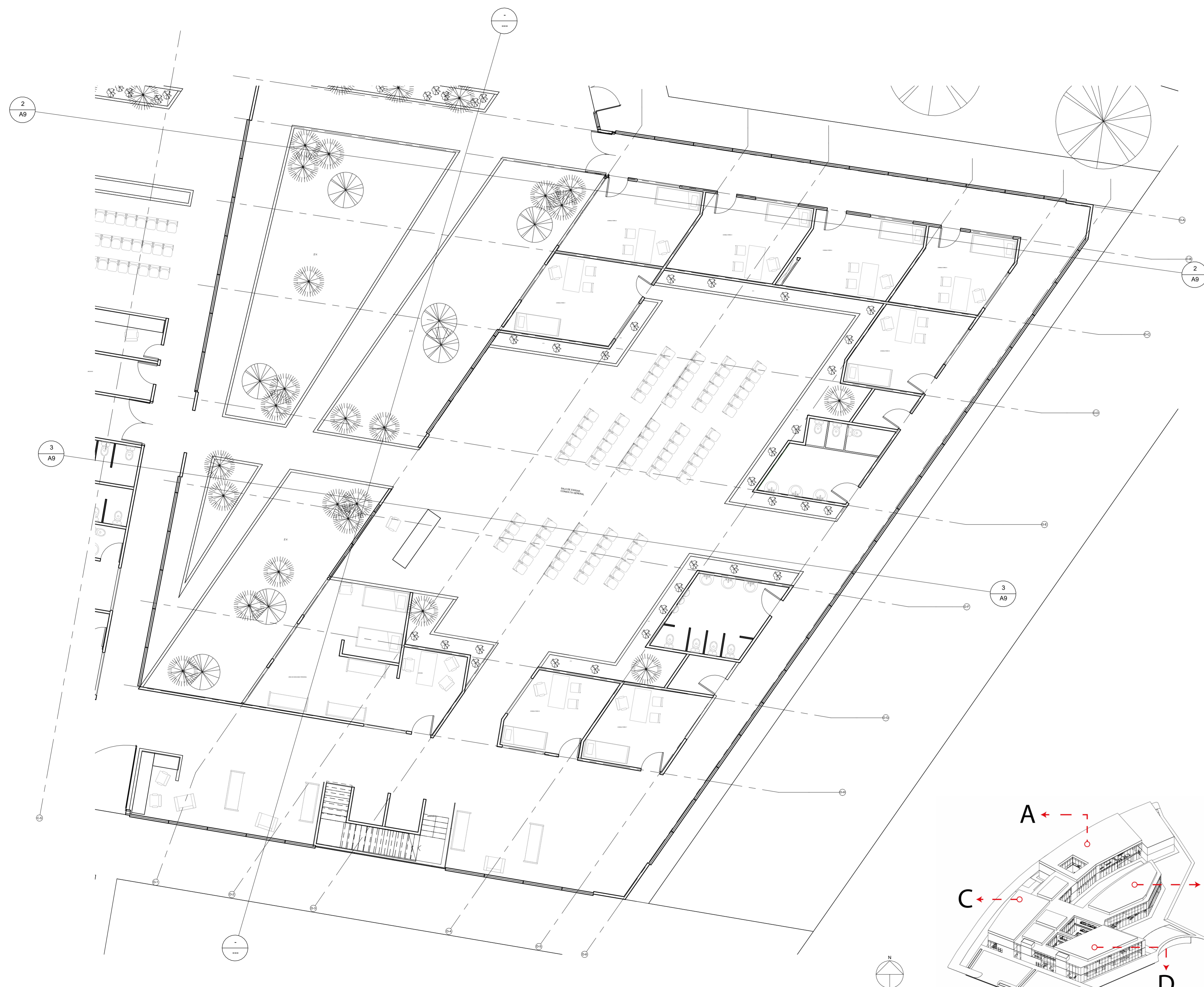
3 PISO 1 BLOQUE D 1:100
