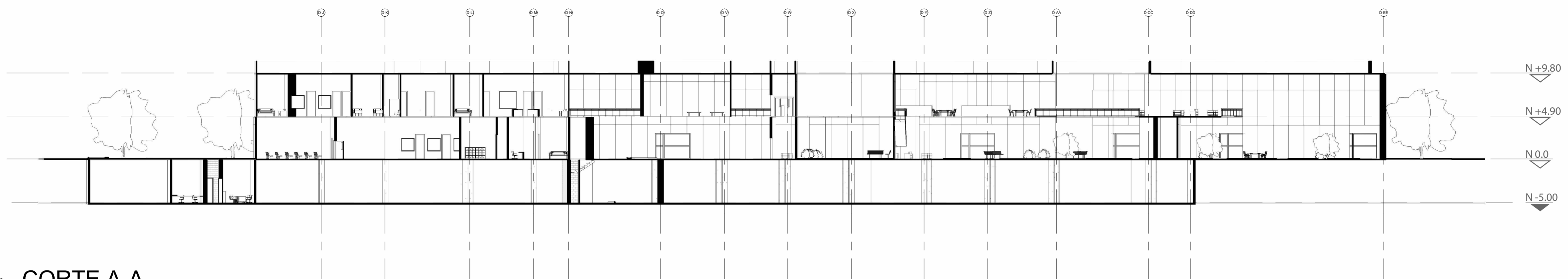
4 CORTE A-A 1 : 300
