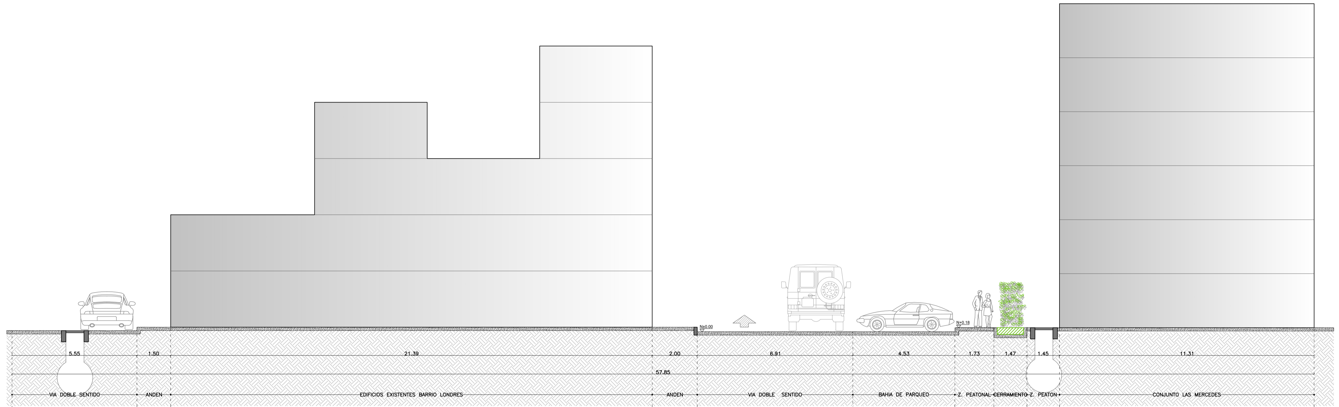
PERFIL URBANO ACTUAL SOBRE BARRIO LONDRES ESC_____1:100
