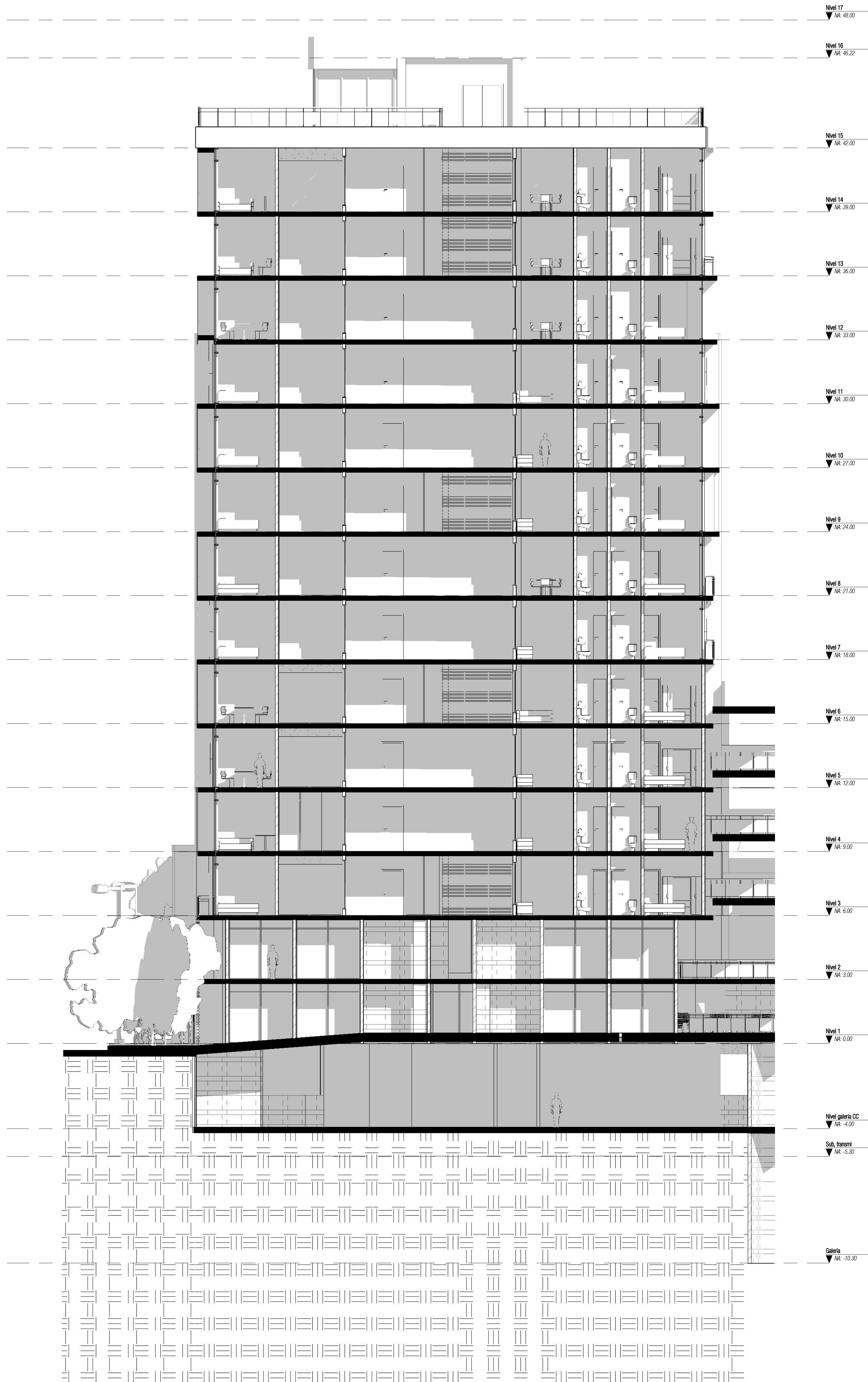
27 CORTE LONGITUDINAL B-B ESCALA: 1 : 100
