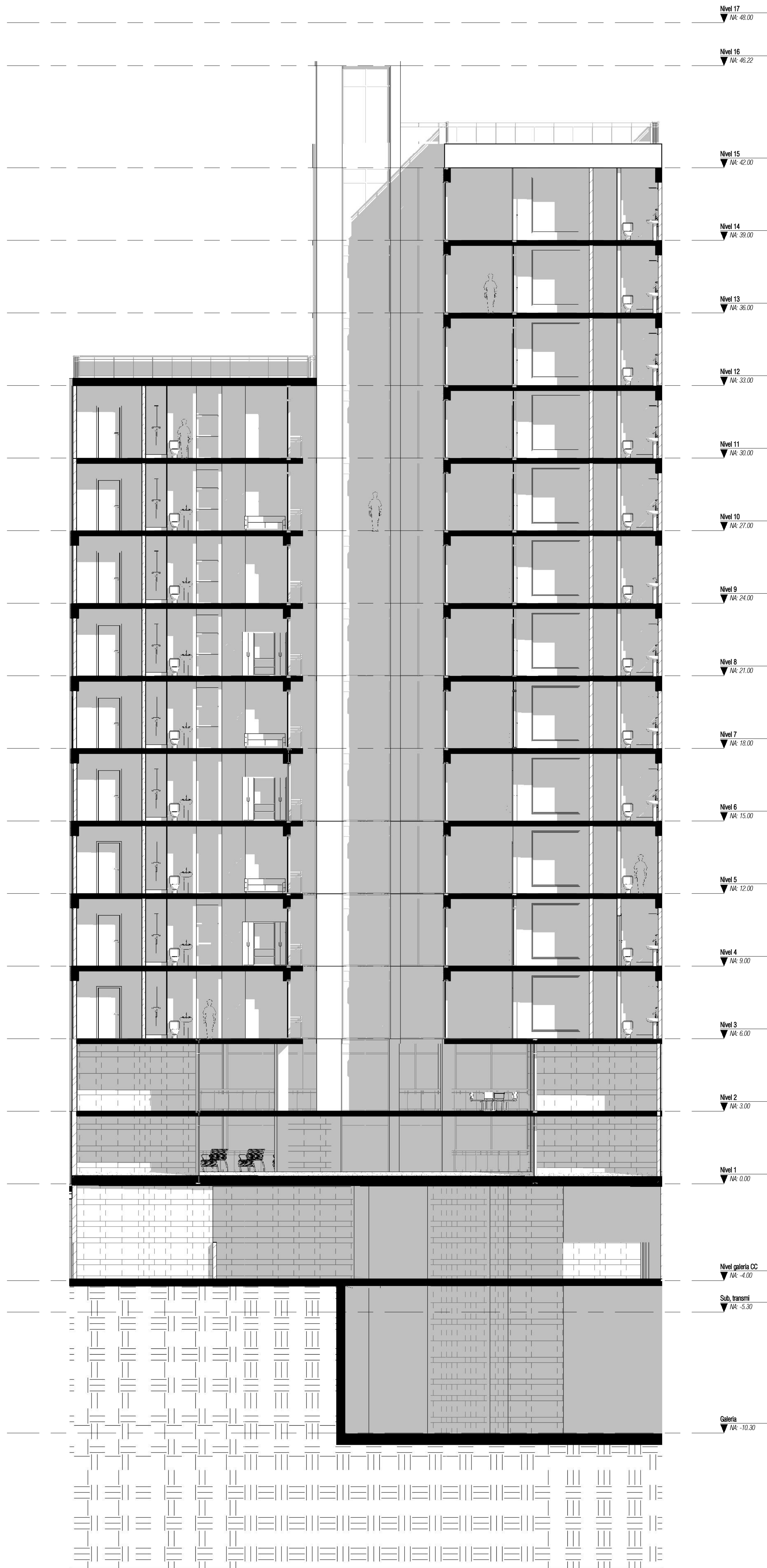
26 CORTE TRANSVERSAL A-A ESCALA: 1 : 100
