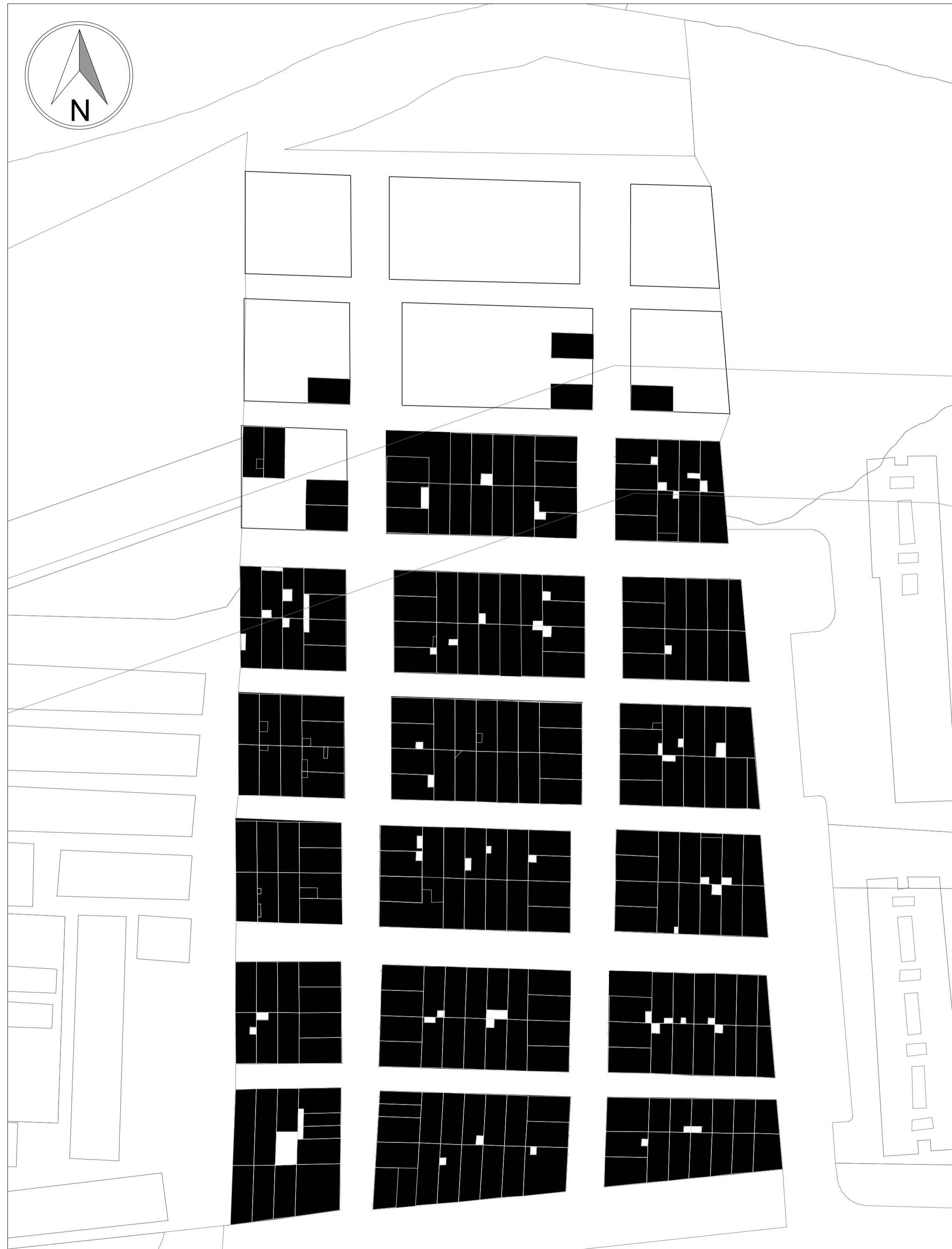
BARRIO LONDRES PLANO DE LLENOS Y VACÍOS ANTES DE INTERVENCIÓN
