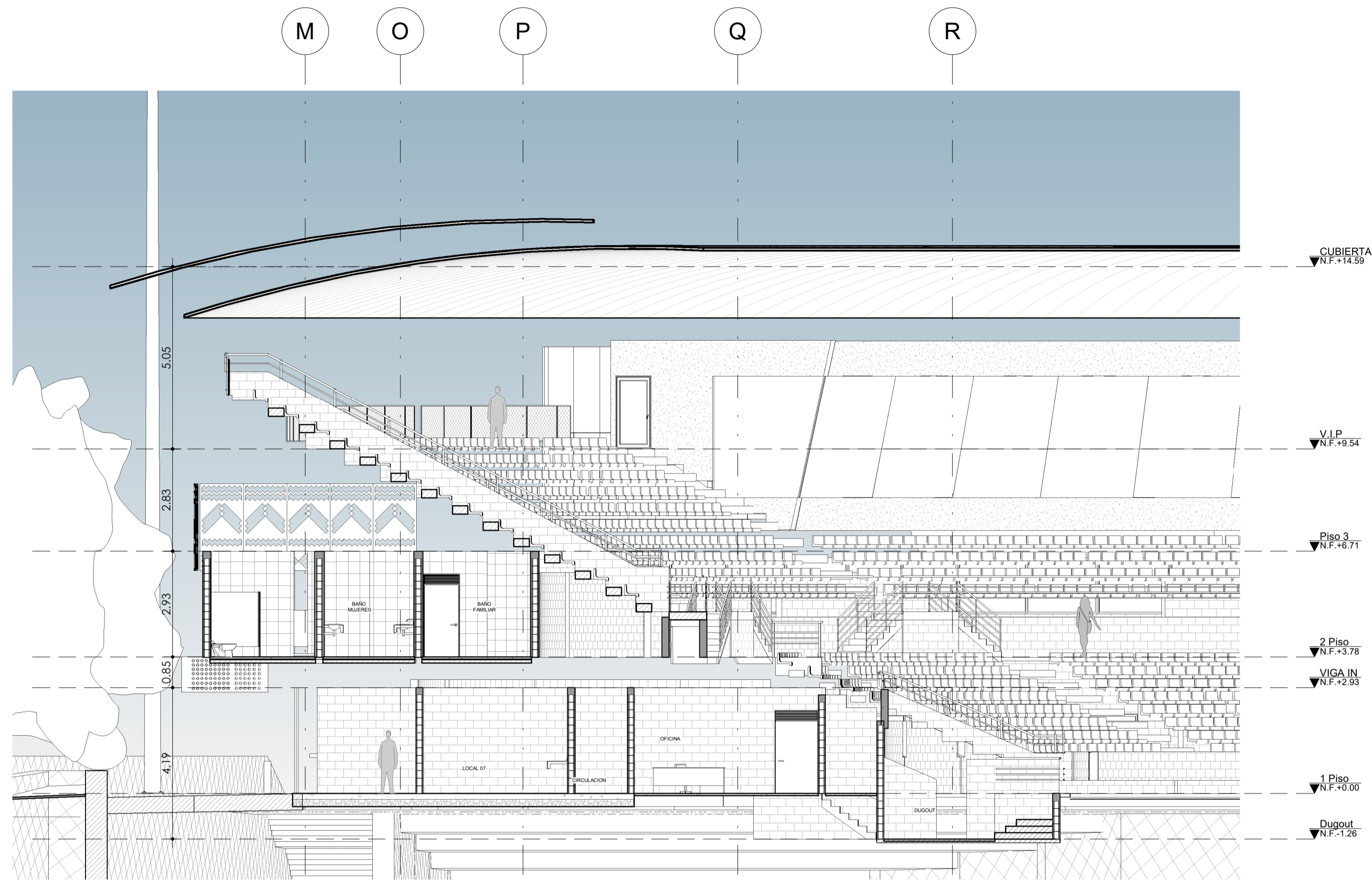
1 CORTE DUGOUT-02 1 : 100
