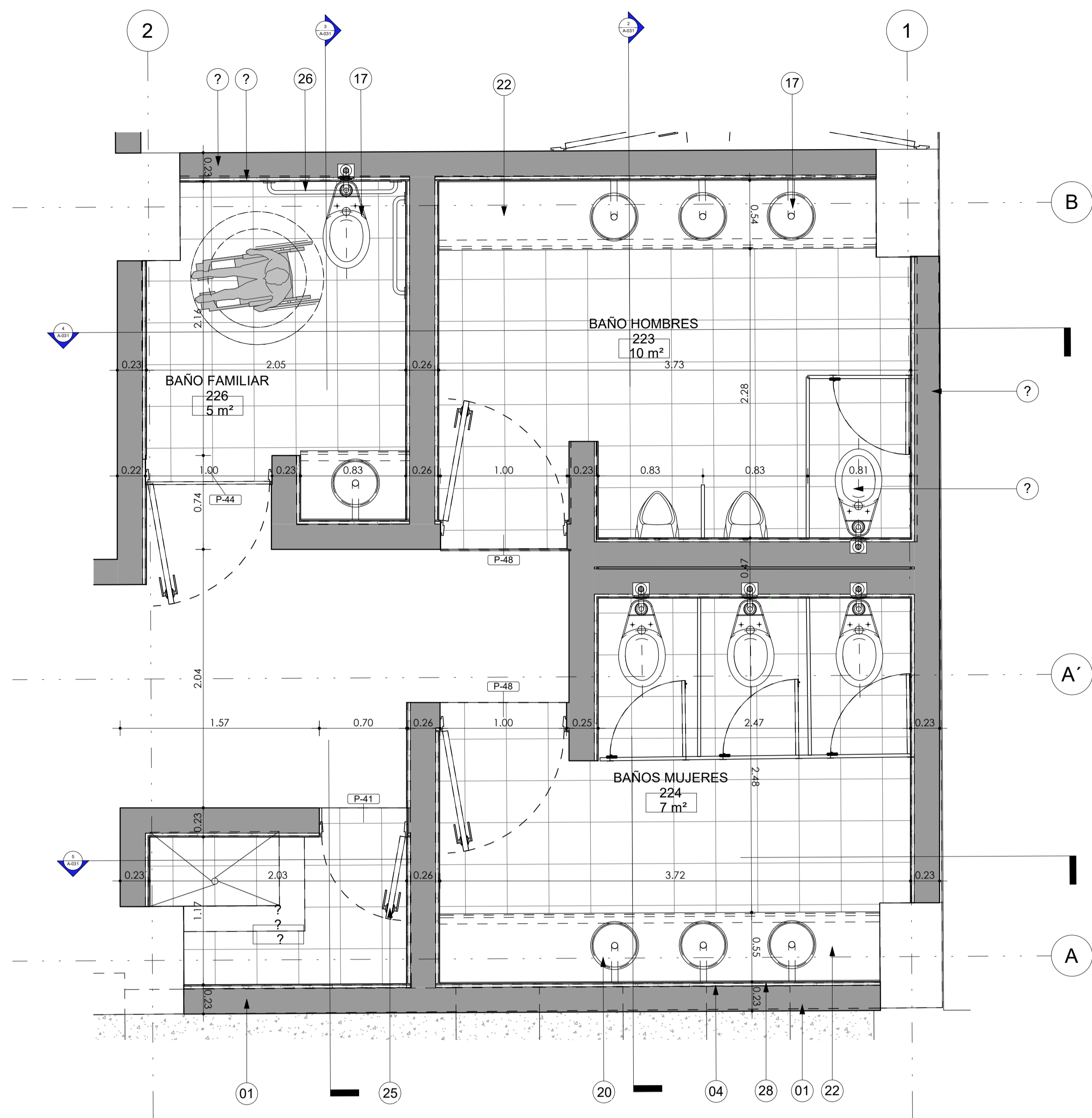
1 PLANTA BAÑO PUBLICO PRIMER PISO 1:25
