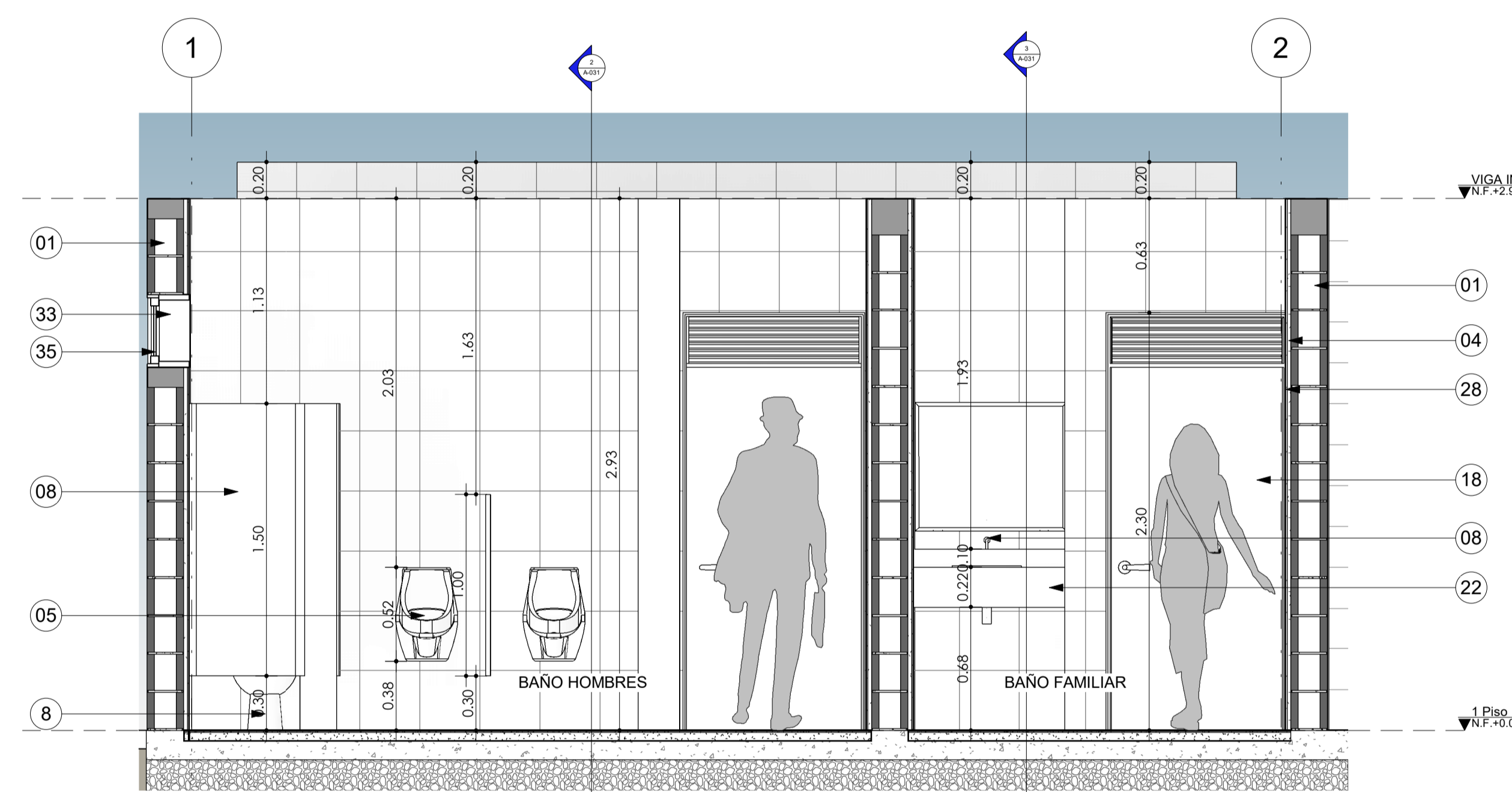
2 CORTE BAÑO PUBLICO A-A' 1:25
