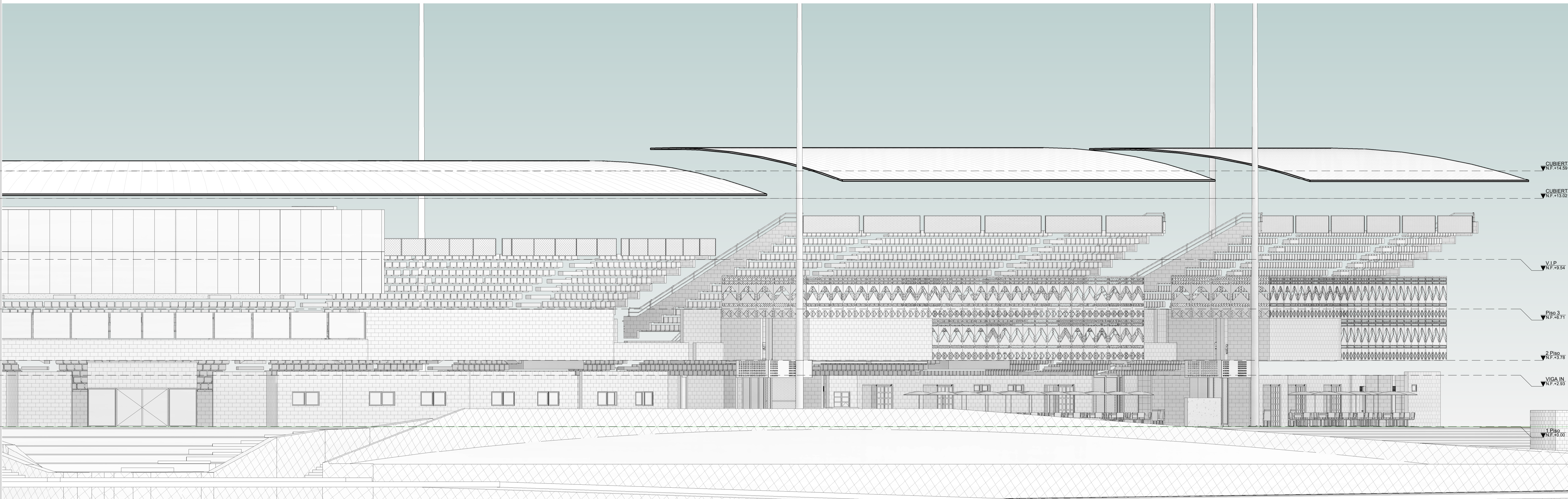
2 Oeste Seccion 2 1 : 100
