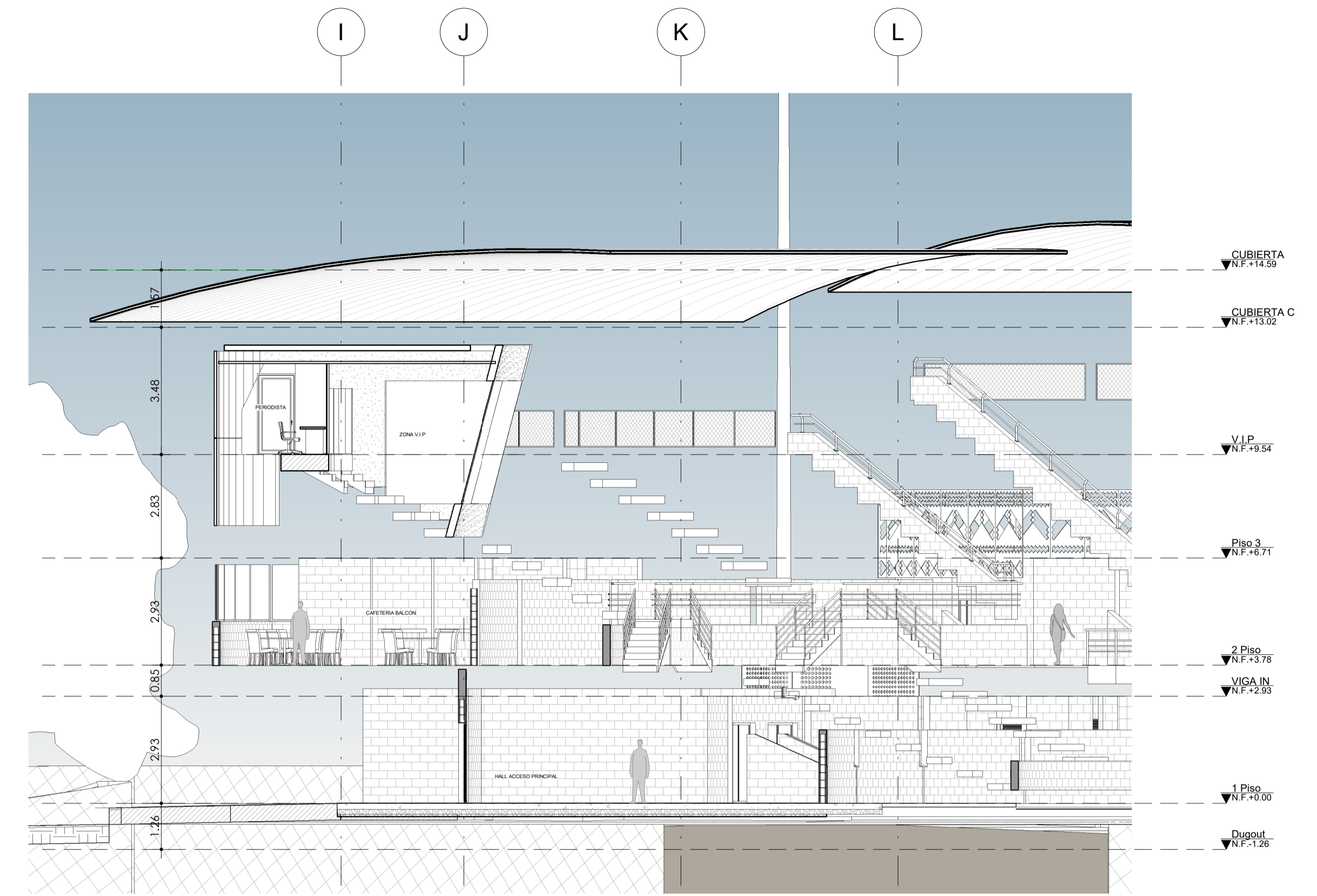
2 CORTE-ENTRADA PRINCIPAL 1 : 100
