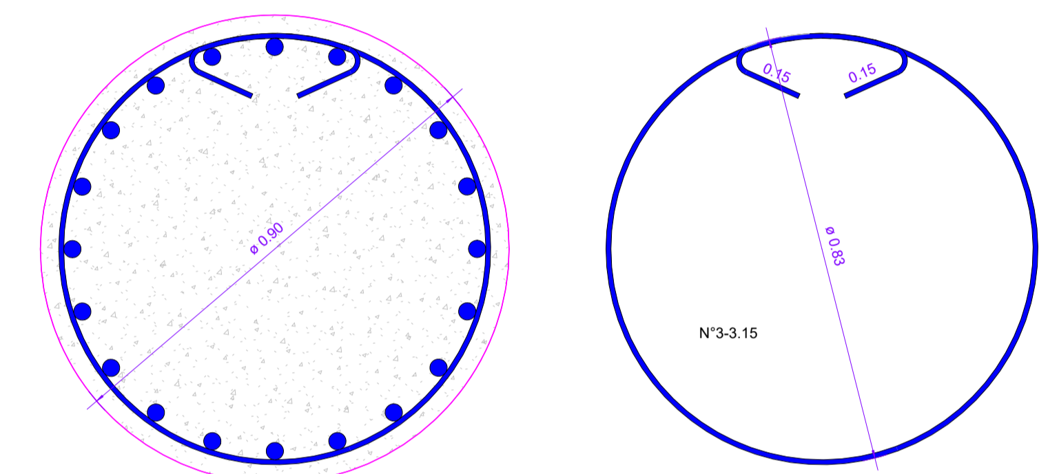
D2 C-0.90 1:10
