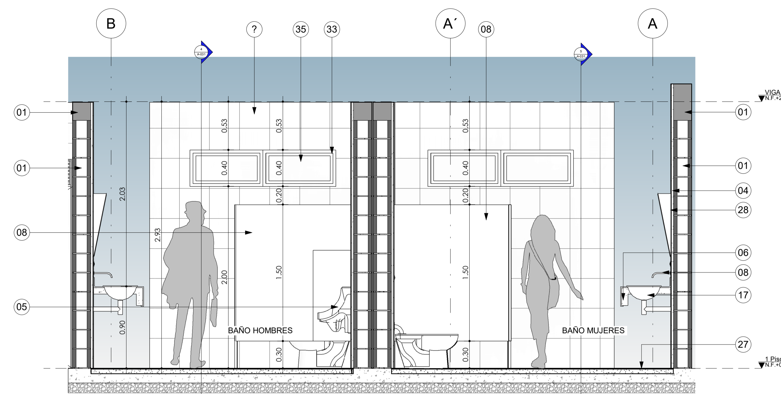
2 CORTE BAÑO PUBLICO A-A' 1:25
