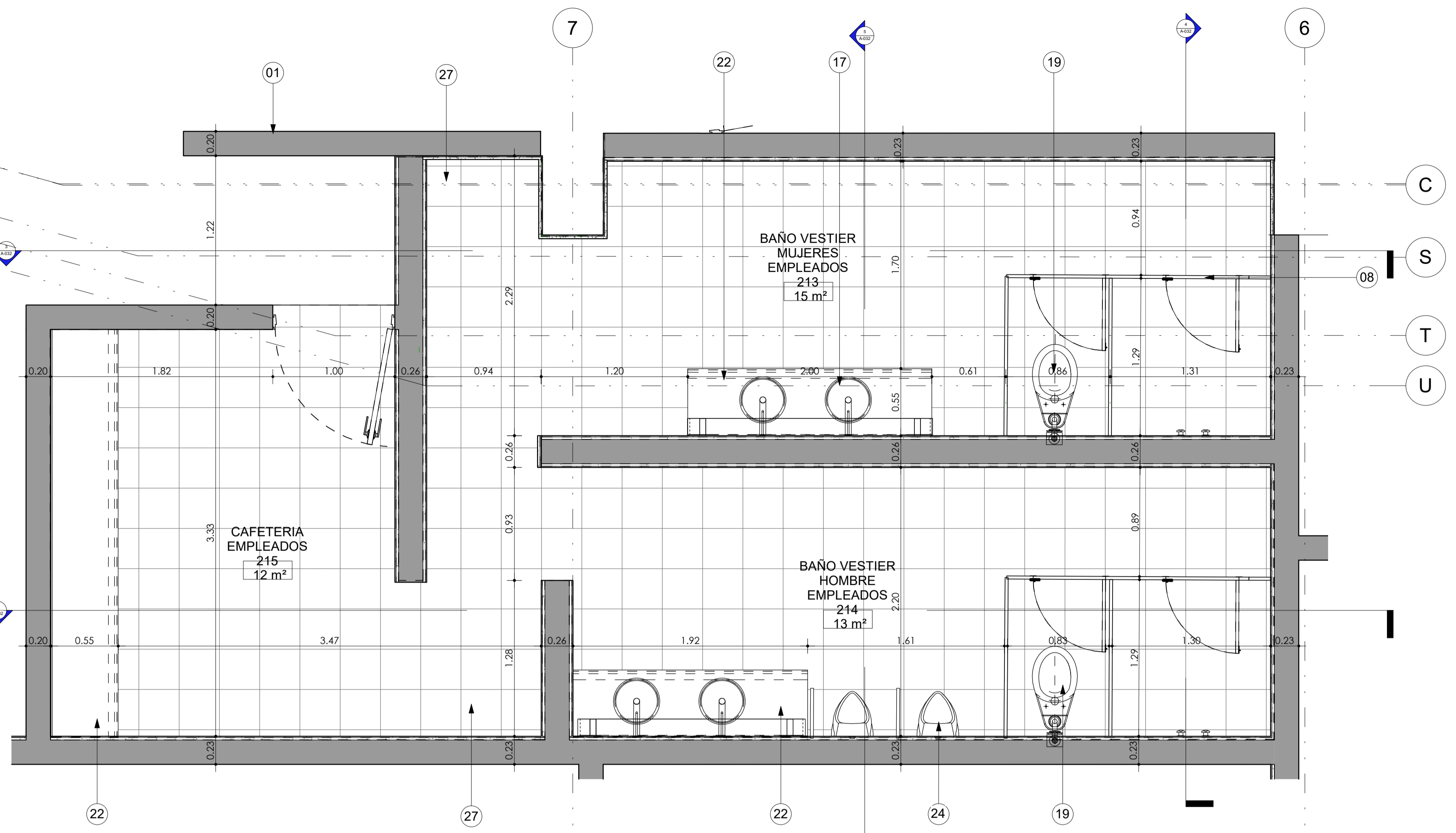
1 PLANTA BAÑOS VESTIER EMPLEADOS 1 : 25
