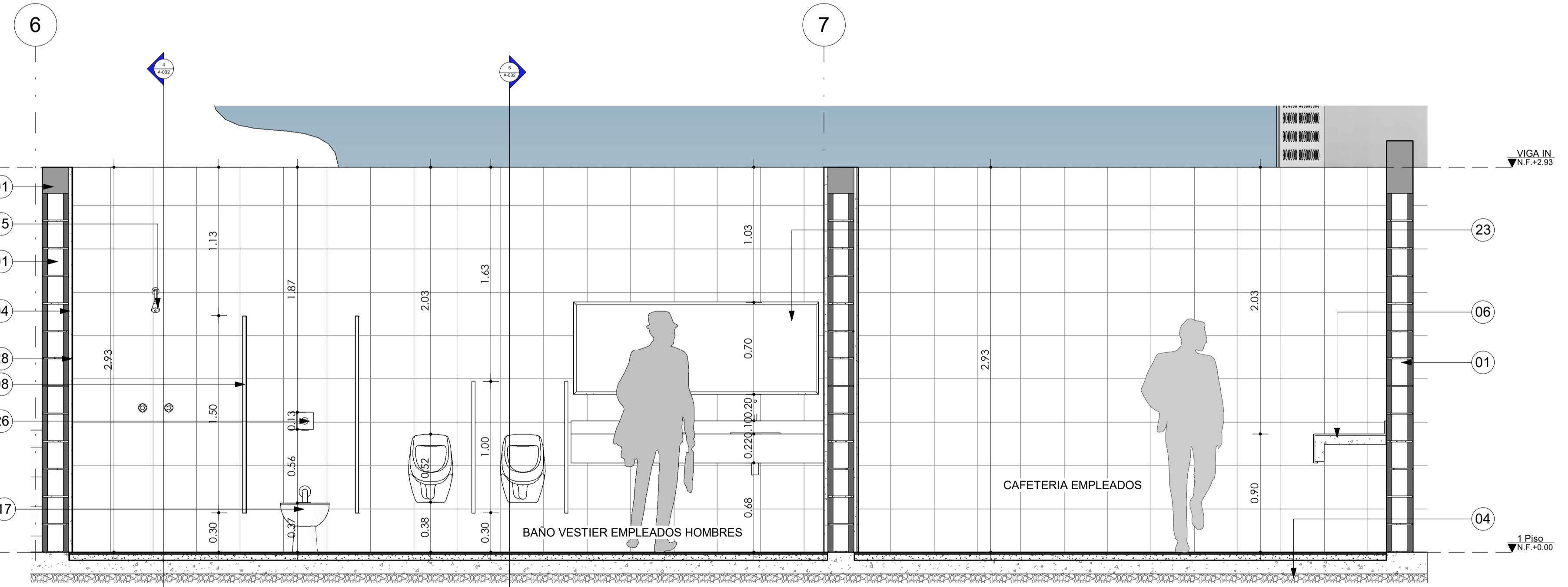
2 CORTE BAÑO VESTIER A-A' 1 : 25
