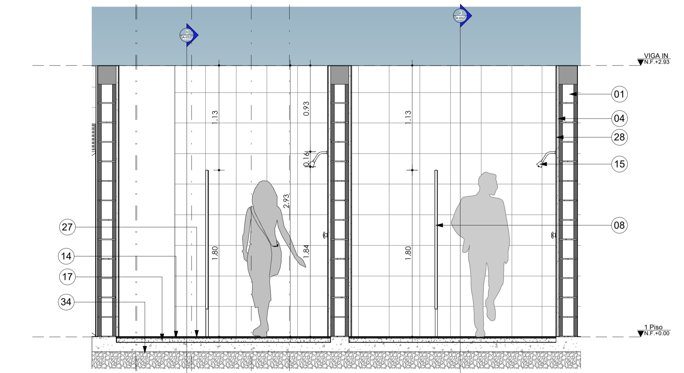
4 CORTE BAÑO VESTIER C-C' 1 : 25
