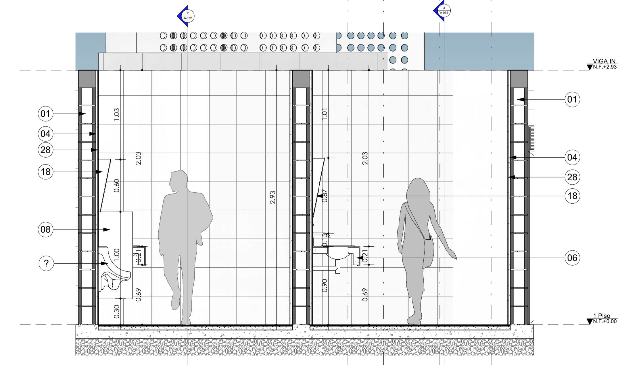
5 CORTE BAÑO VESTIER D-D' 1 : 25
