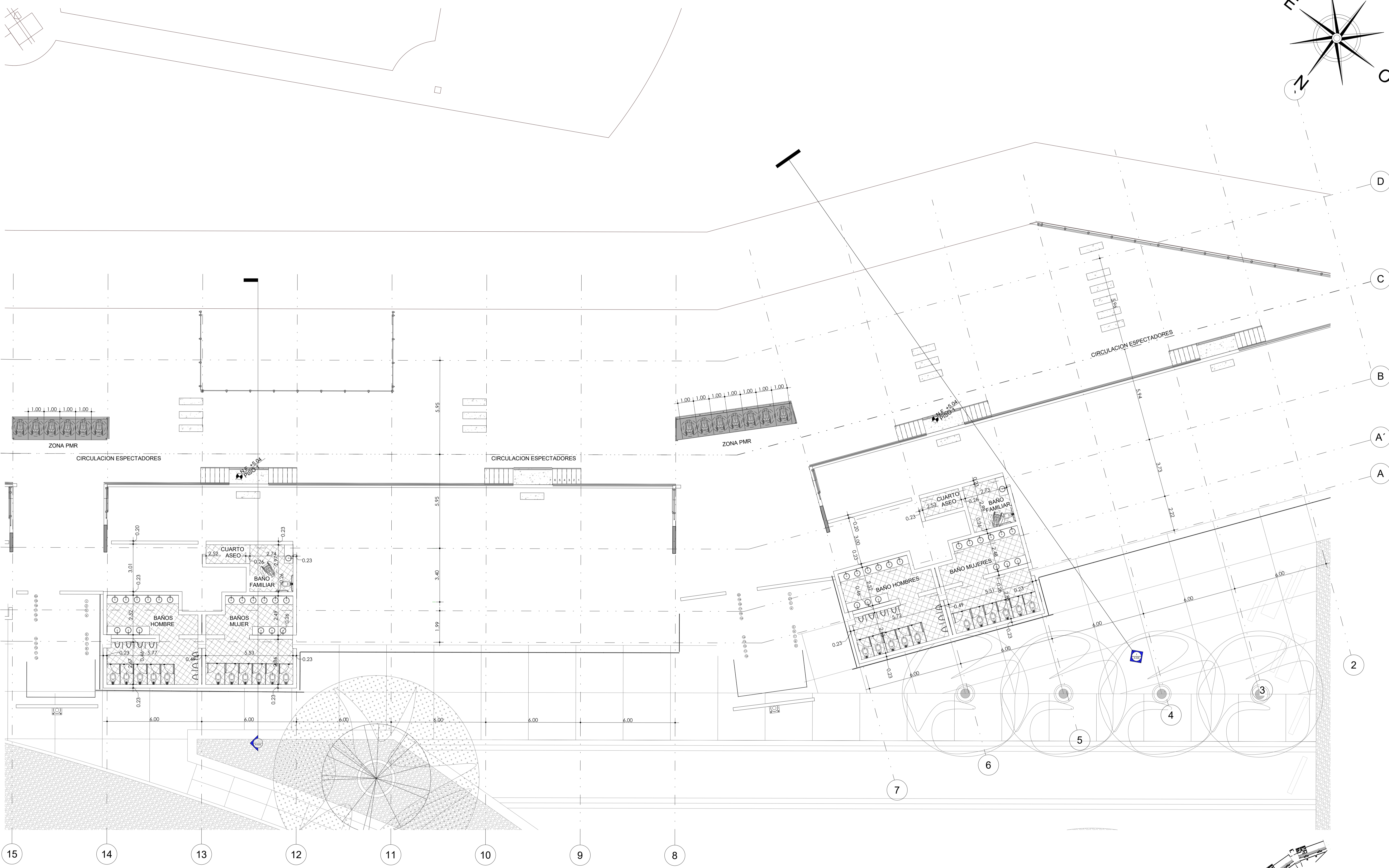
1 PLANTA SEGUNDO PISO SECCION 1 1 : 100
