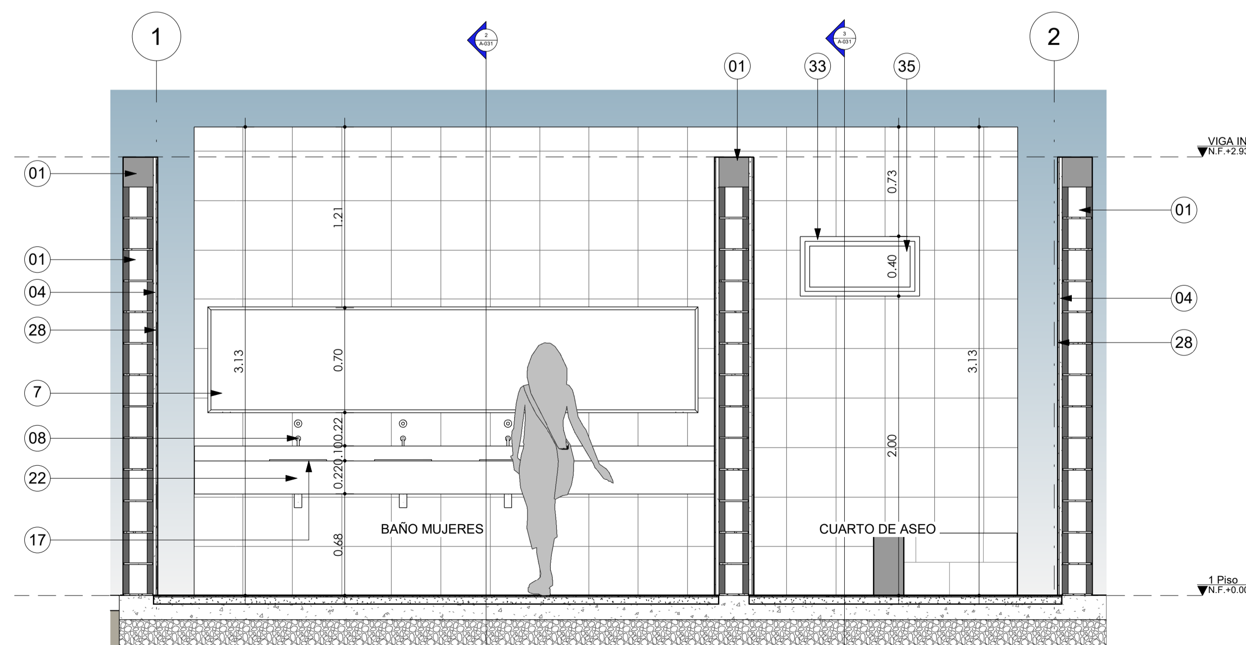
5 CORTE BAÑO PUBLICO D-D' 1:25
