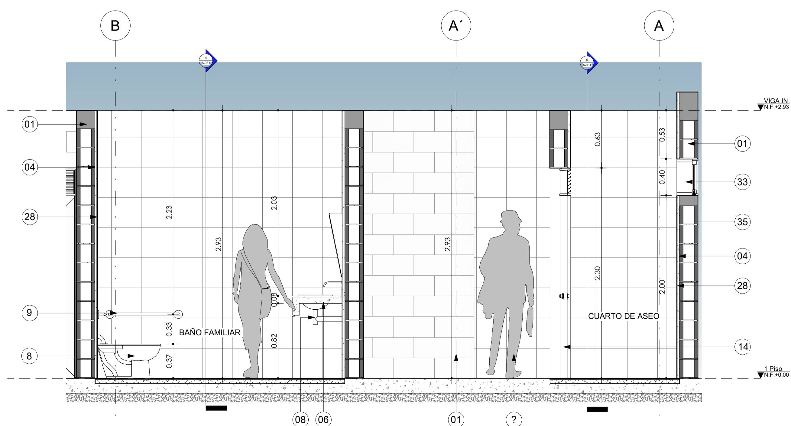
3 CORTE BAÑO PUBLICO B-B' 1:25
