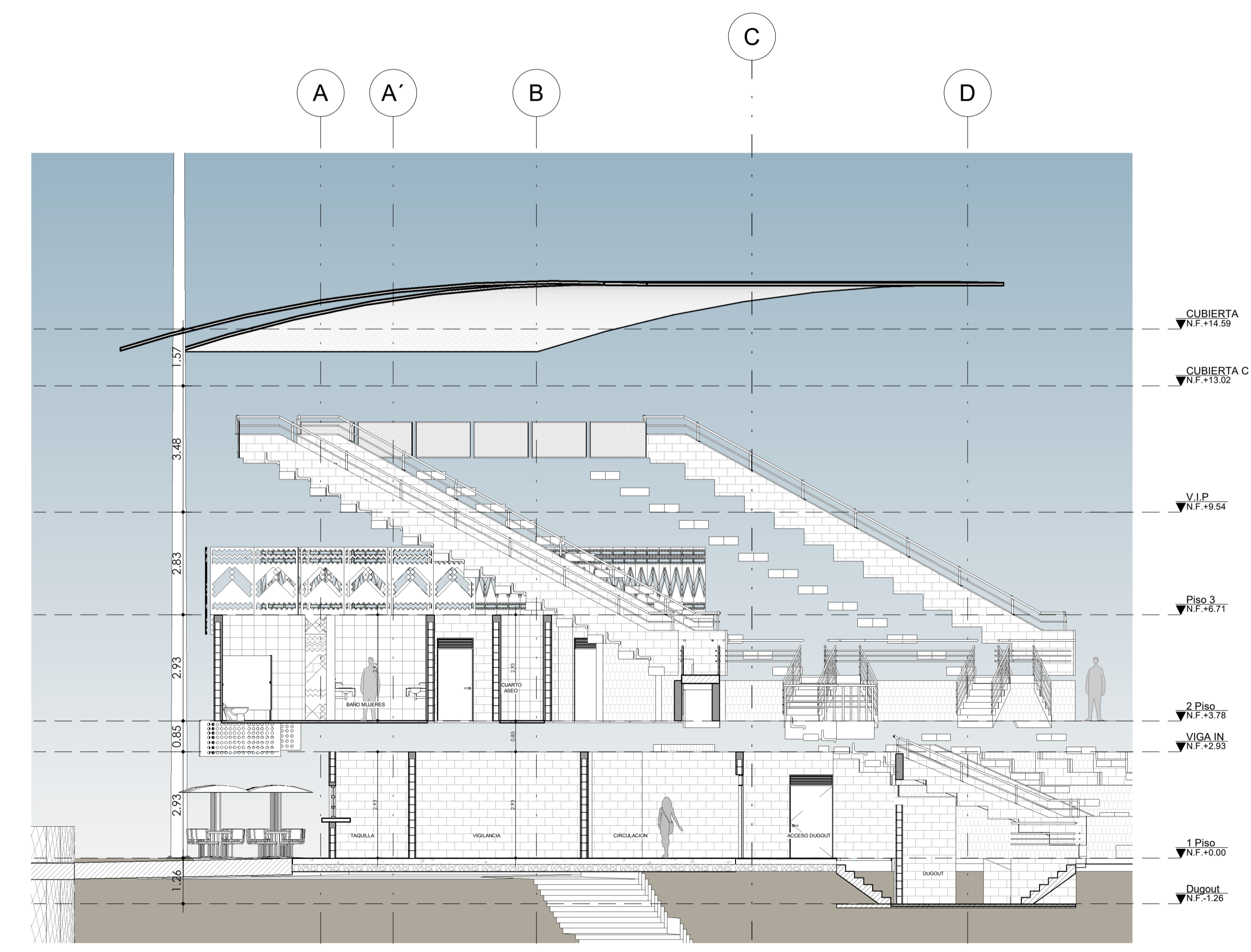
3 CORTE DUGOUT-01 1 : 100
