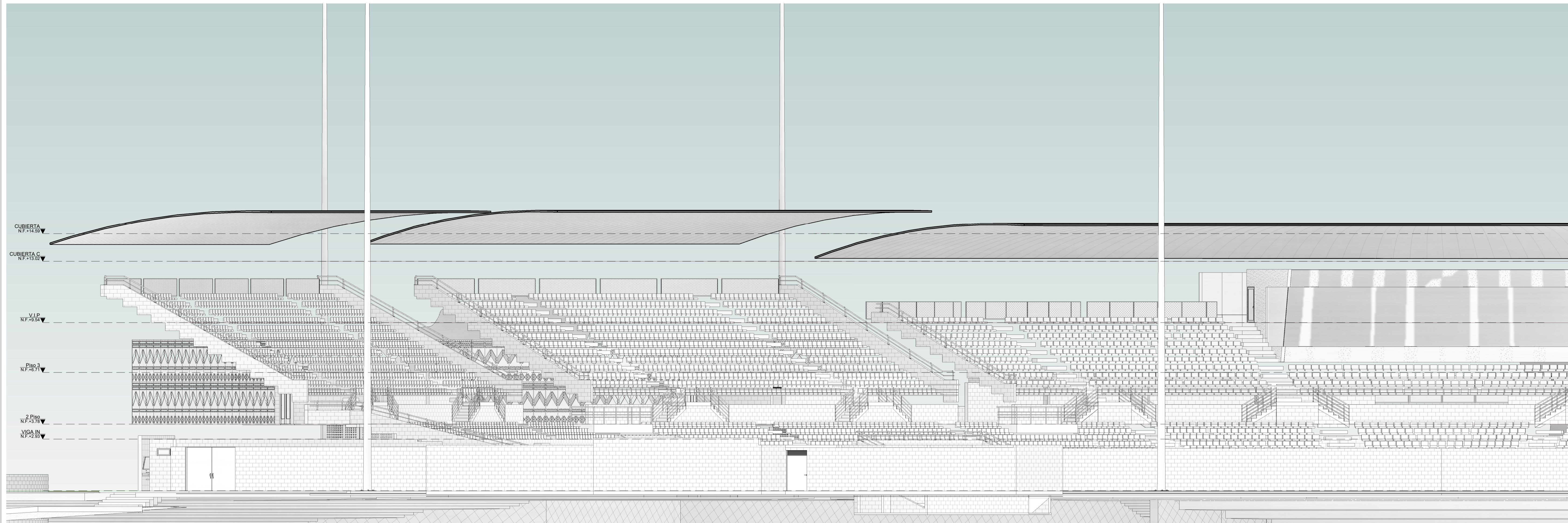
1 Este Seccion 1 1 : 100
