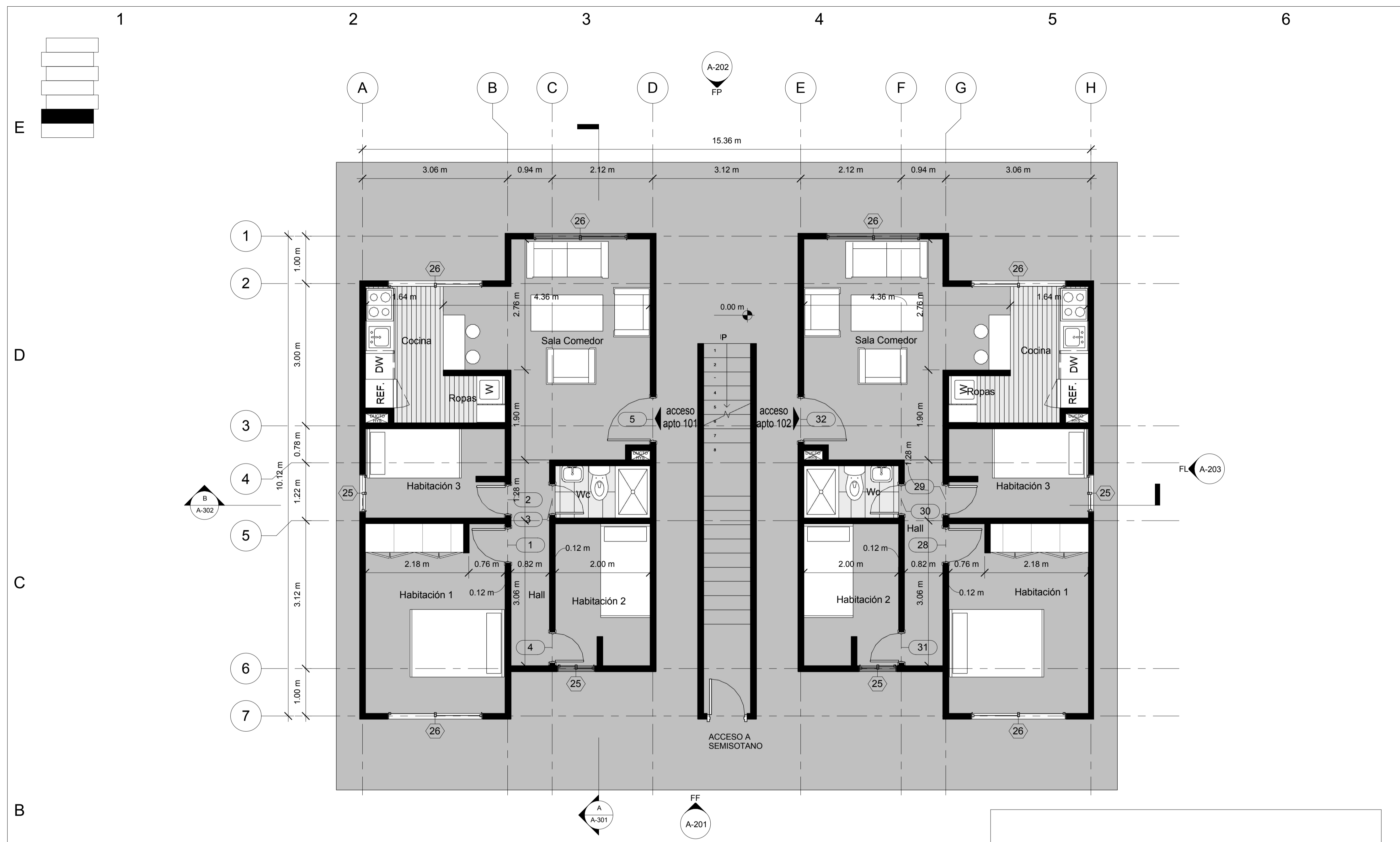
1 Planta 1 Bloque 54 1 : 50
