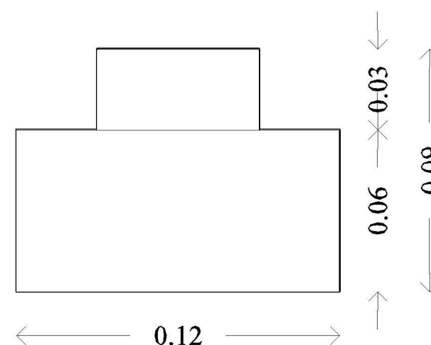
VISTA FRONTAL ESCALA 1:2
