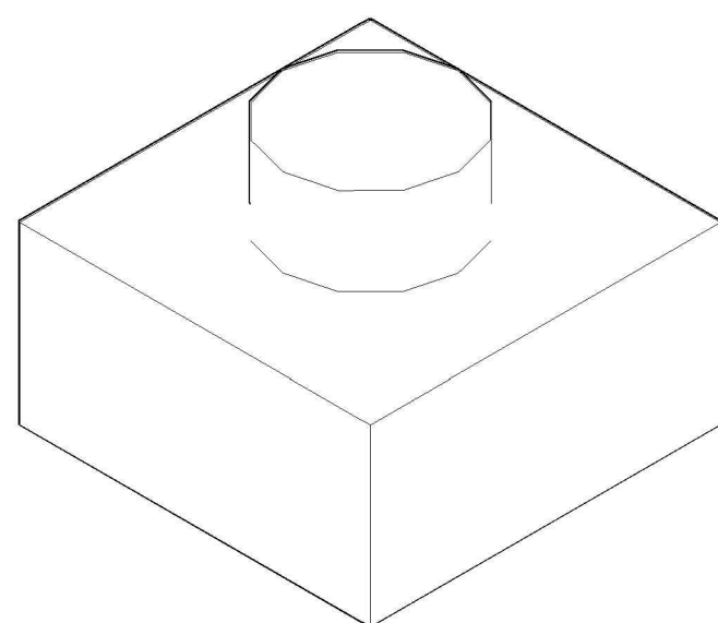
VISTA ISOMETRICA MEDIO LADRILLO ESCALA 1:2
